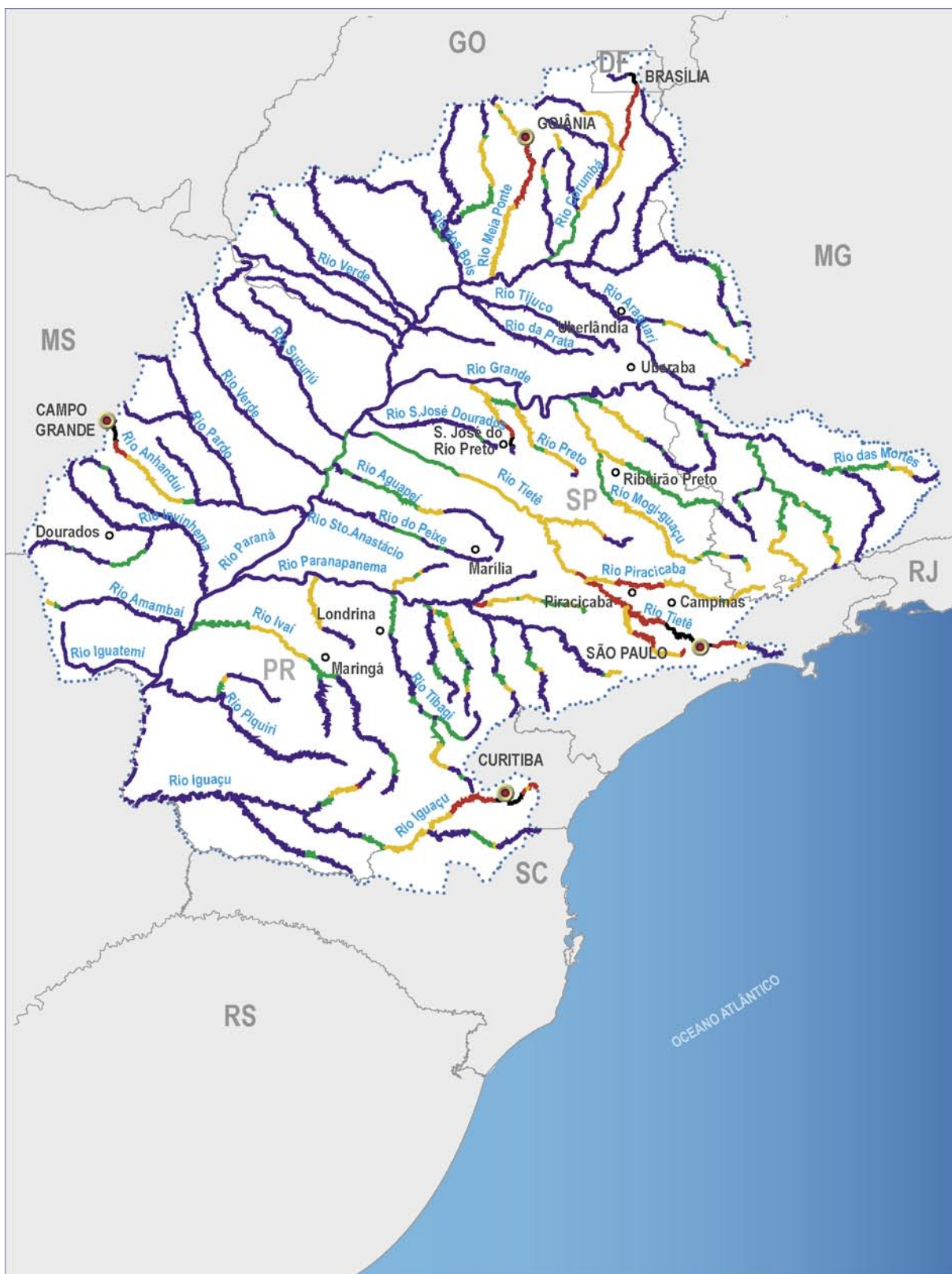
Figura 54 – Qualidade das águas em função do lançamento dos esgotos domésticos – Região Hidrográfica do Paraná
