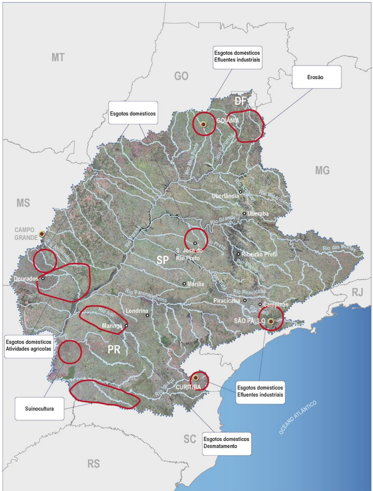
Figura 39 – Principais áreas críticas e suas respectivas fontes de poluição – Região Hidrográfica do Paraná
