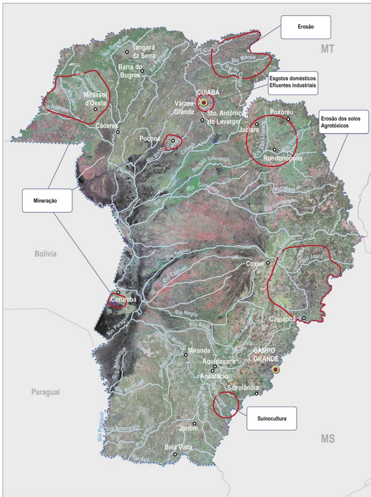
Figura 49 – Principais áreas críticas e suas respectivas fontes de poluição – Região Hidrográfica do Paraguai
