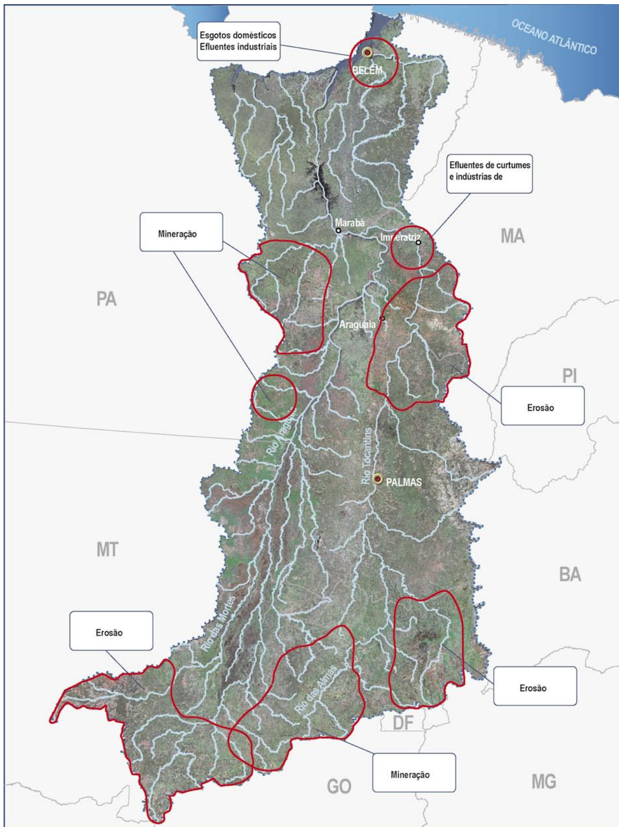
Figura 20 - Principais Áreas Críticas e suas Respectivas Fontes de Poluição - Região Hidrográfica do Tocantins
