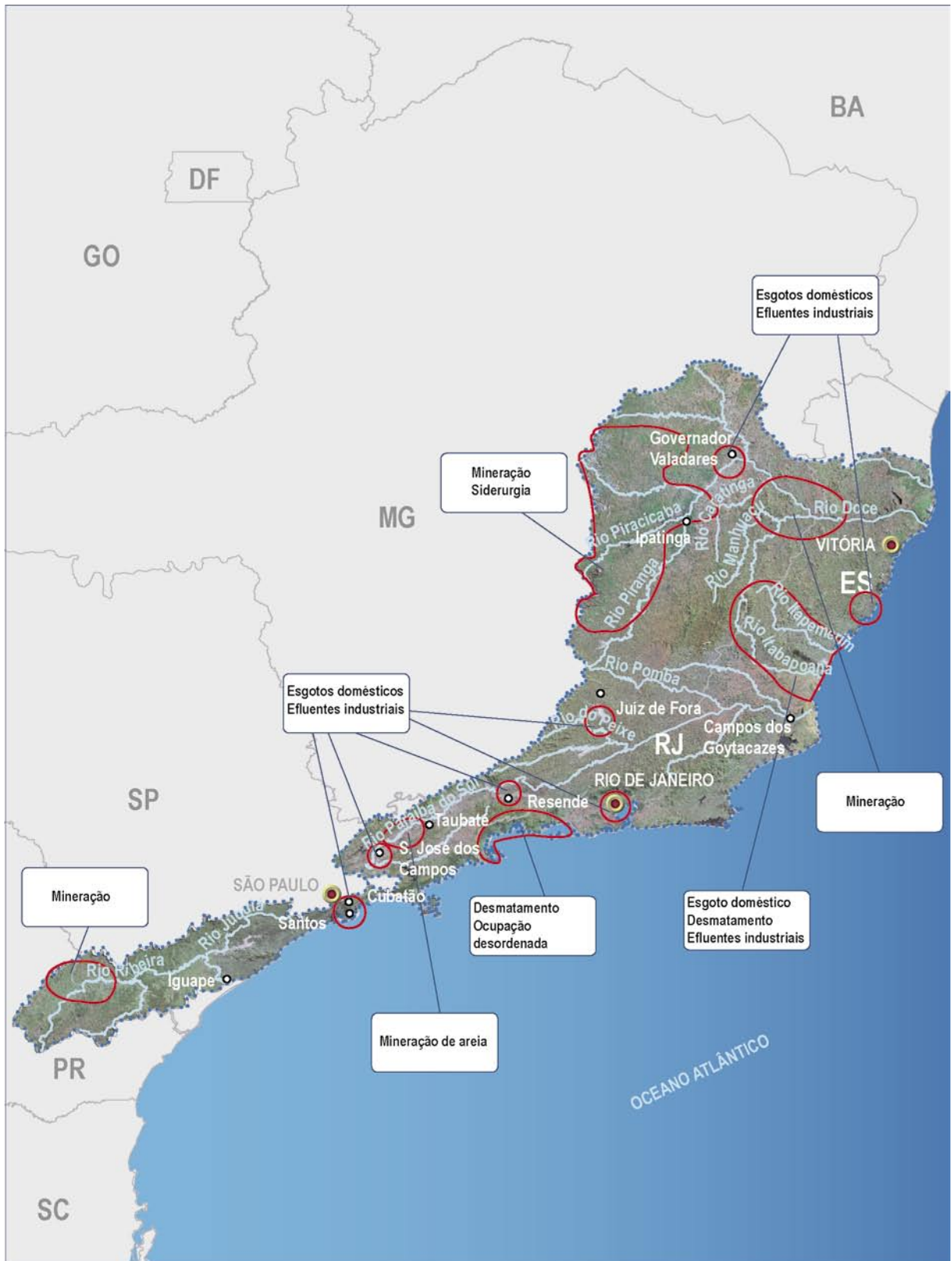
Figura 35 – Principais áreas críticas e suas respectivas fontes de poluição – Região Hidrográfica Atlântico Sudeste
