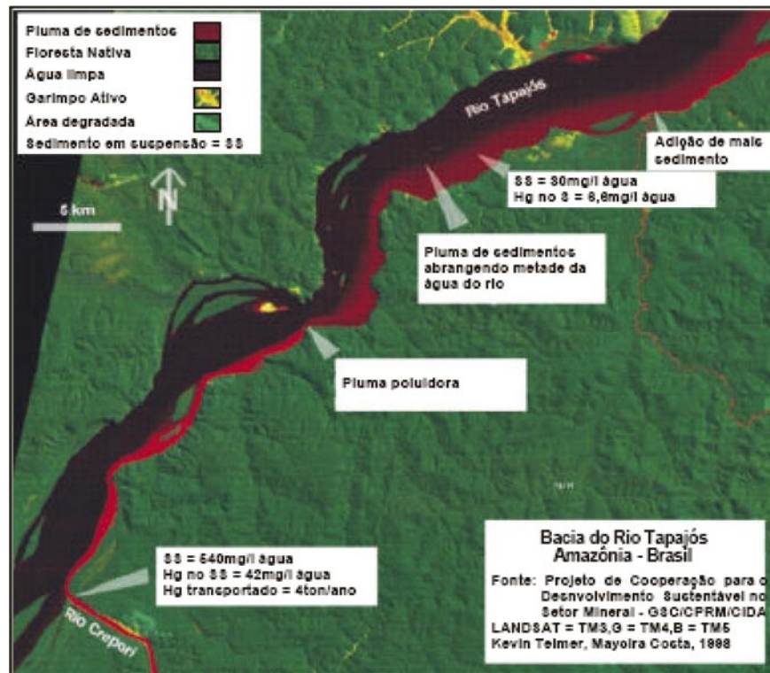
Figura 15 - Pluma de poluição causada pelo garimpo de ouro no rio Tapajós.
