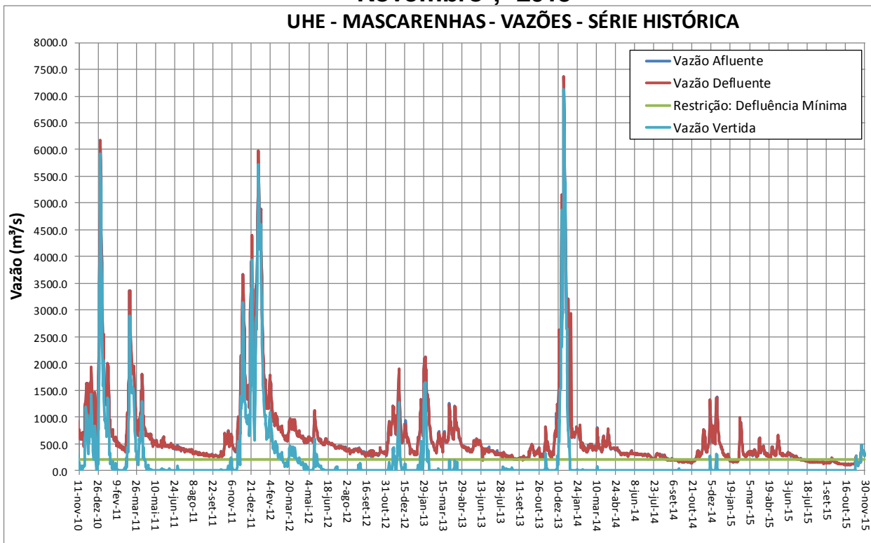
UHE - MASCARENHAS - VAZÕES - MENSAL
