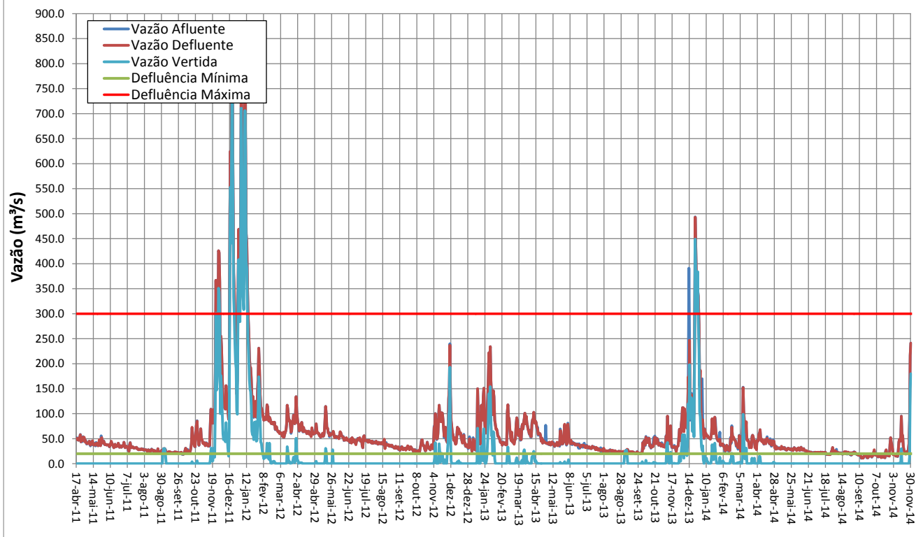
UHE - SÁ CARVALHO - VAZÕES - SÉRIE HISTÓRICA
