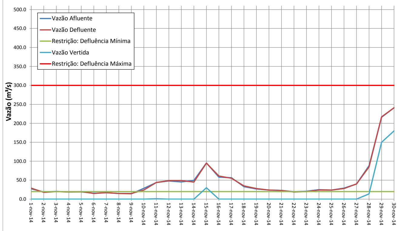
UHE - SÁ CARVALHO - VAZÕES - MENSAL
