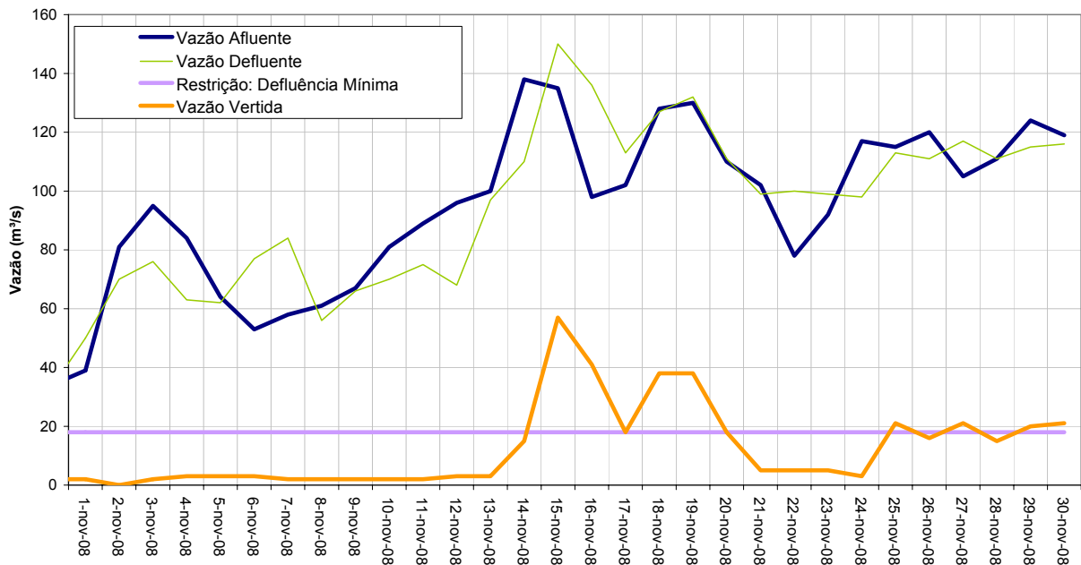
AHE - SALTO GRANDE - VAZÕES - novembro 2008
