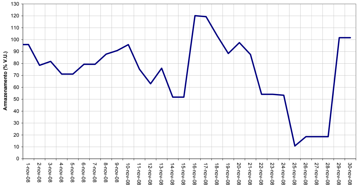
AHE - MASCARENHAS - VOLUME ARMAZENADO - novembro 2008
