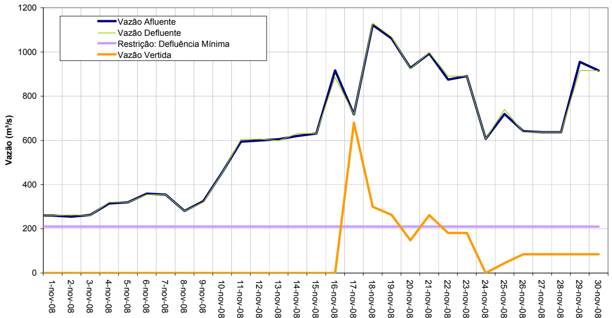
AHE - MASCARENHAS - VAZÕES - novembro 2008
