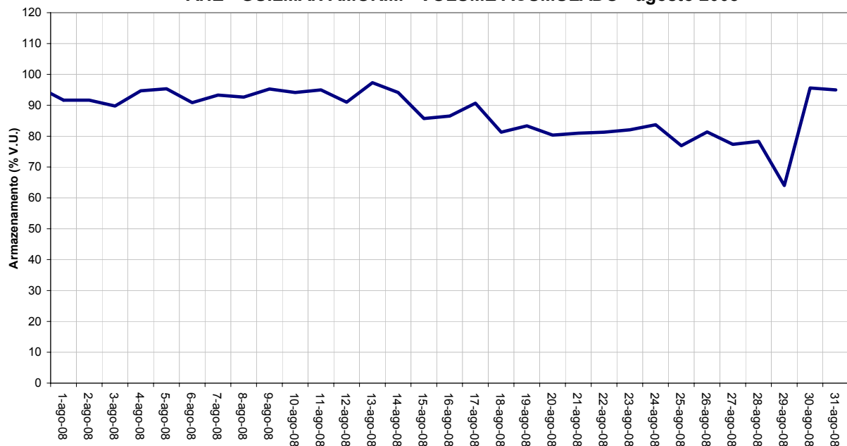
AHE - GUILMAN AMORIM - VOLUME ACUMULADO - agosto 2008
