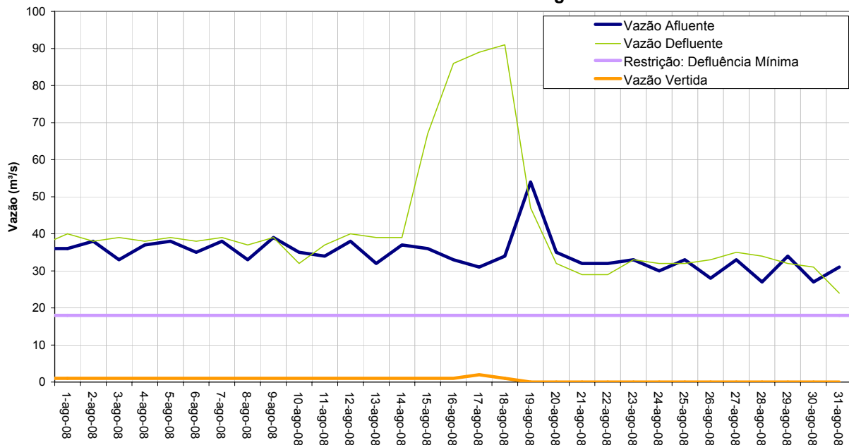
AHE - SALTO GRANDE - VAZÕES - agosto 2008
