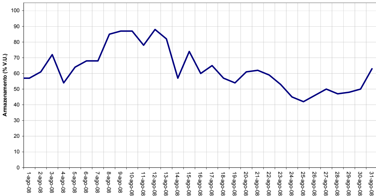
AHE - CANDONGA - VOLUME ARMAZENADO - agosto 2008
