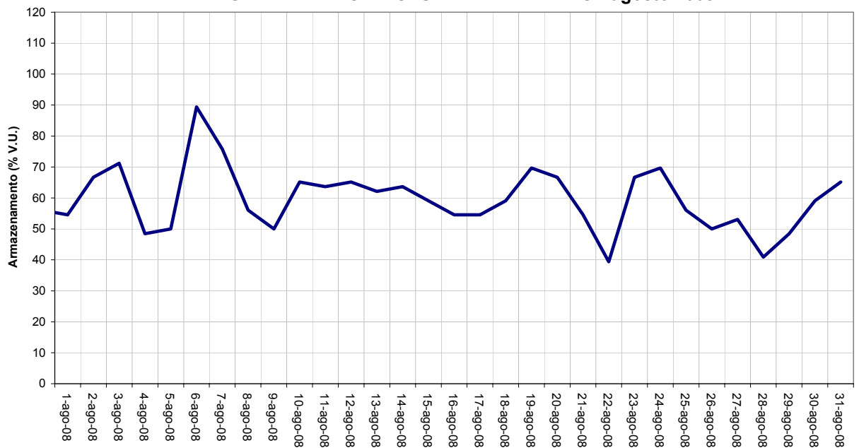
AHE - SÁ CARVALHO - VOLUME ARMAZENADO - agosto 2008
