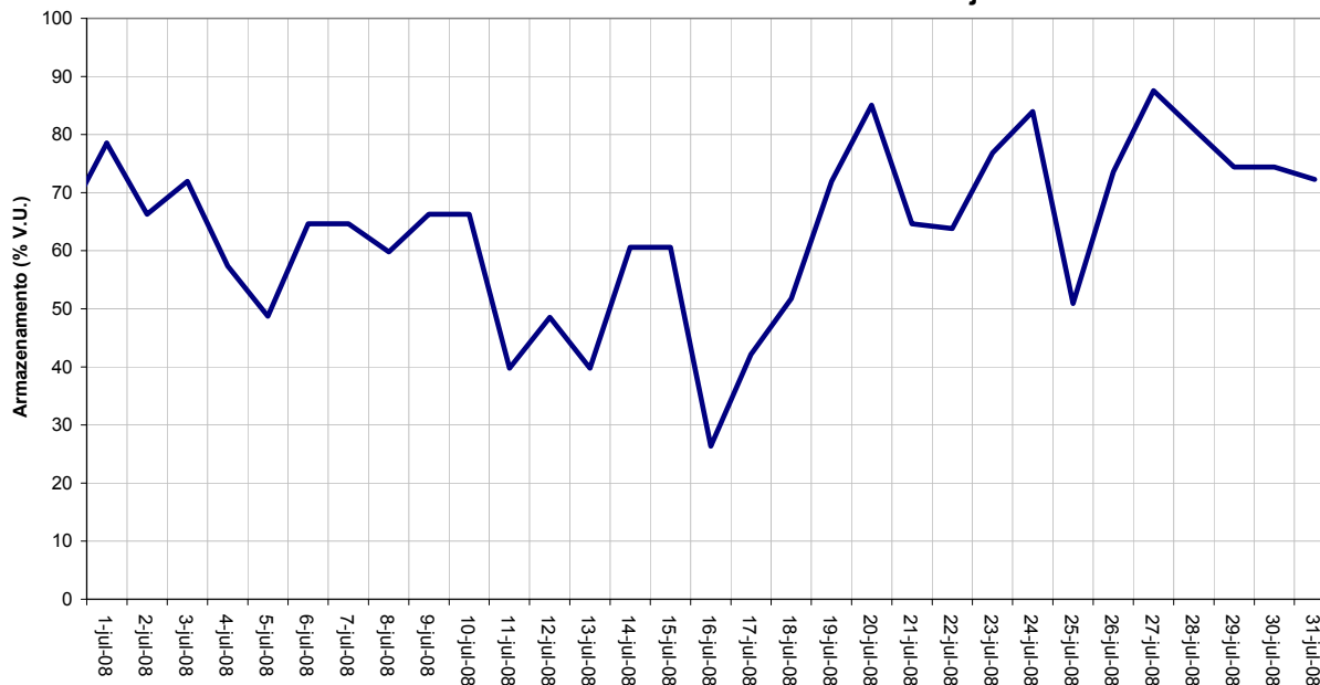
AHE - MASCARENHAS - VOLUME ARMAZENADO - julho 2008
