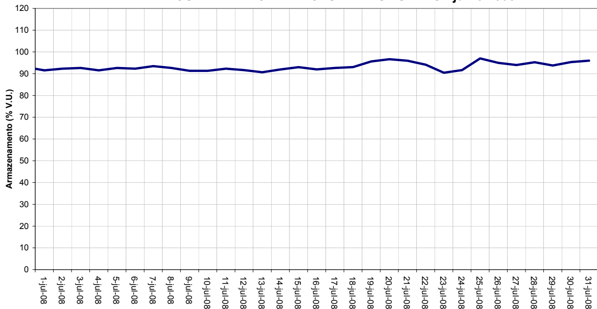
AHE - GUILMAN AMORIM - VOLUME ACUMULADO - julho 2008
