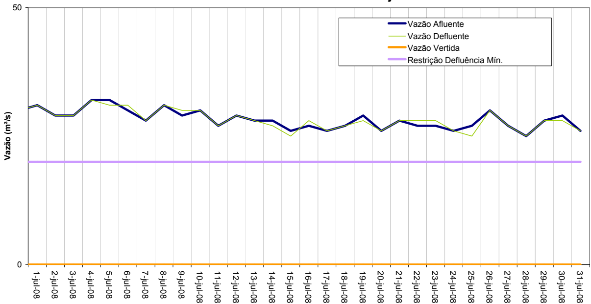
AHE - GUILMAN AMORIM - VAZÕES - julho 2008
