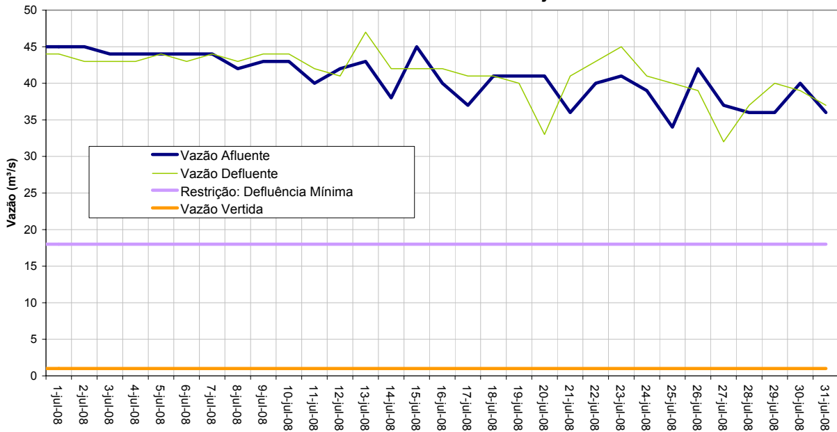
AHE - SALTO GRANDE - VAZÕES - julho 2008
