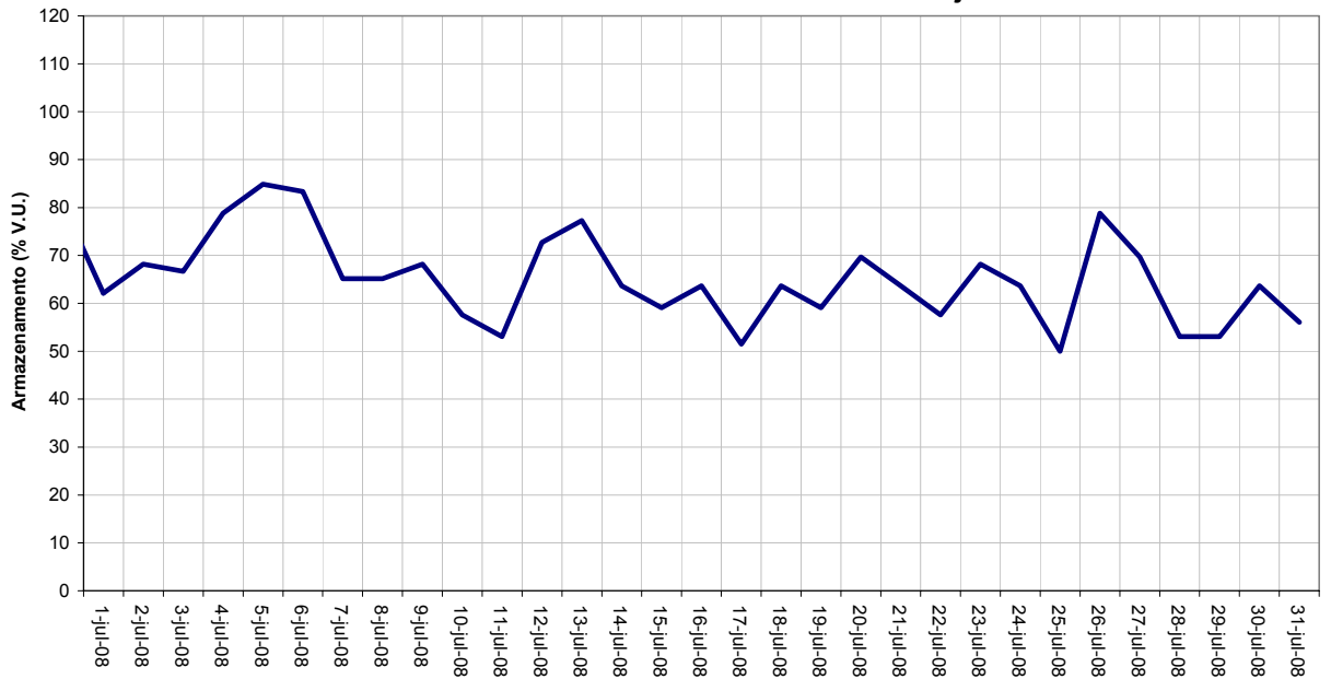
AHE - SÁ CARVALHO - VOLUME ARMazenADO - julho 2008
