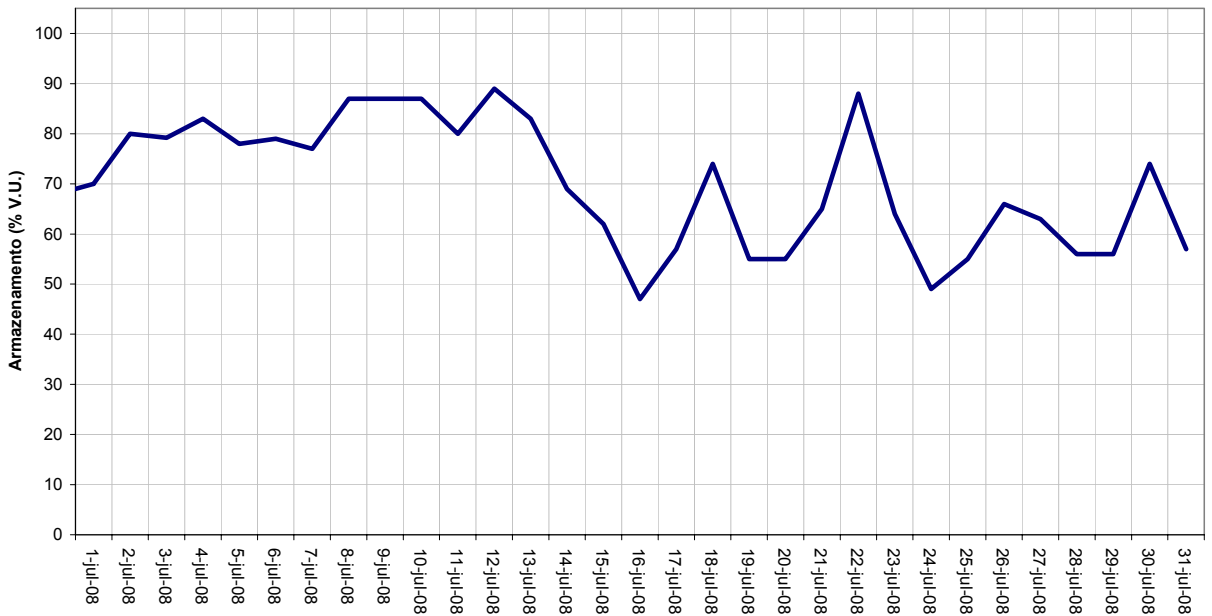
AHE - CANDONGA - VOLUME ARMAZENADO - julho 2008
