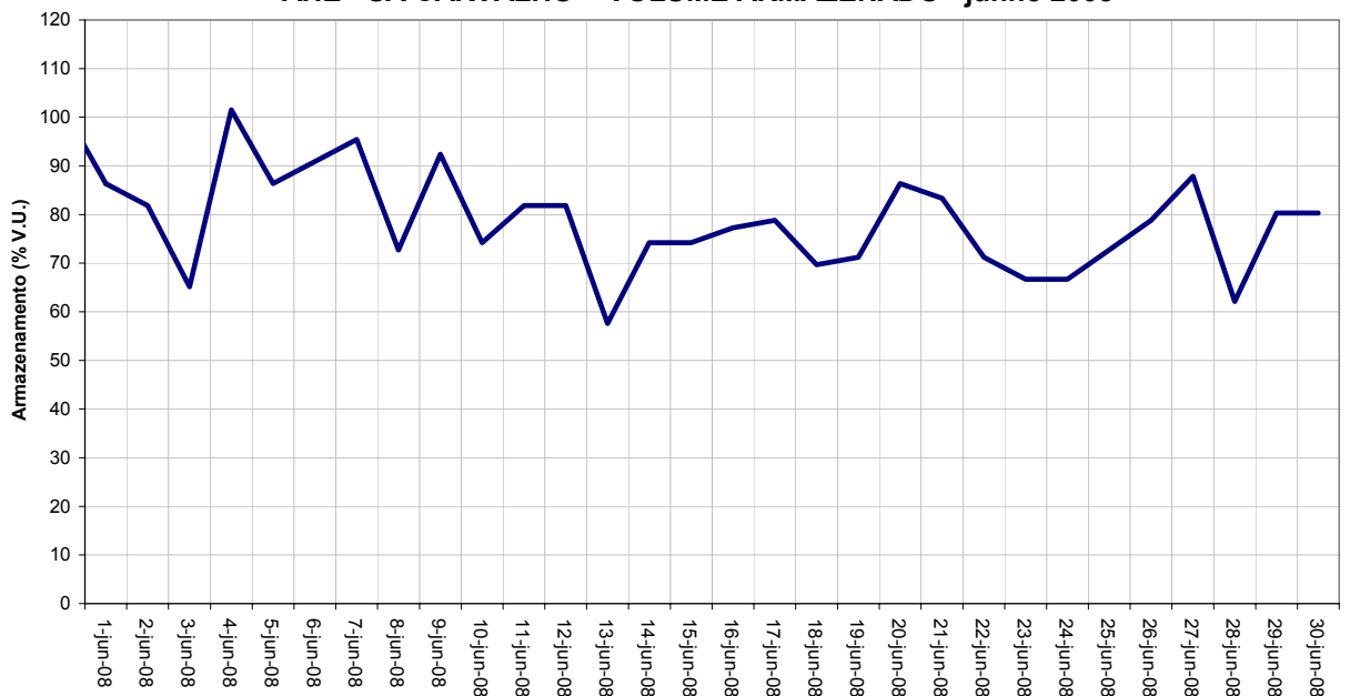
AHE - SÁ CARVALHO - VOLUME ARMAZENADO - junho 2008
