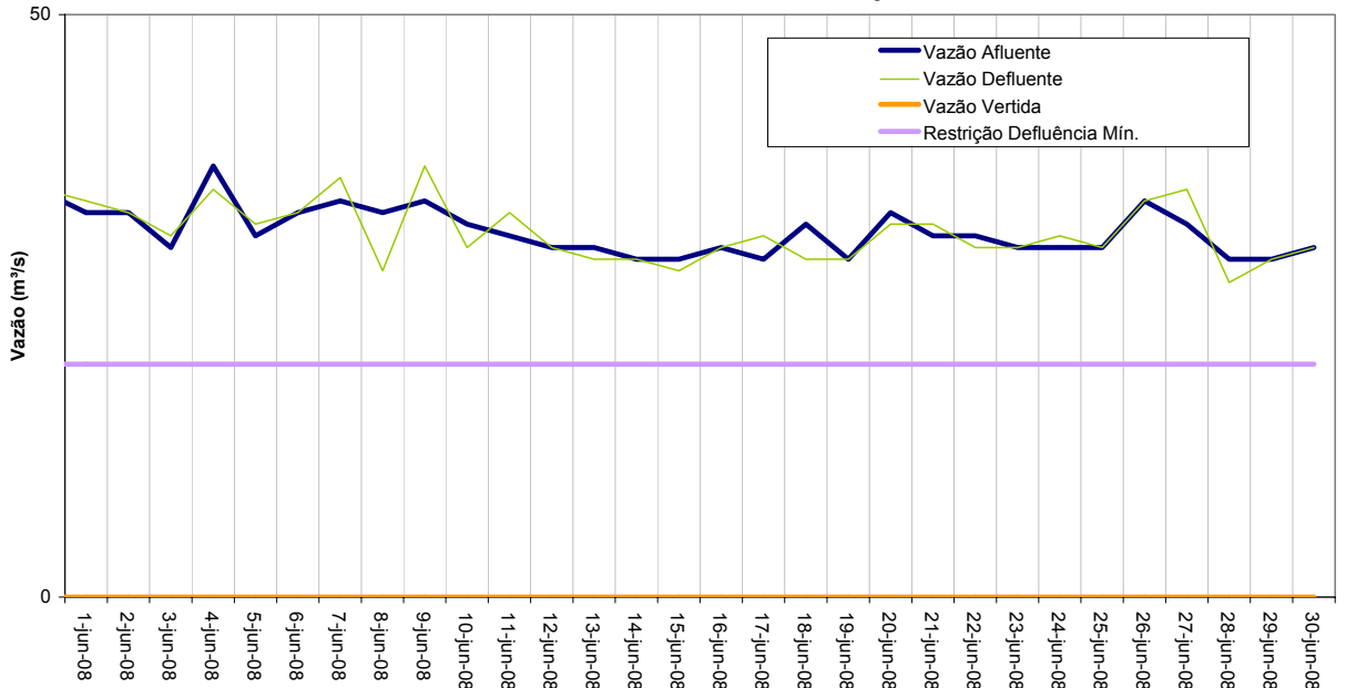
AHE - GUILMAN AMORIM - VAZÕES - junho 2008
