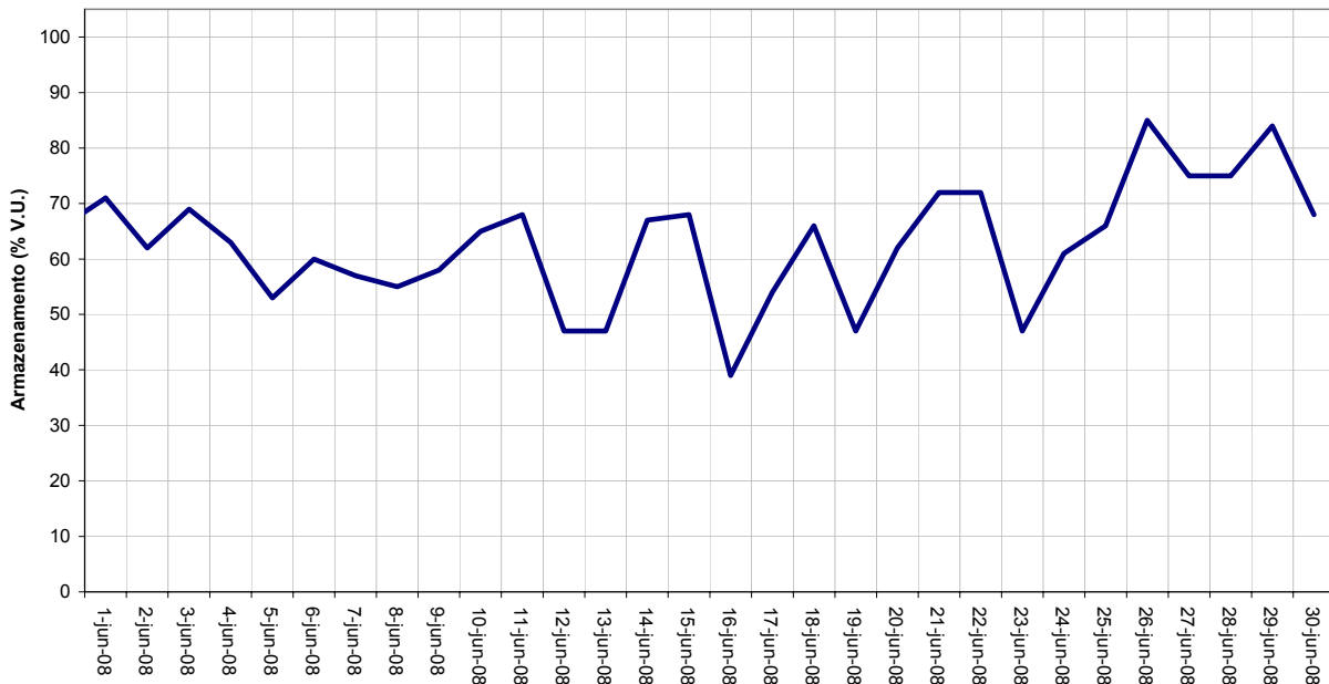
AHE - CANDONGA - VOLUME ARMAZENADO - junho 2008
