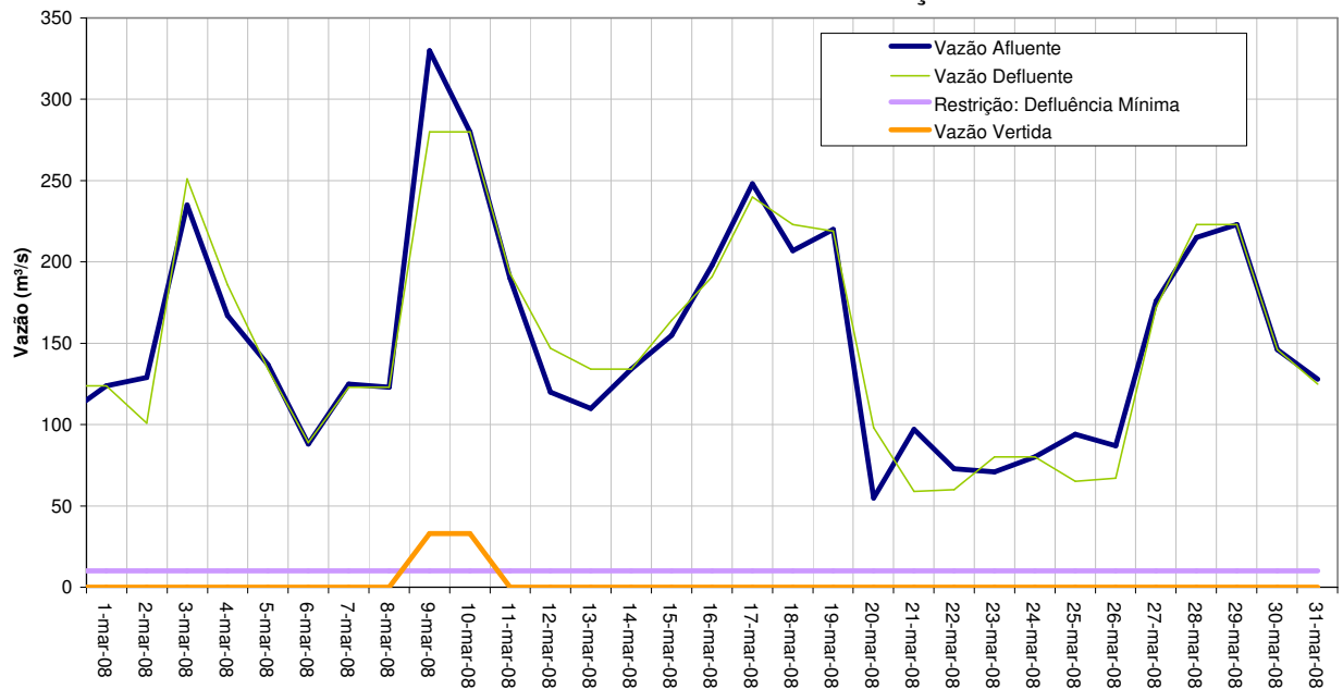
AHE - PORTO ESTRELA - VAZÕES - março 2008
