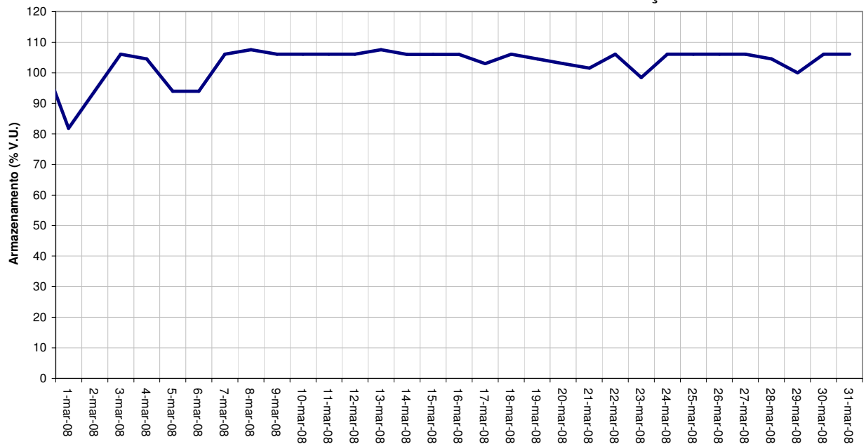
AHE - SÁ CARVALHO - VOLUME ARMAZENADO - março 2008
