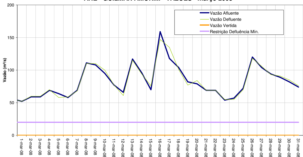
AHE - GUILMAN AMORIM - VAZÕES - março 2008
