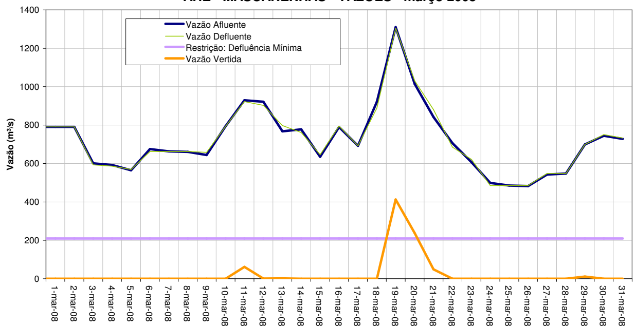
AHE - MASCARENHAS - VAZÕES - março 2008
