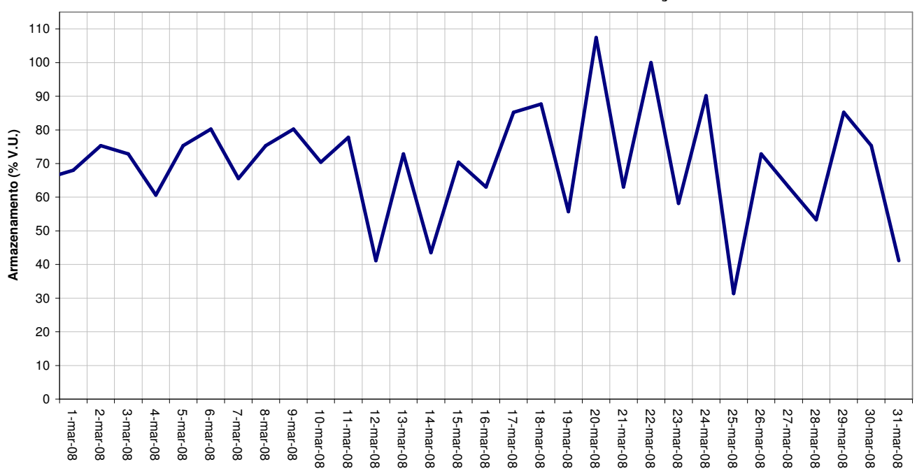
AHE - AIMORÉS - VOLUME ARMAZENADO - março 2008
