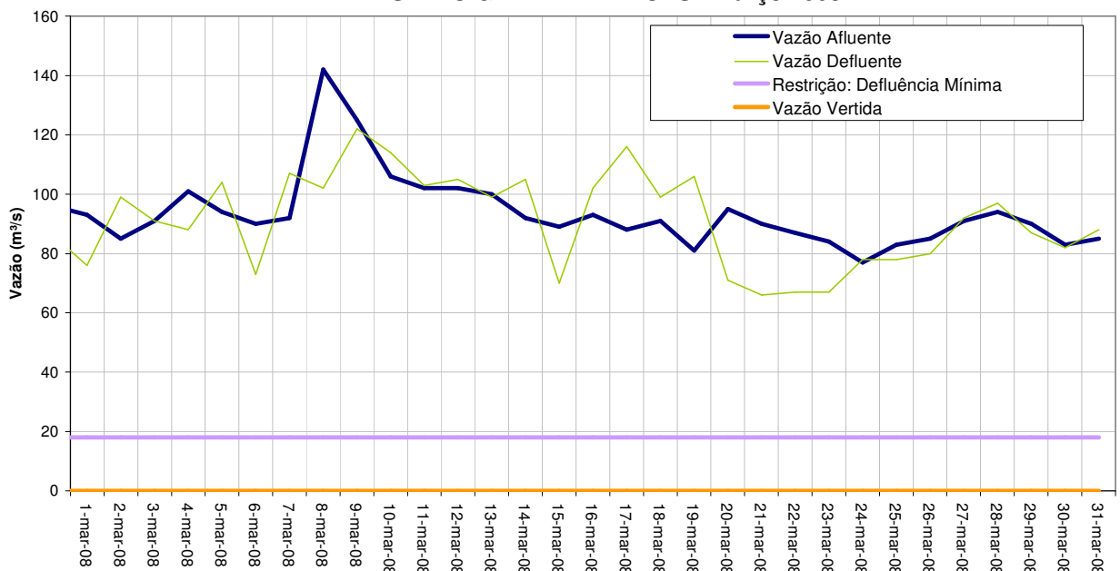
AHE - SALTO GRANDE - VAZÕES - março 2008
