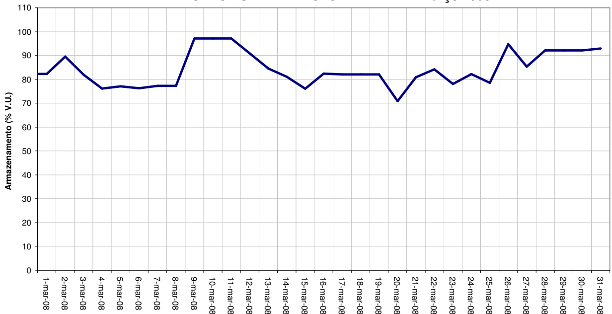
AHE - PORTO ESTRELA - VOLUME ARMAZ. - março 2008
