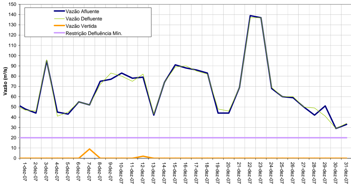
AHE - GUILMAN AMORIM - VAZÕES - dezembro 2007
