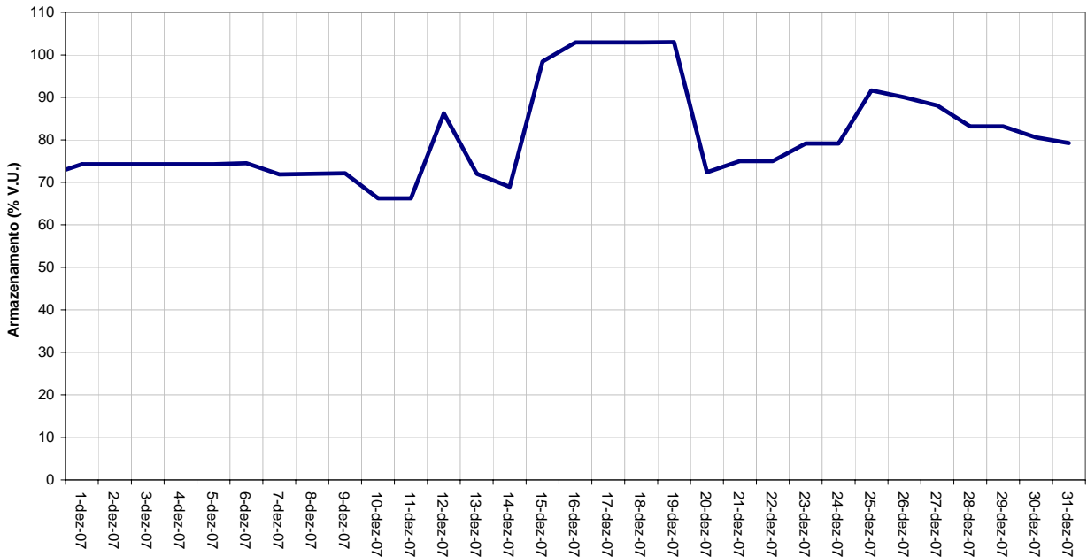
AHE - PORTO ESTRELA - VOLUME ARMAZ. - dezembro 2007
