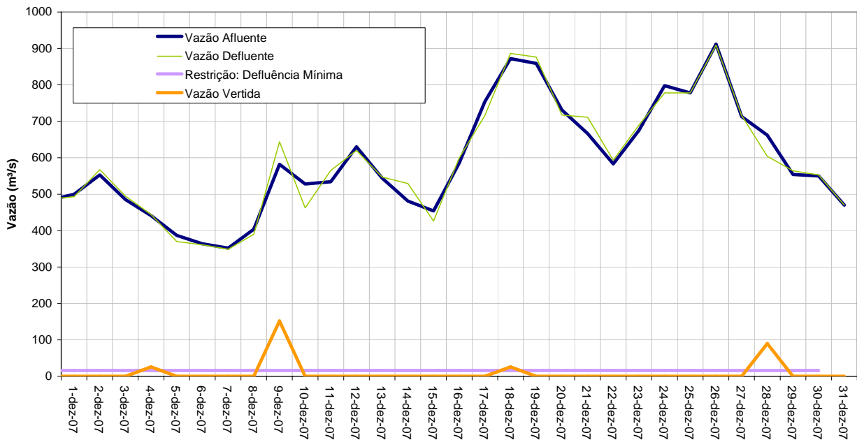
AHE - AIMORÉS - VAZÕES - dezembro 2007
