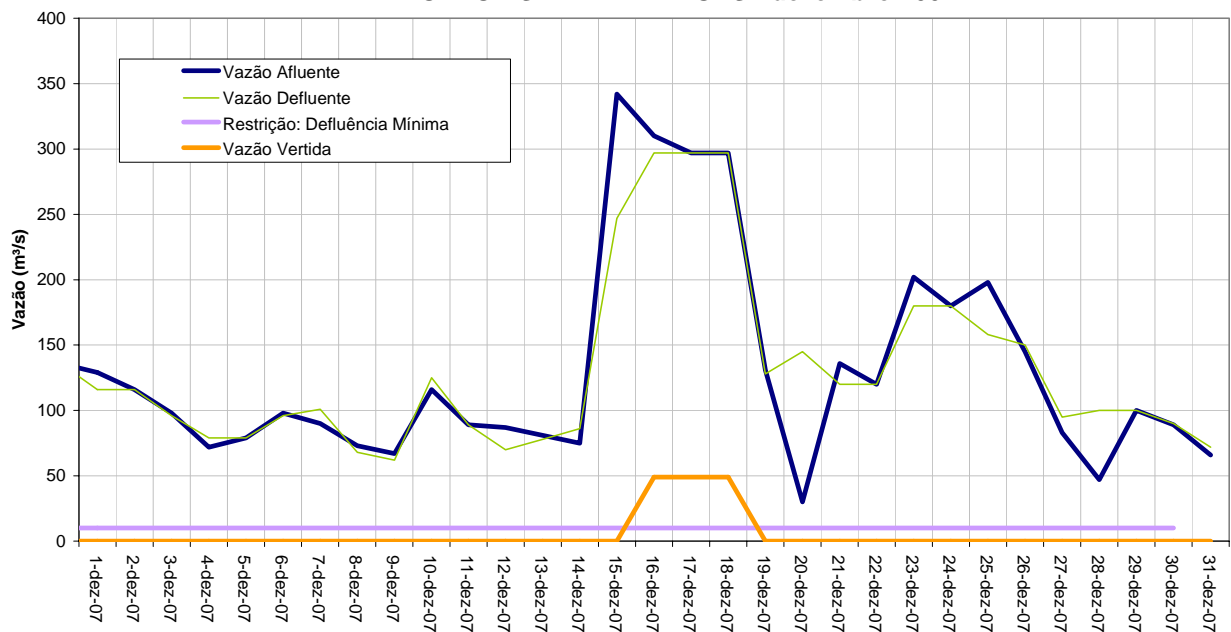
AHE - PORTO ESTRELA - VAZÕES - dezembro 2007
