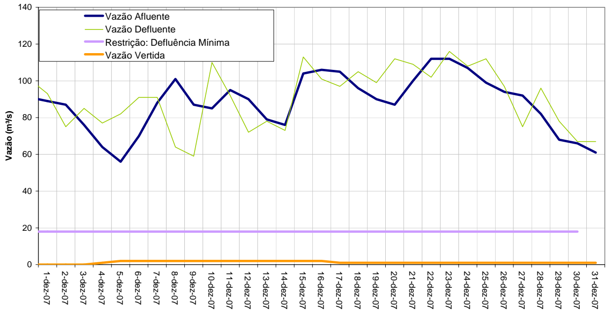
AHE - SALTO GRANDE - VAZÕES - dezembro 2007
