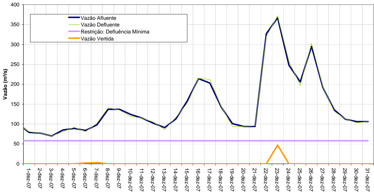
AHE - CANDONGA - VAZÕES - dezembro 2007
