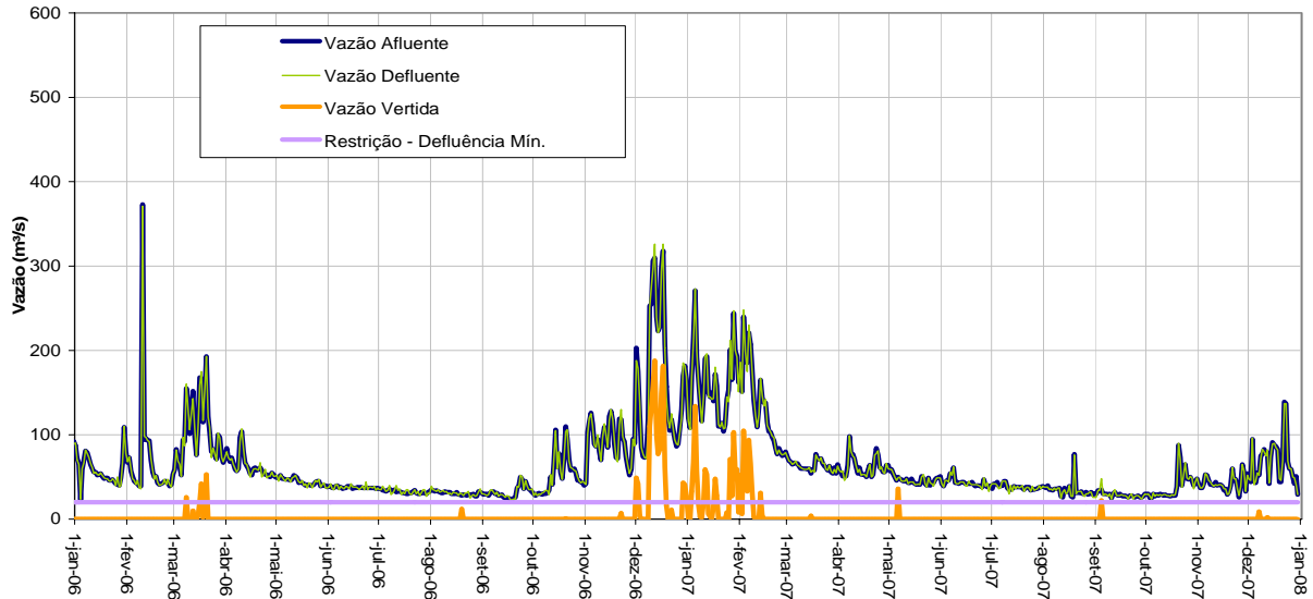
AHE - GUILMAN AMORIM - VAZÕES
