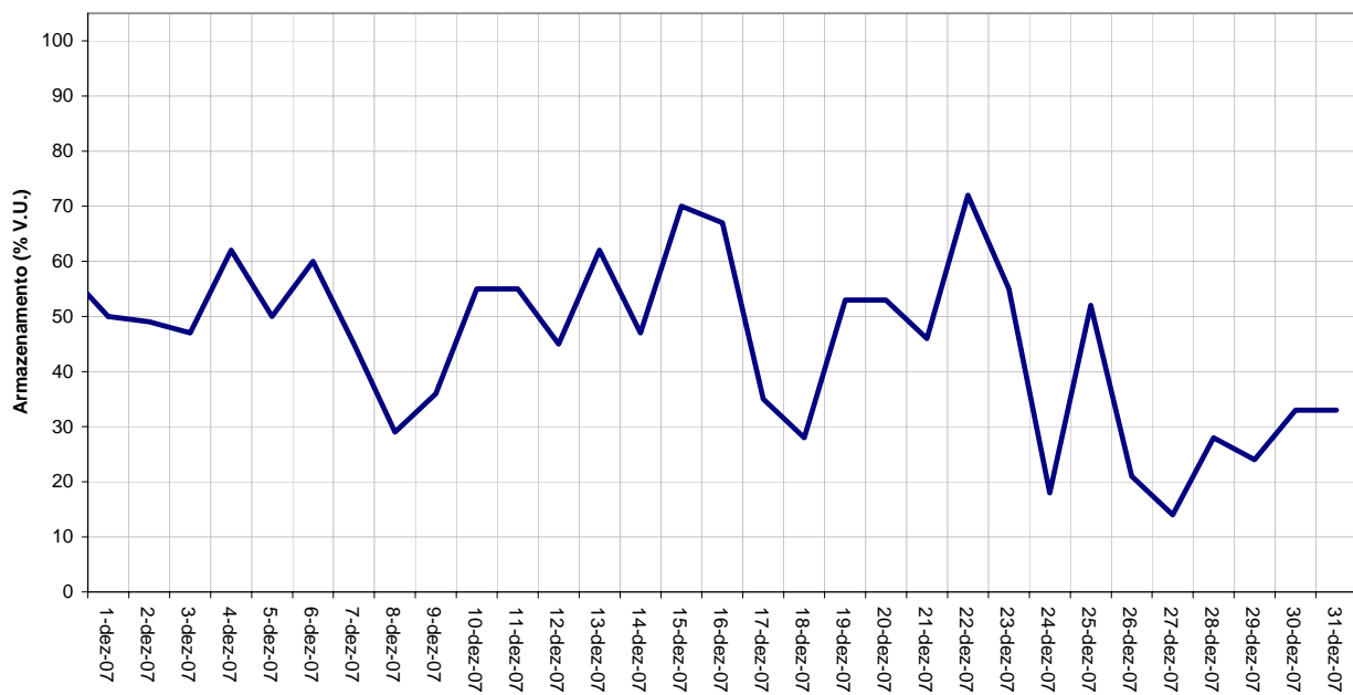
AHE - CANDONGA - VOLUME ARMAZENADO - dezembro 2007
