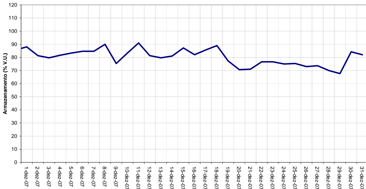
AHE - GUILMAN AMORIM - VOLUME ACUMULADO - dezembro 2007
