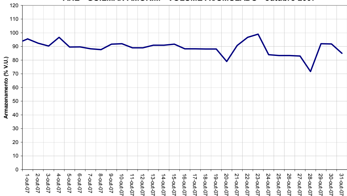
AHE - GUILMAN AMORIM - VOLUME ACUMULADO - outubro 2007
