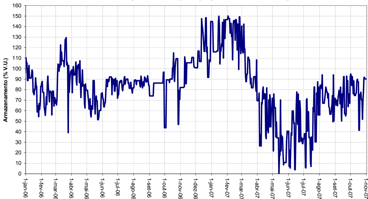
AHE - MASCARENHAS - VOLUME ARMAZENADO
