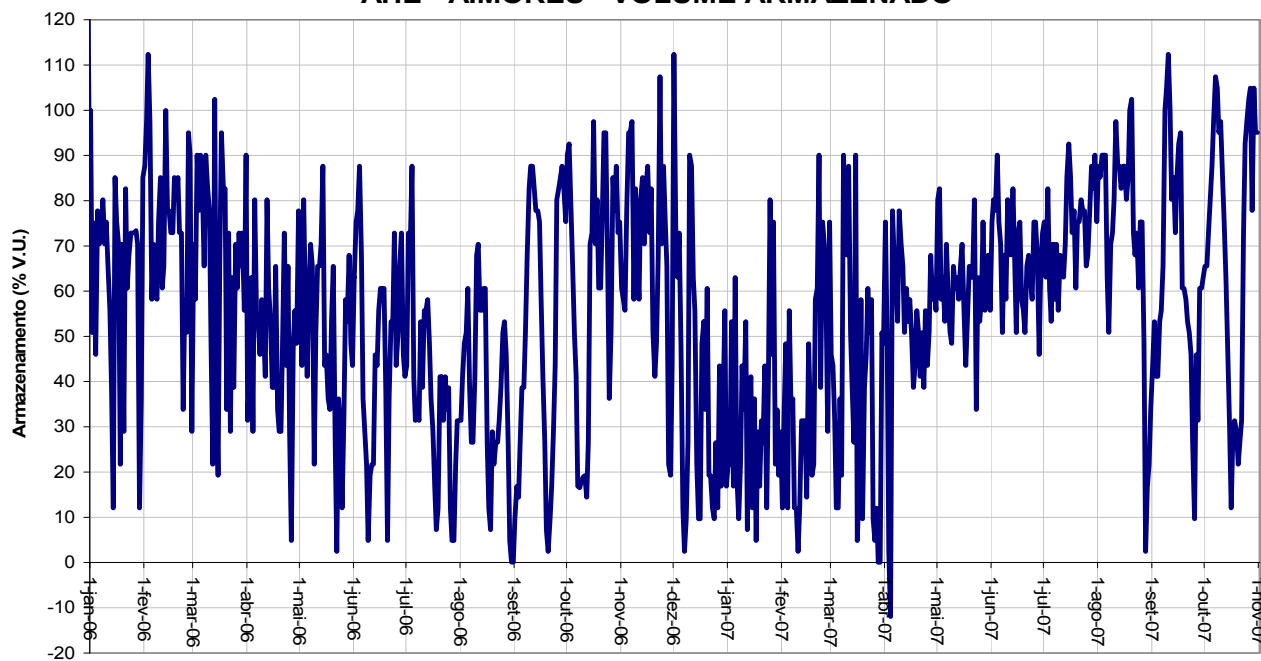
AHE - AIMORÉS - VOLUME ARMazenADO
