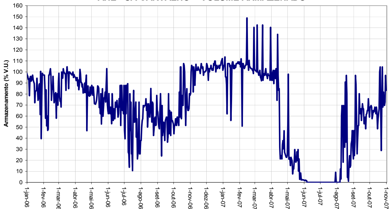
AHE - SÁ CARVALHO - VOLUME ARMAZENADO
