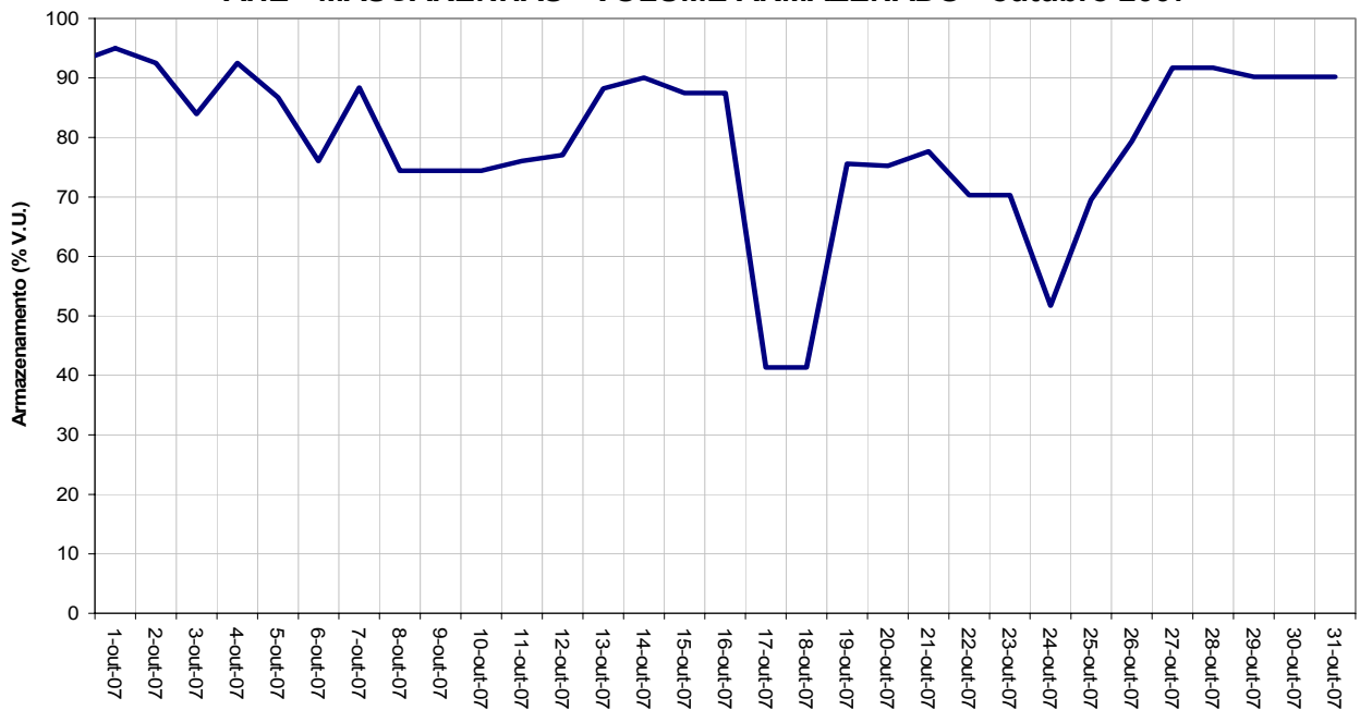
AHE - MASCARENHAS - VOLUME ARMAZENADO - outubro 2007
