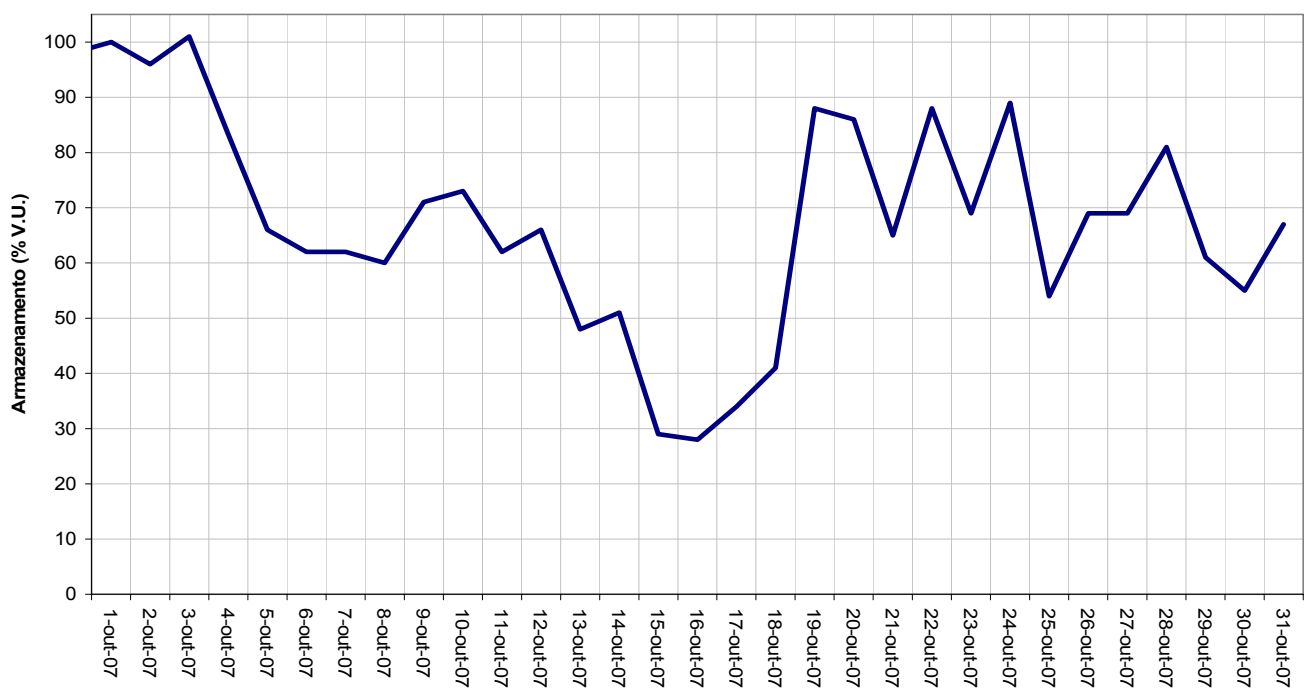
AHE - CANDONGA - VOLUME ARMAZENADO - outubro 2007
