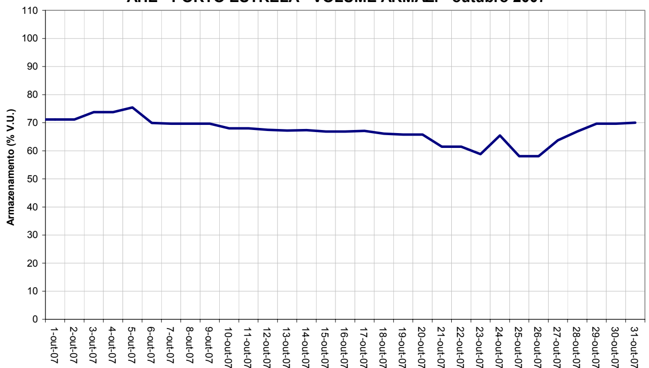
AHE - PORTO ESTRELA - VOLUME ARMAZ. - outubro 2007
