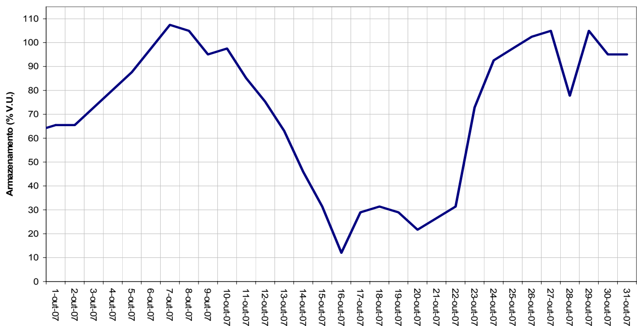
AHE - AIMORÉS - VOLUME ARMazenADO - outubro 2007
