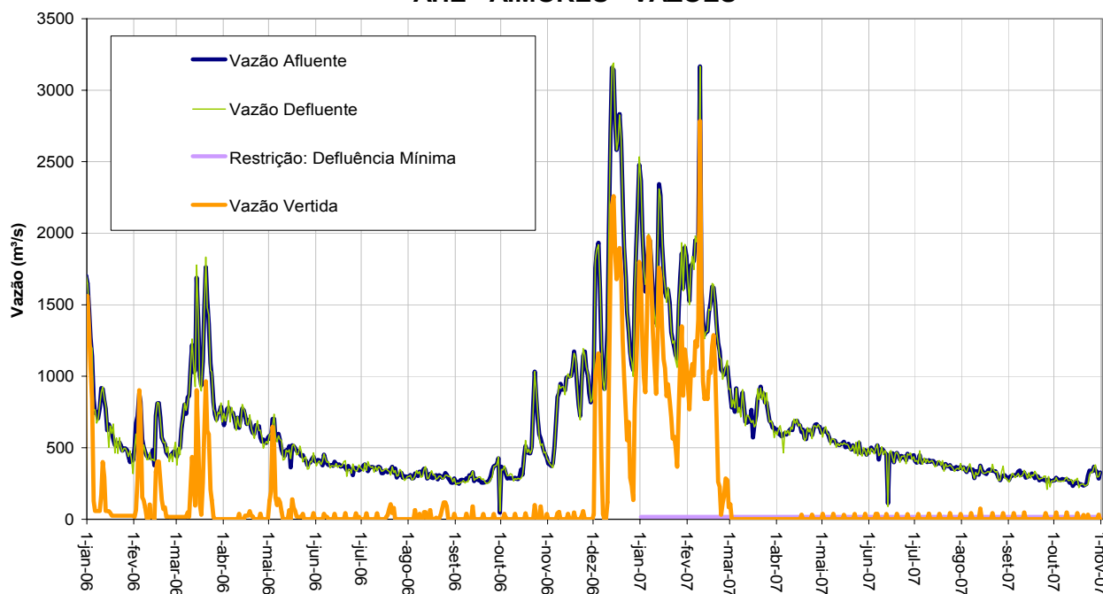
AHE - AIMORÉS - VAZÕES - outubro 2007
