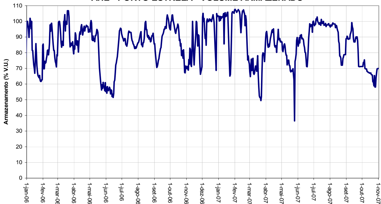
AHE - PORTO ESTRELA - VOLUME ARMAZENADO
