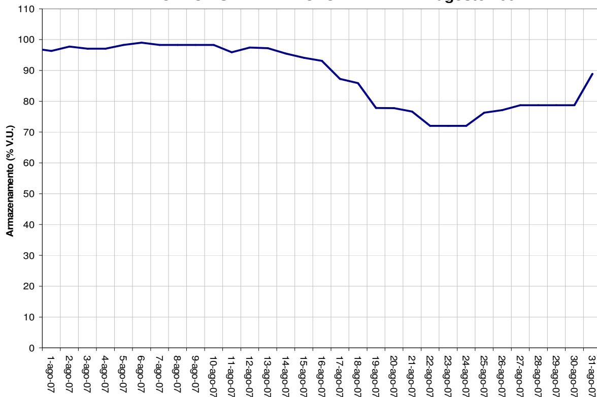
AHE - PORTO ESTRELA - VOLUME ARMAZ. - agosto 2007
