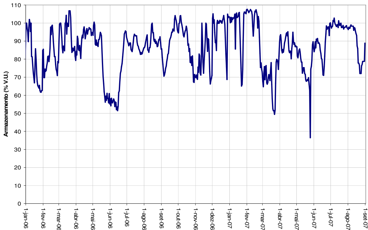
AHE - PORTO ESTRELA - VOLUME ARMAZ. - agosto 2007
