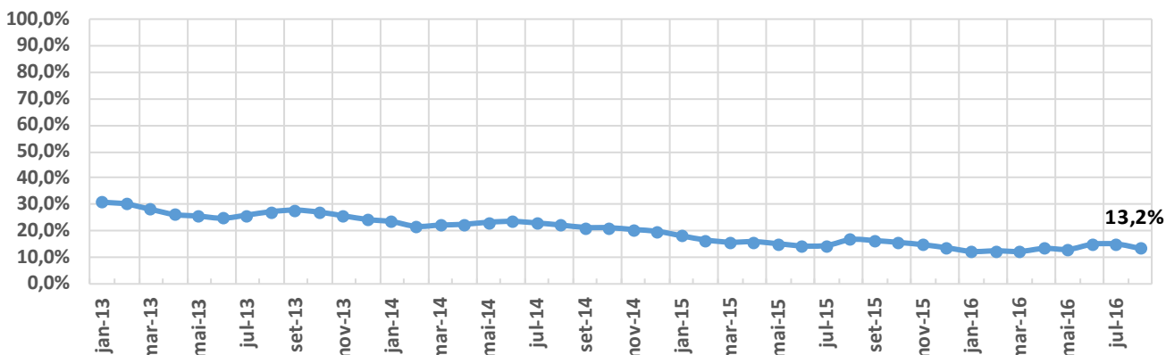
Volume do reservatório equivalente de Pernambuco
