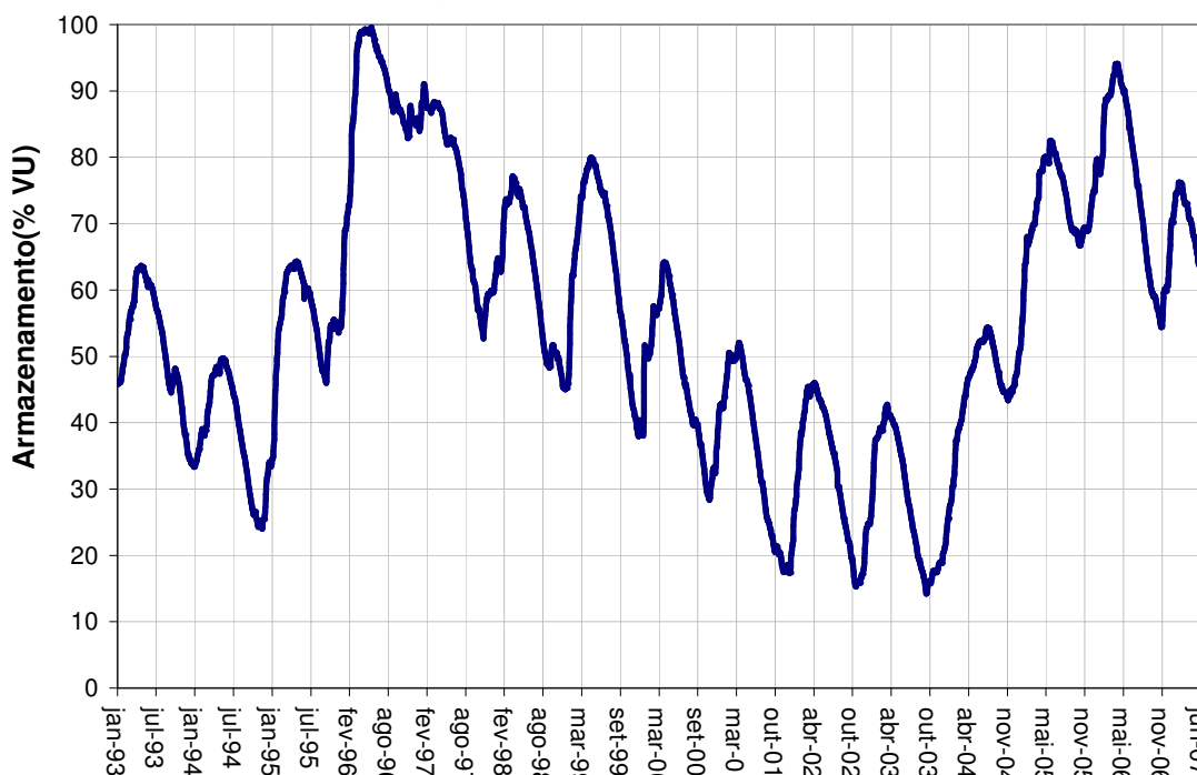
RESERVATÓRIO EQUIVALENTE - VOLUME ACUMULADO DESDE 1993
