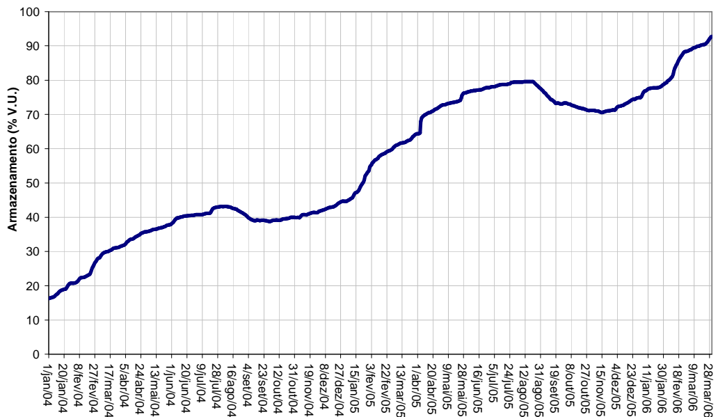
PARAIBUNA - VOLUME ACUMULADO (% V.U.)
