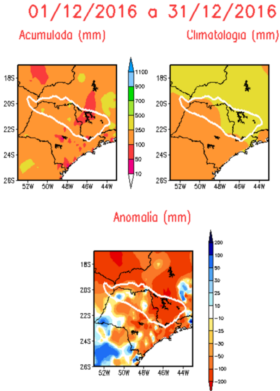
Figura 10 – Precipitação mensal acumulada, média climatológica e anomalia de precipitação na Bacia do rio Grande, no período de 01/12/16 a 31/12/16.
