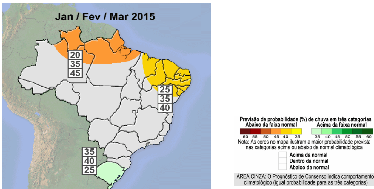
Figura 12 – Previsão climática para o trimestre jan/ fev/ mar de 2015.
