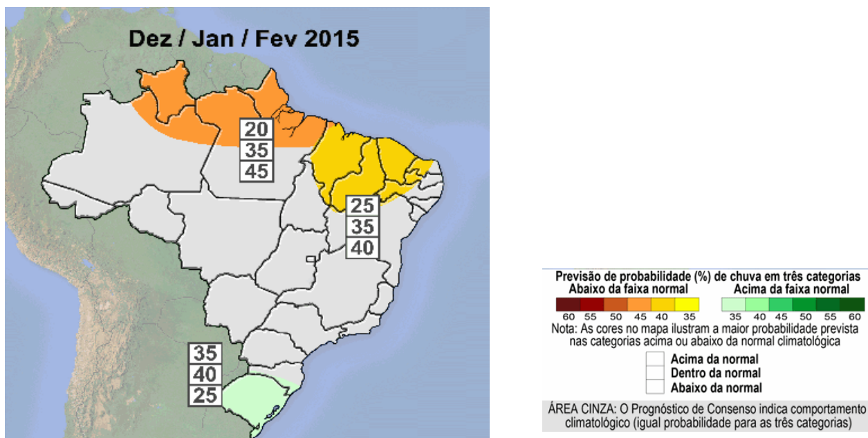
Figura 12 – Previsão climática para o trimestre dez/ jan/ fev de 2015.
