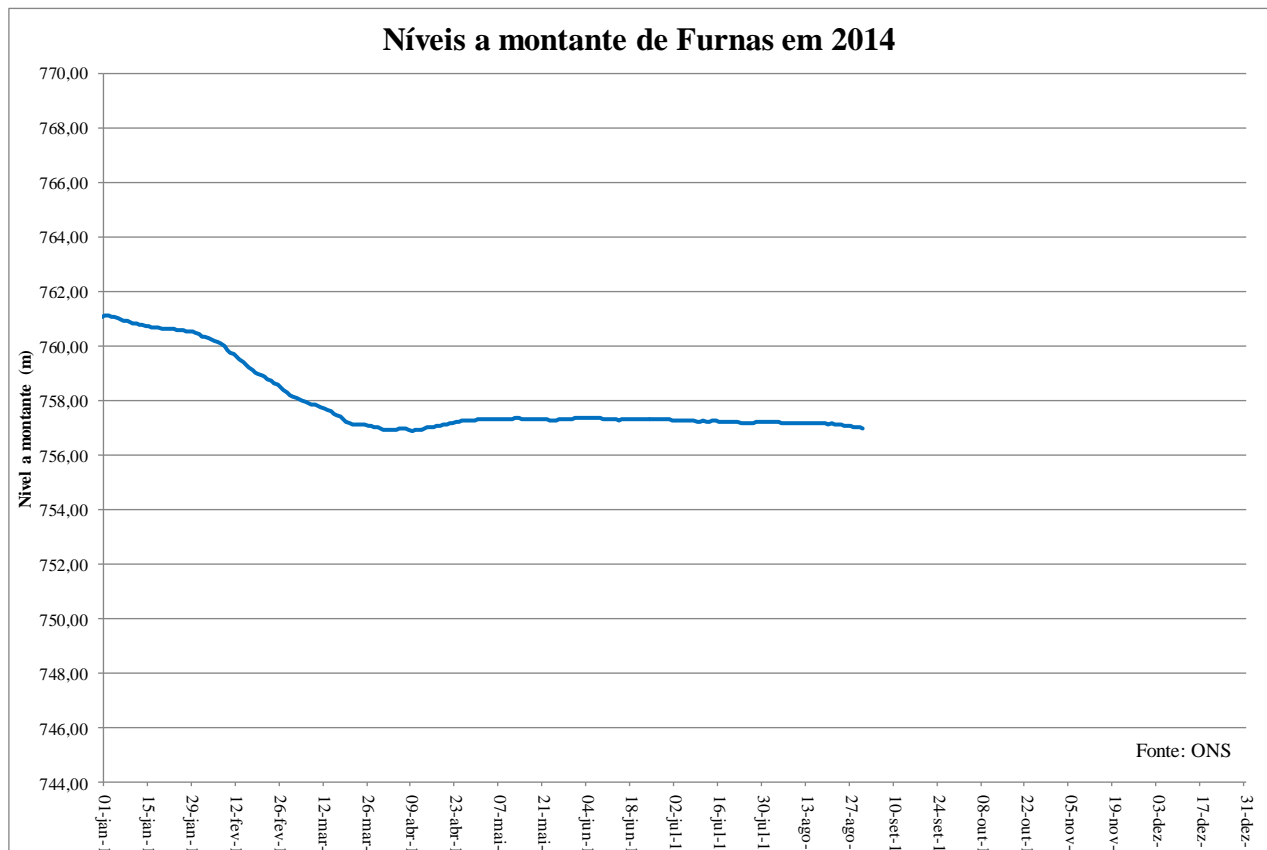
Figura 7 – Níveis a montante do reservatório de Furnas em 2014
