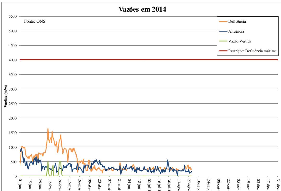
Figura 3 – Vazões no reservatório de Furnas em 2014
