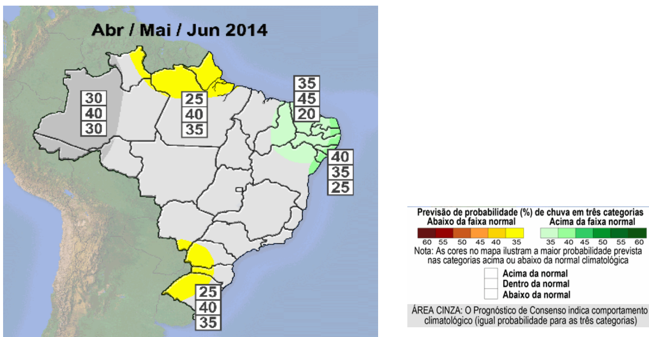
Figura 12 – Previsão climática para o trimestre abr/ mai / jun de 2014.
