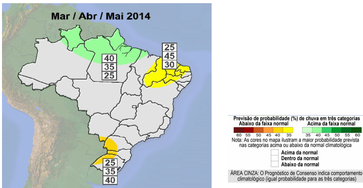
Figura 12 – Previsão climática para o trimestre mar / abr / mai de 2014.
