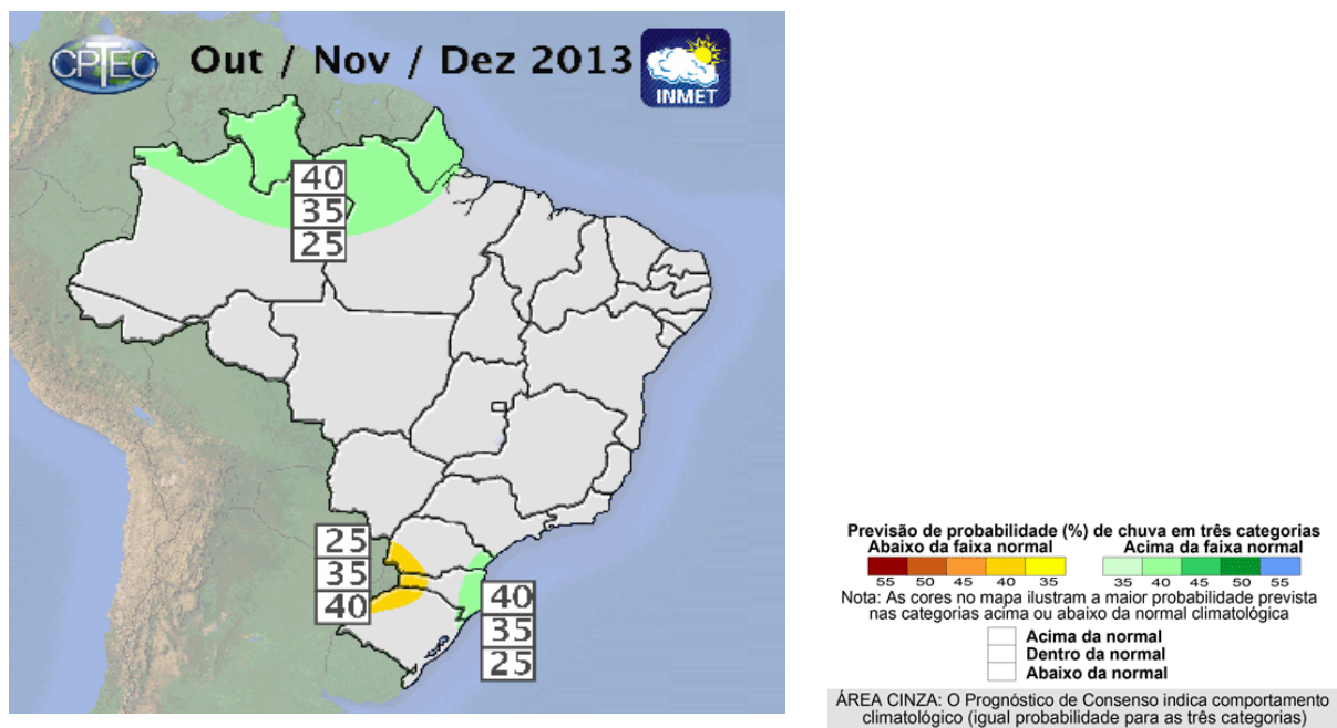
Figura 12 – Previsão climática para o trimestre out / nov/ dez de 2013.
