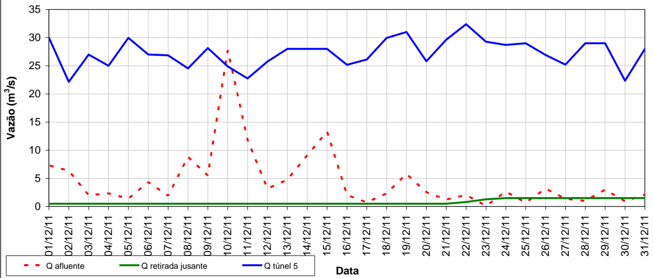
Vazões características do reservatório Atibainha - Dez/2011
