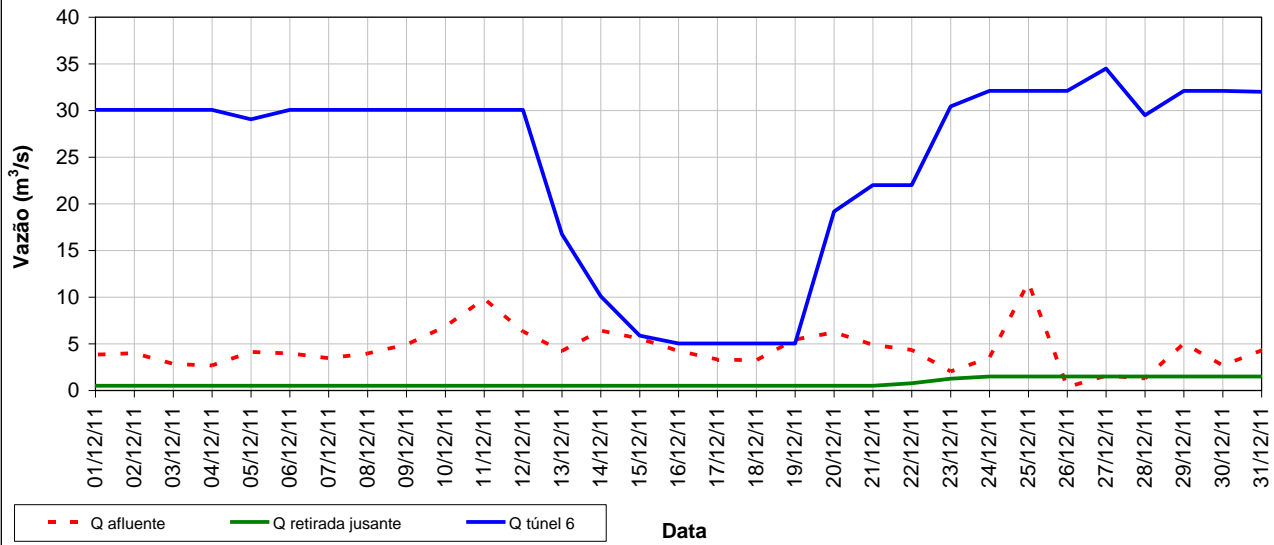
Vazões características do reservatório Cachoeira - Dez/2011
