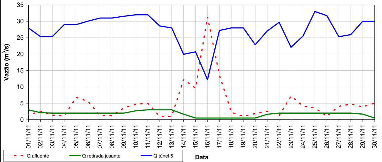
Vazões características do reservatório Atibainha - Nov/2011
