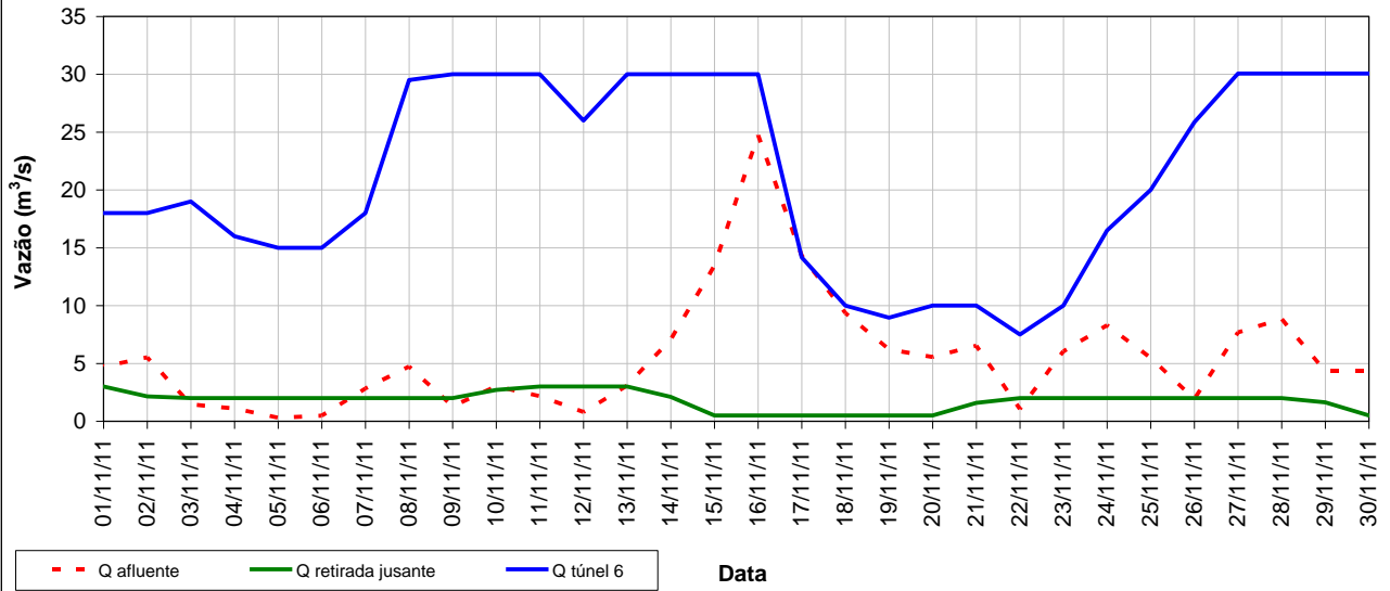
Vazões características do reservatório Cachoeira - Nov/2011
