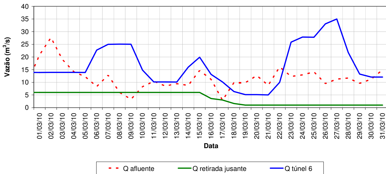
Vazões características do reservatório Cachoeira - Março/2010
