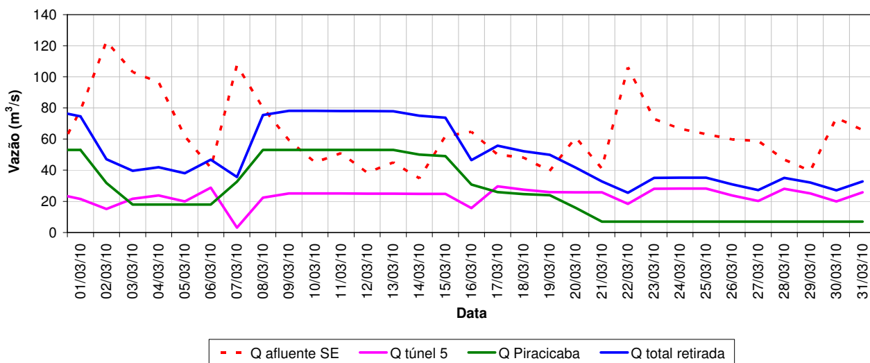
Vazões características do Sistema Cantareira - Março/2010
