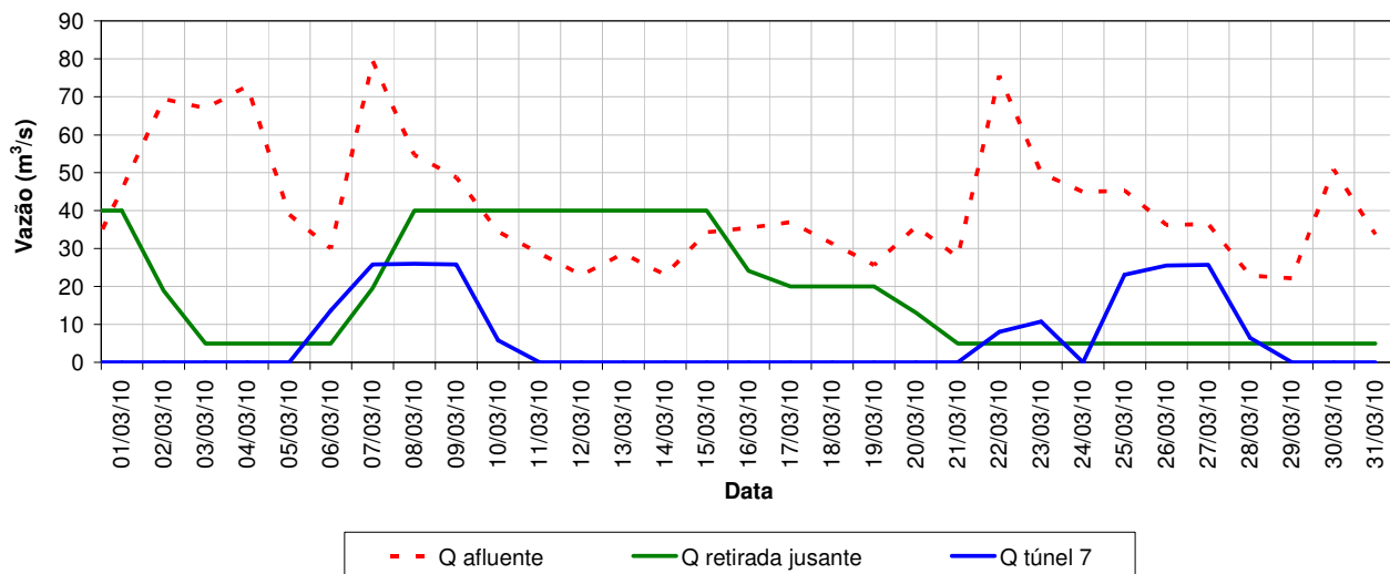
Vazões características do reservatório Jaguari-Jacareí - Março/2010
