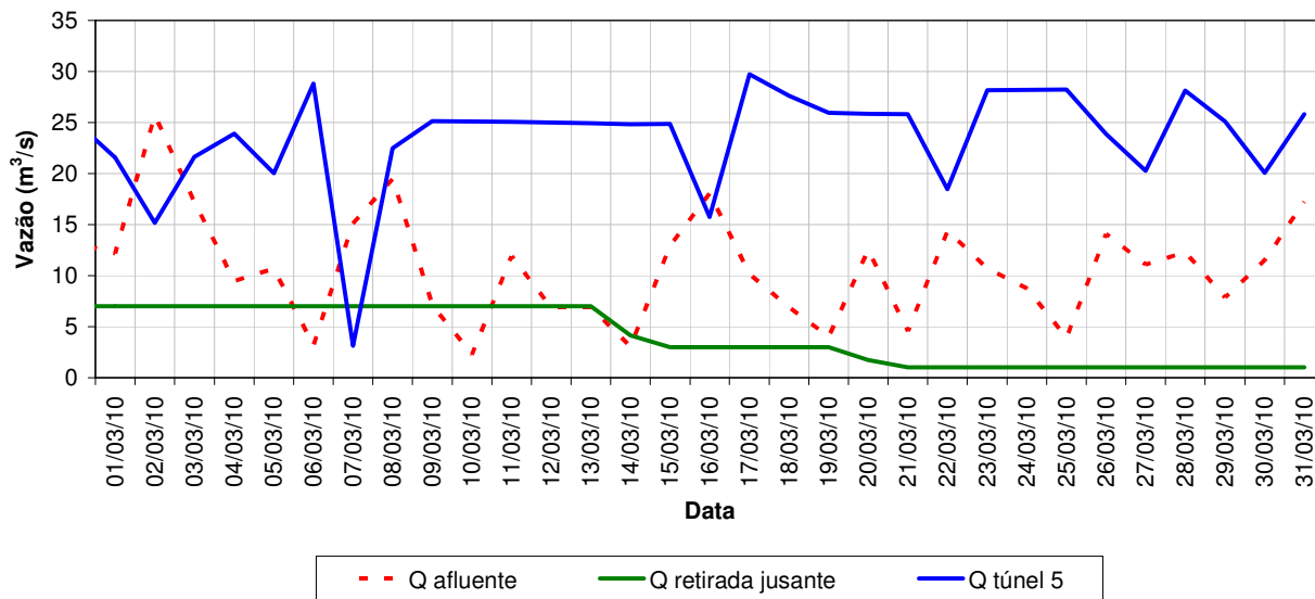
Vazões características do reservatório Atibainha - Março/2010
