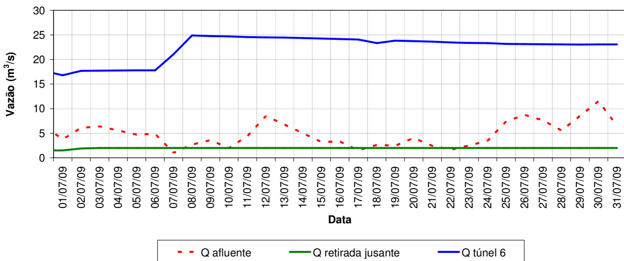
Vazões características do reservatório Cachoeira - Julho/2009
