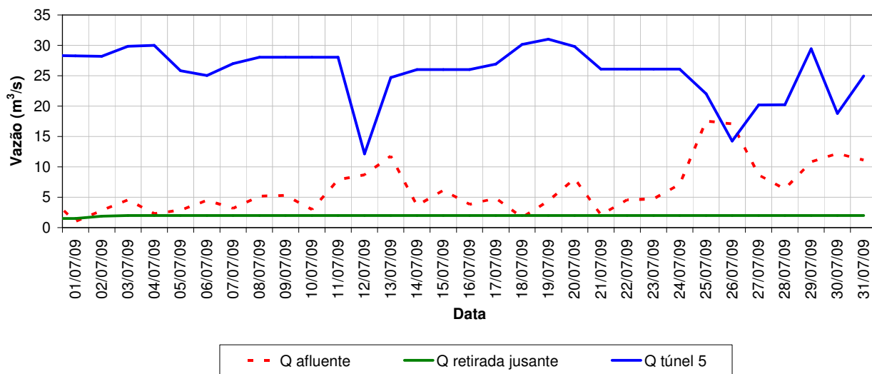
Vazões características do reservatório Atibainha - Julho/2009
