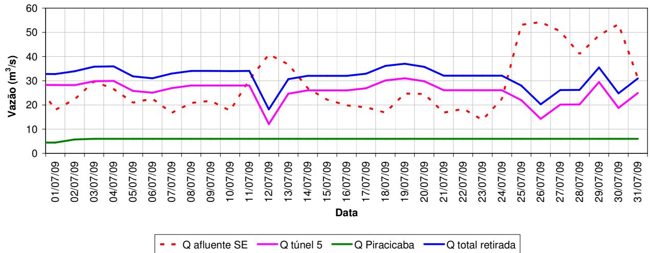
Vazões Características do Sistema Cantareira - Julho/2009
