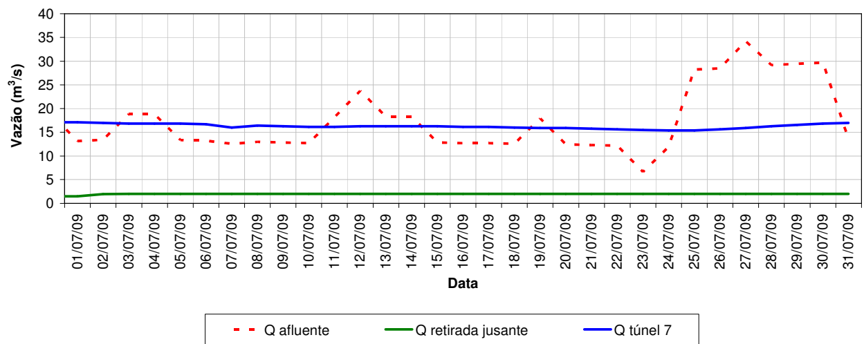
Vazões características do reservatório Jaguari-Jacareí - Julho/2009
