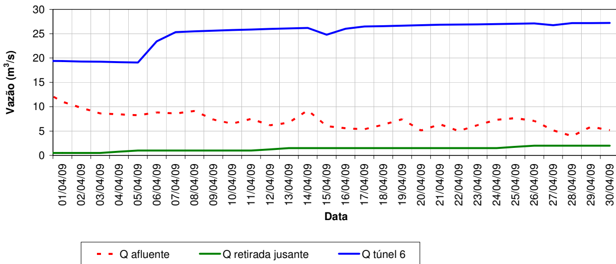
Vazões características do reservatório Cachoeira - Abril/2009
