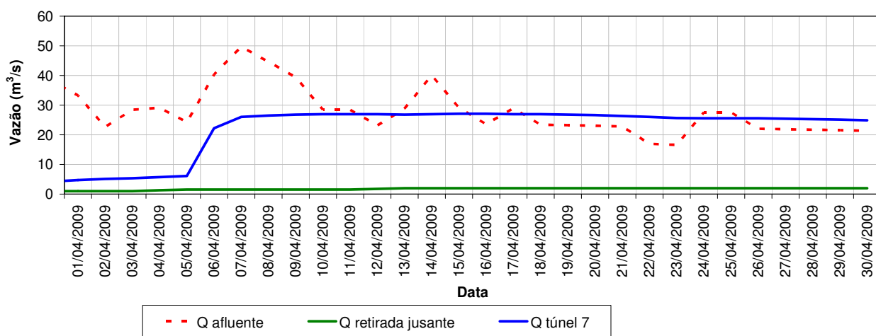
Vazões características do reservatório Jaguari-Jacaré - Abril/2009
