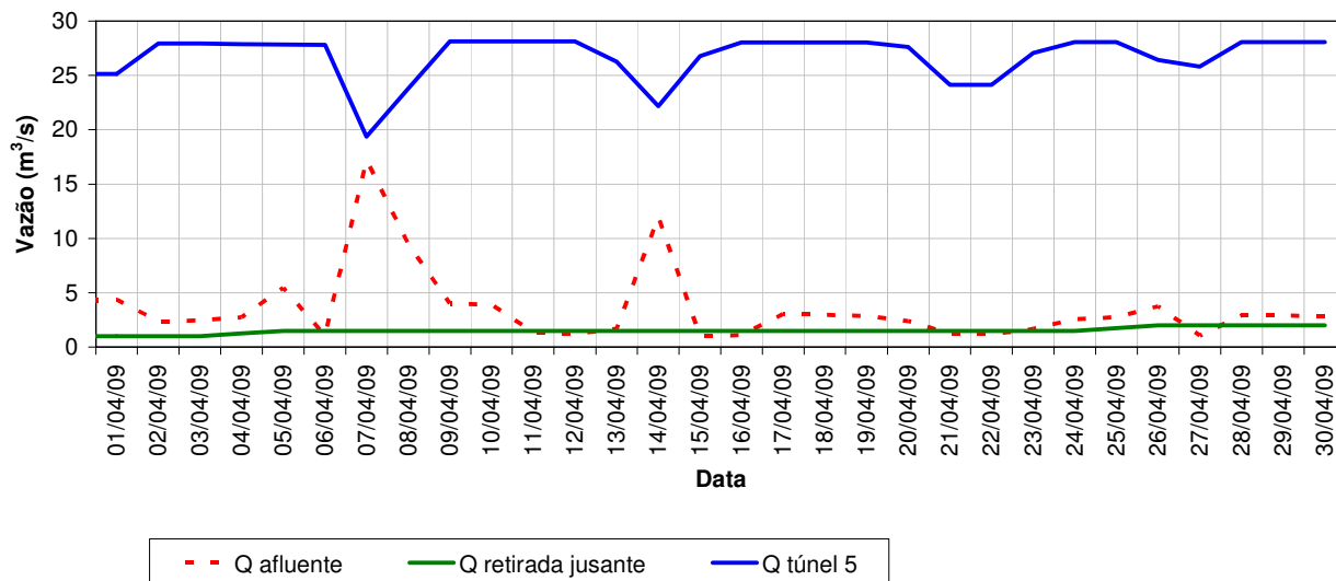
Vazões características do reservatório Atibainha - Abril/2009
