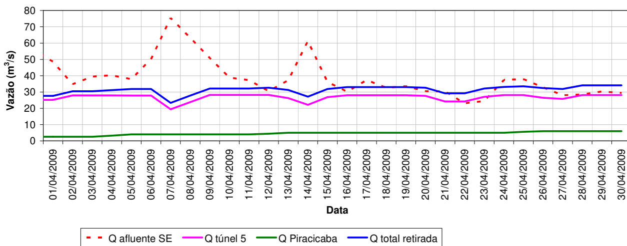
Vazões Características do Sistema Cantareira - Abril/2009
