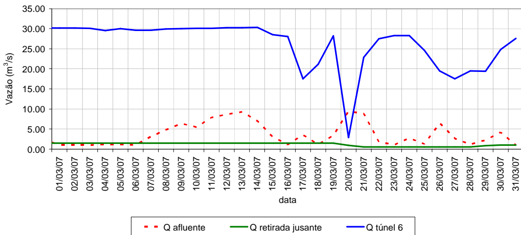
Vazões características do reservatório Cachoeira - Março/2007
