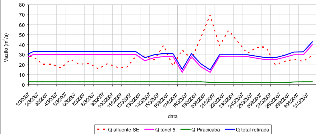
Vazões Características do Sistema Cantareira - Março/2007
