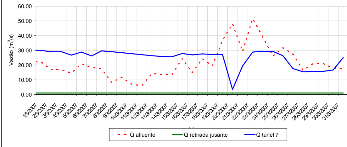
Vazões características do reservatório Jaguari-Jacareí - Março/2007
