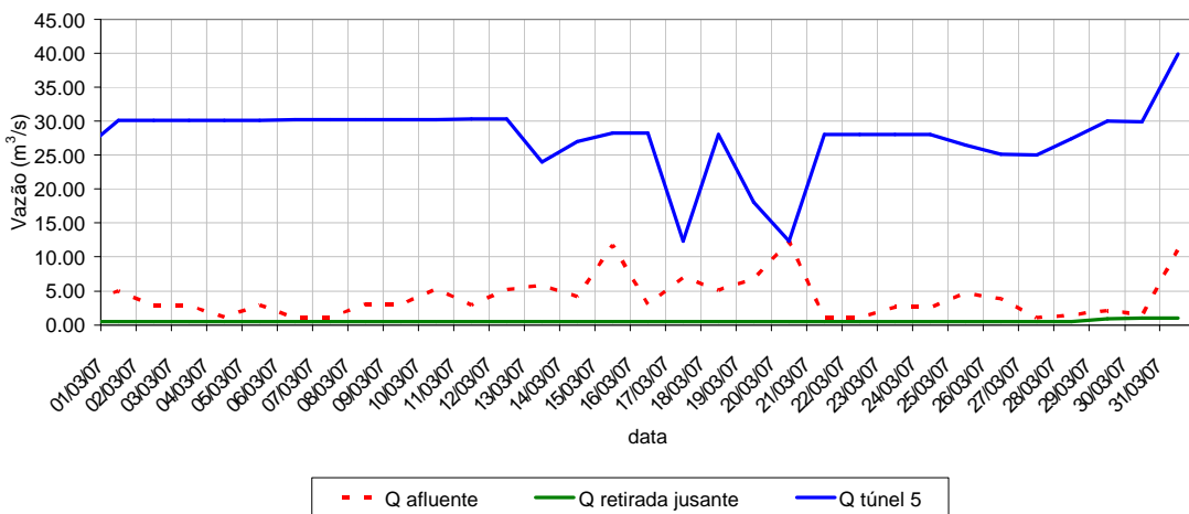
Vazões características do reservatório Atibainha - Março/2007
