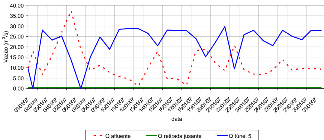
Vazões características do reservatório Atibainha - janeiro/2007
