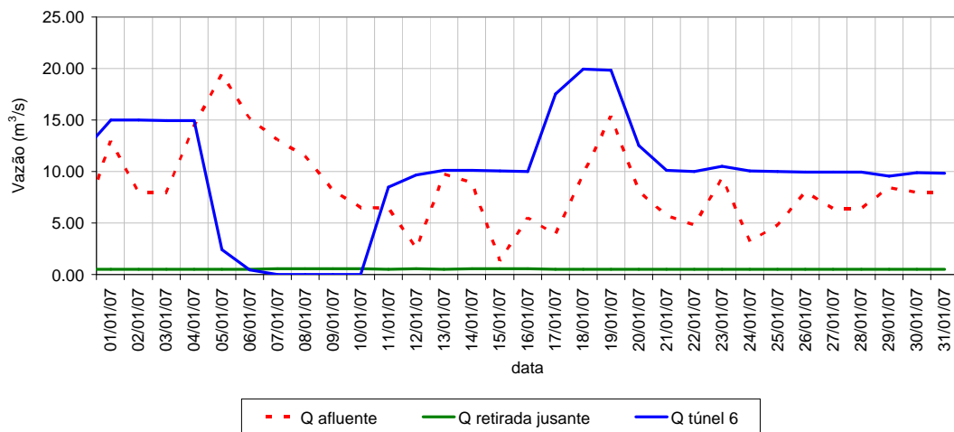
Vazões características do reservatório Cachoeira - Janeiro/2007
