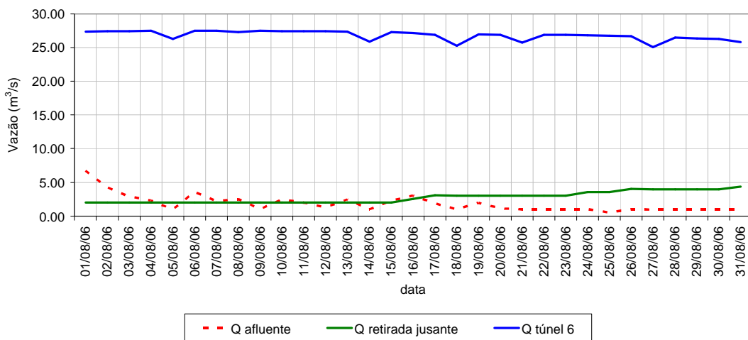
Vazões características do reservatório Cachoeira - agosto/2006
