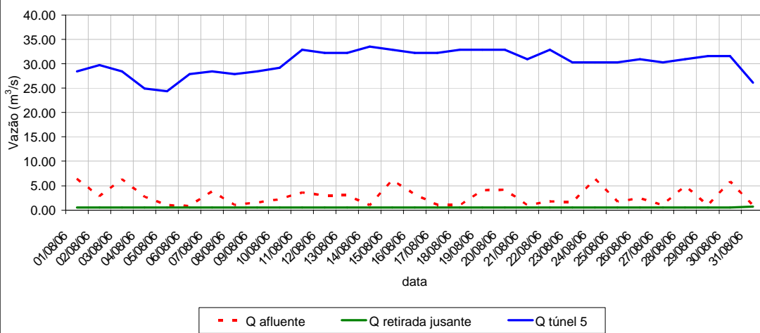
Vazões características do reservatório Atibainha - agosto/2006
