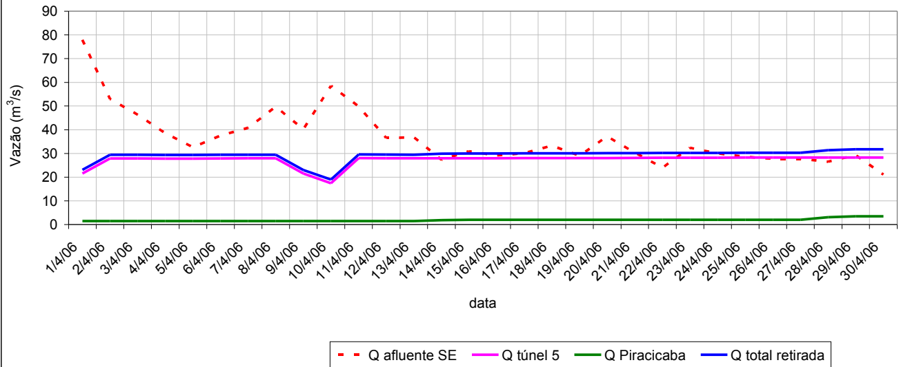
Vazões Características do Sistema Cantareira - abril/2006
