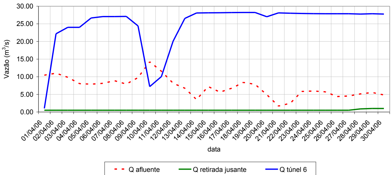
Vazões características do reservatório Cachoeira - abril/2006
