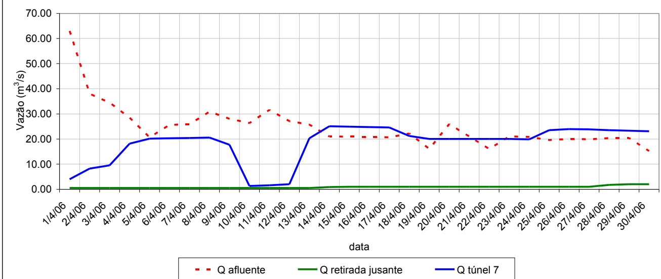
Vazões características do reservatório Jaguari-Jacareí - abril/2006
