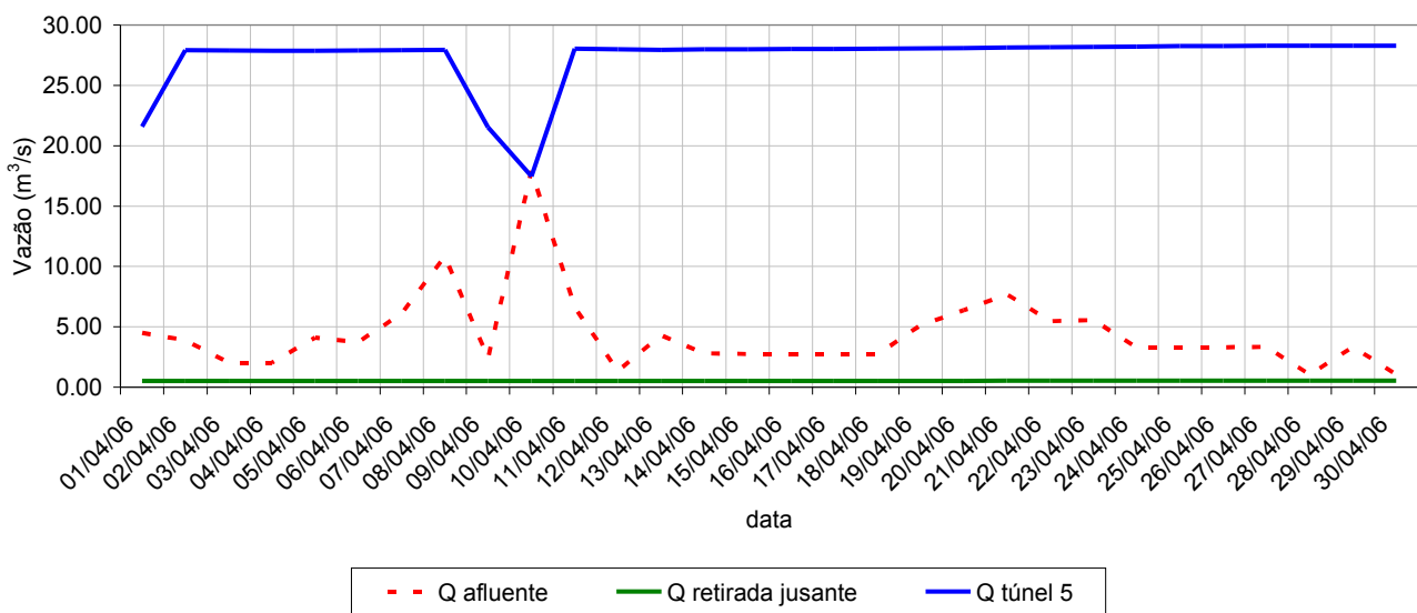
Vazões características do reservatório Atibainha - abril/2006
