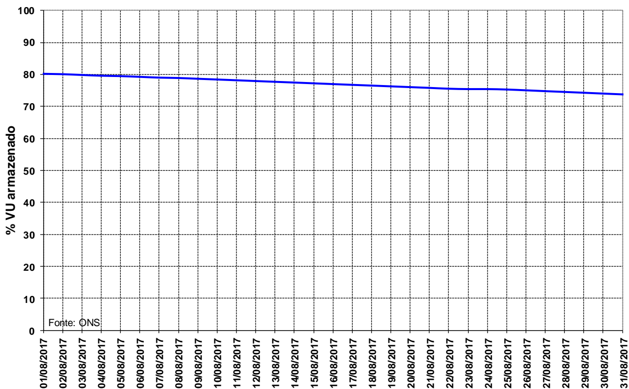
Figura 14 – Volume Útil armazenado na UHE Manso para o mês de agosto de 2017.
