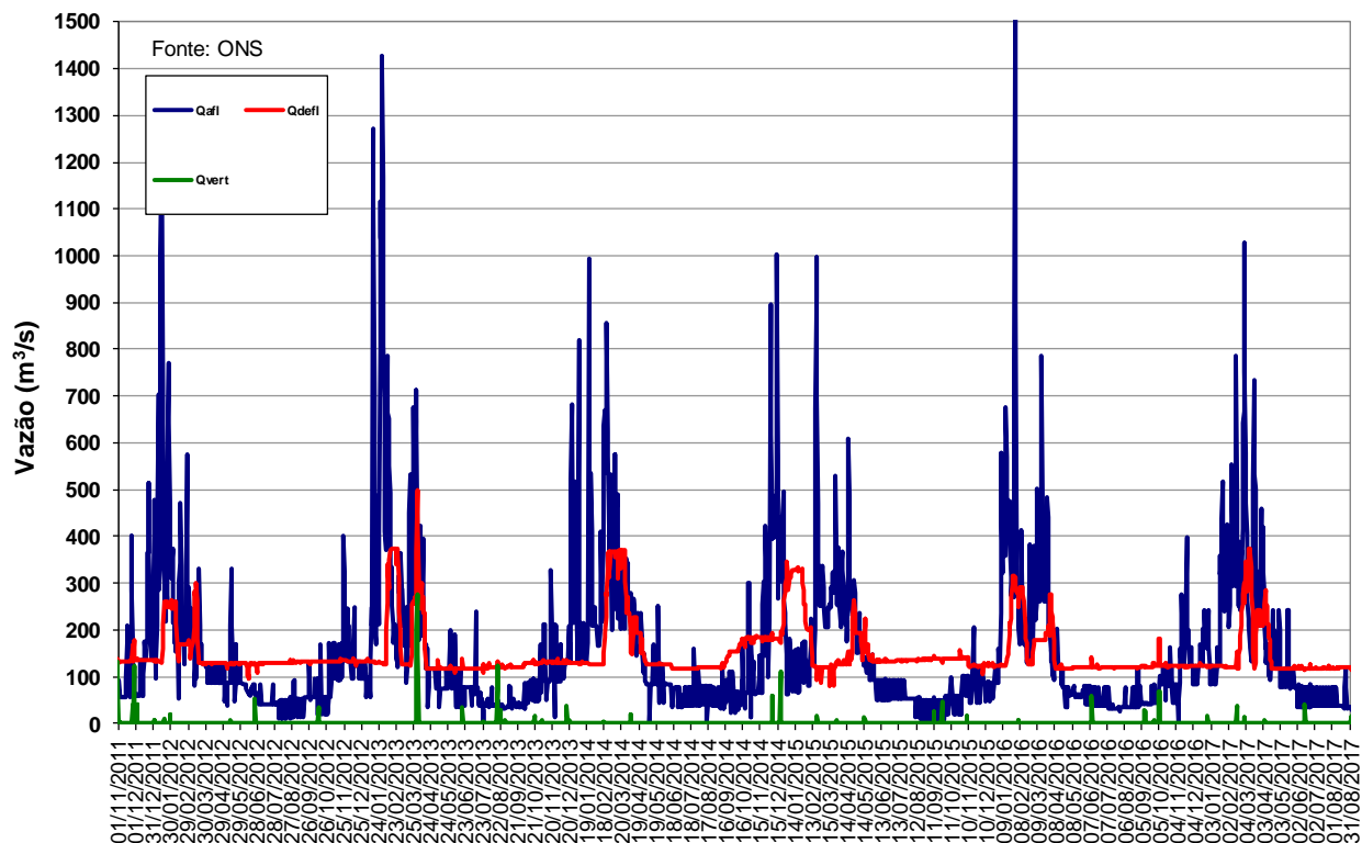
Figura 11 – Vazões na UHE Manso de novembro de 2011 a agosto de 2017.
