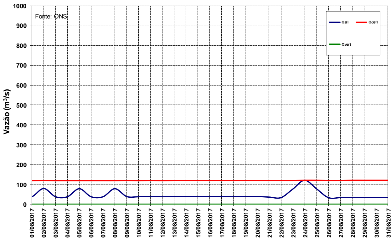
Figura 12 – Vazões na UHE Manso para o mês de agosto de 2017.
