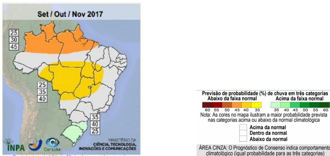
Figura 19 – Previsão climática para o trimestre set./2017 a nov./2017.
