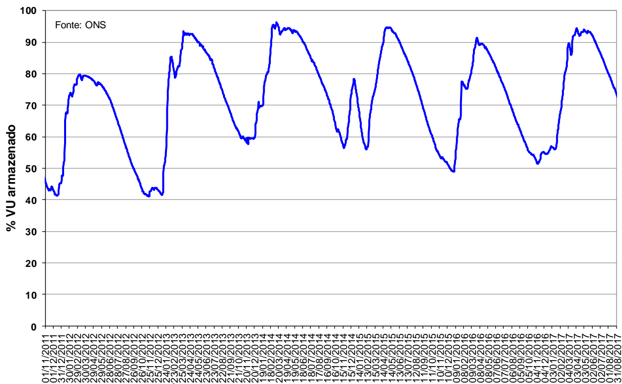
Figura 13 – Volume Útil armazenado na UHE Manso de novembro de 2011 a julho de 2017.
