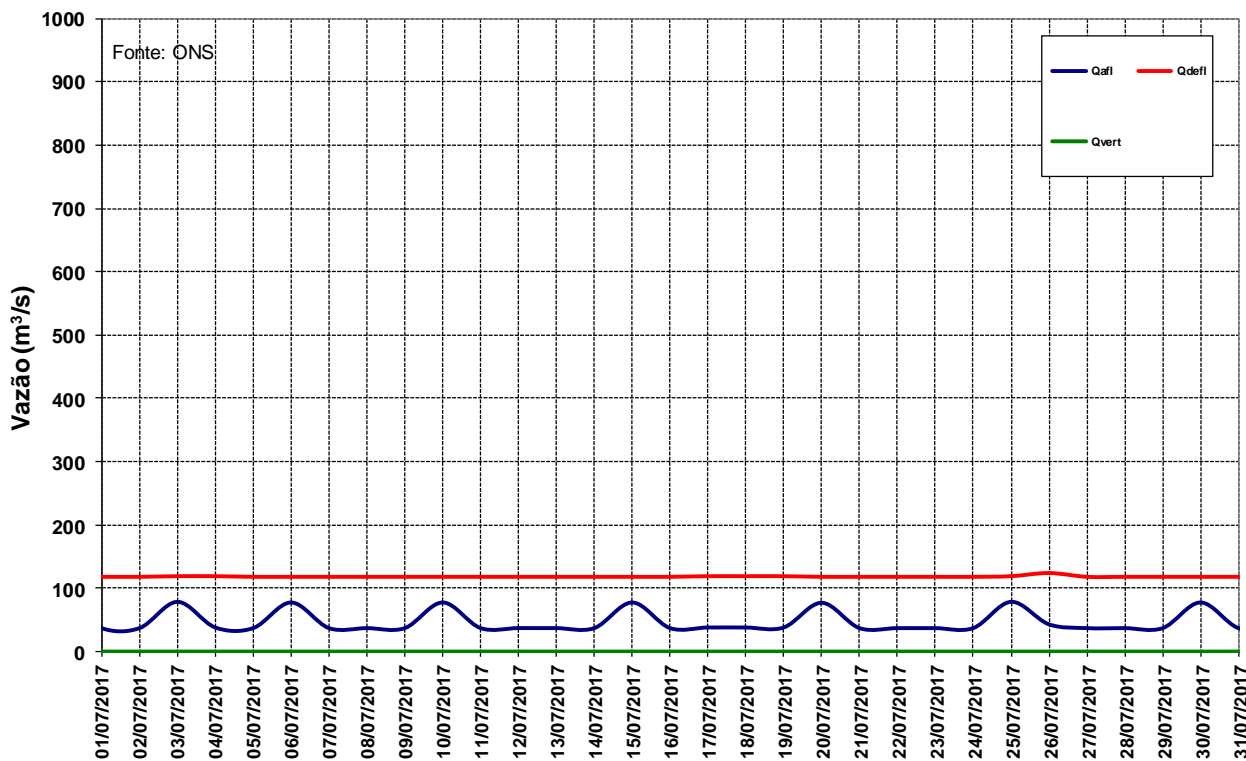
Figura 12 – Vazões na UHE Manso para o mês de julho de 2017.
