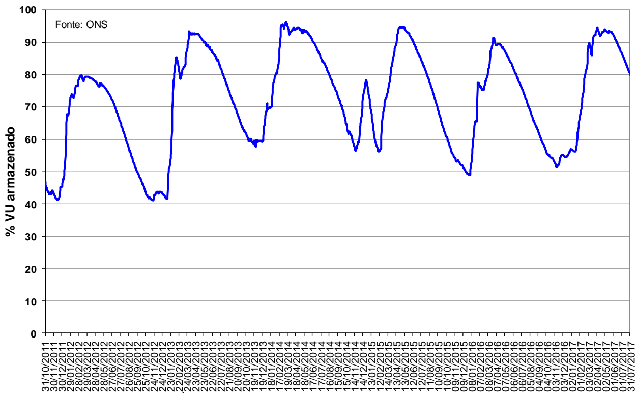
Figura 13 – Volume Útil armazenado na UHE Manso de outubro de 2011 a julho de 2017.
