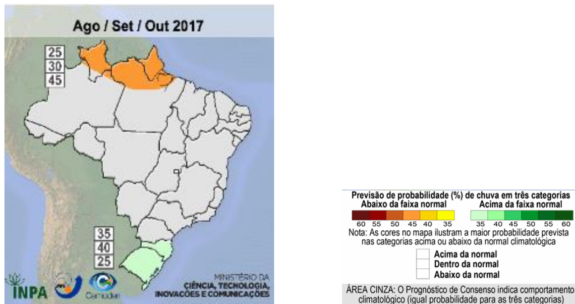
Figura 19 – Previsão climática para o trimestre ago./2017 a out./2017.
