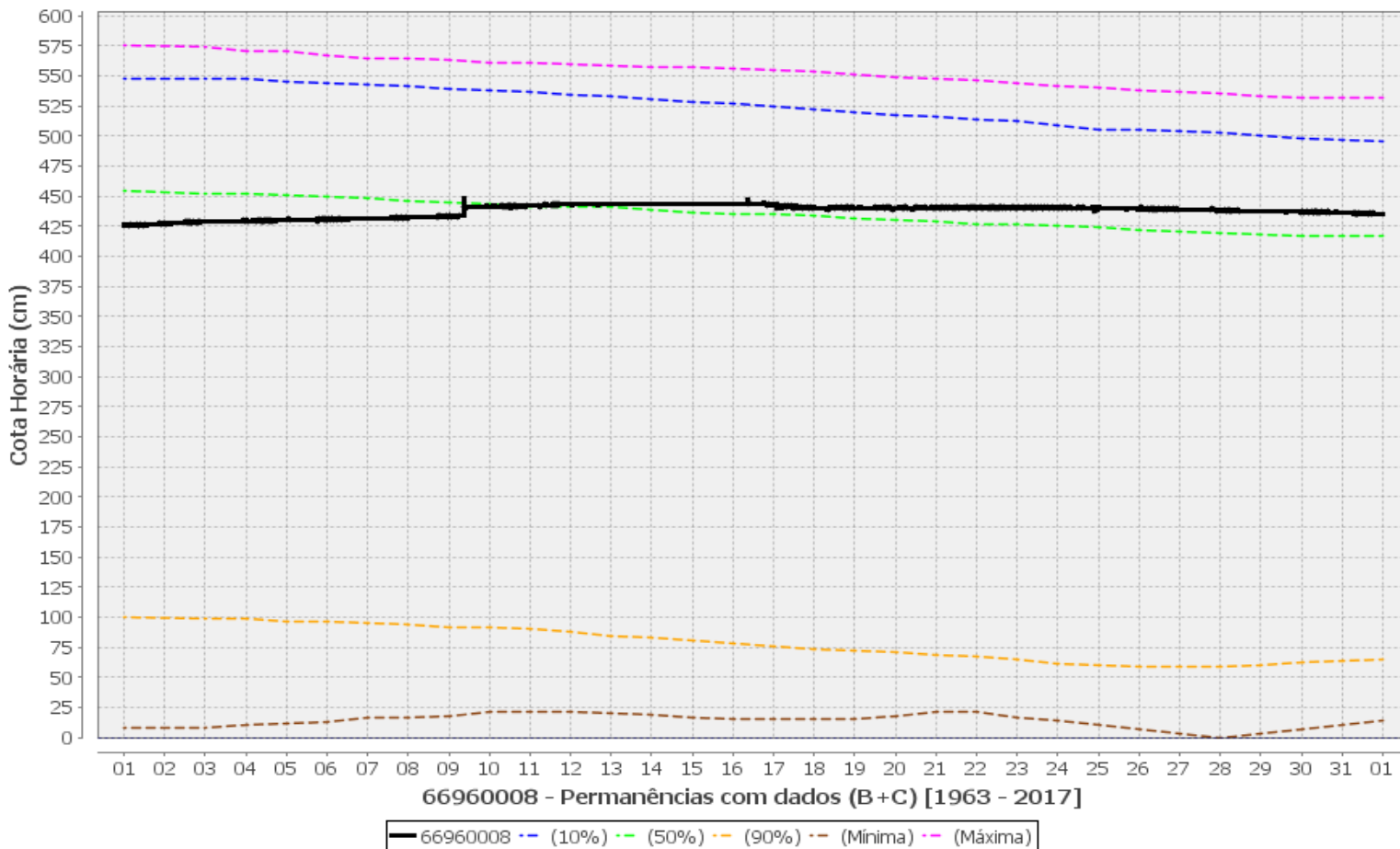
Figura 8 - Gráficos de permanência de cotas, cotas máximas, mínimas e observadas no rio Paraguai, em Porto Esperança.
