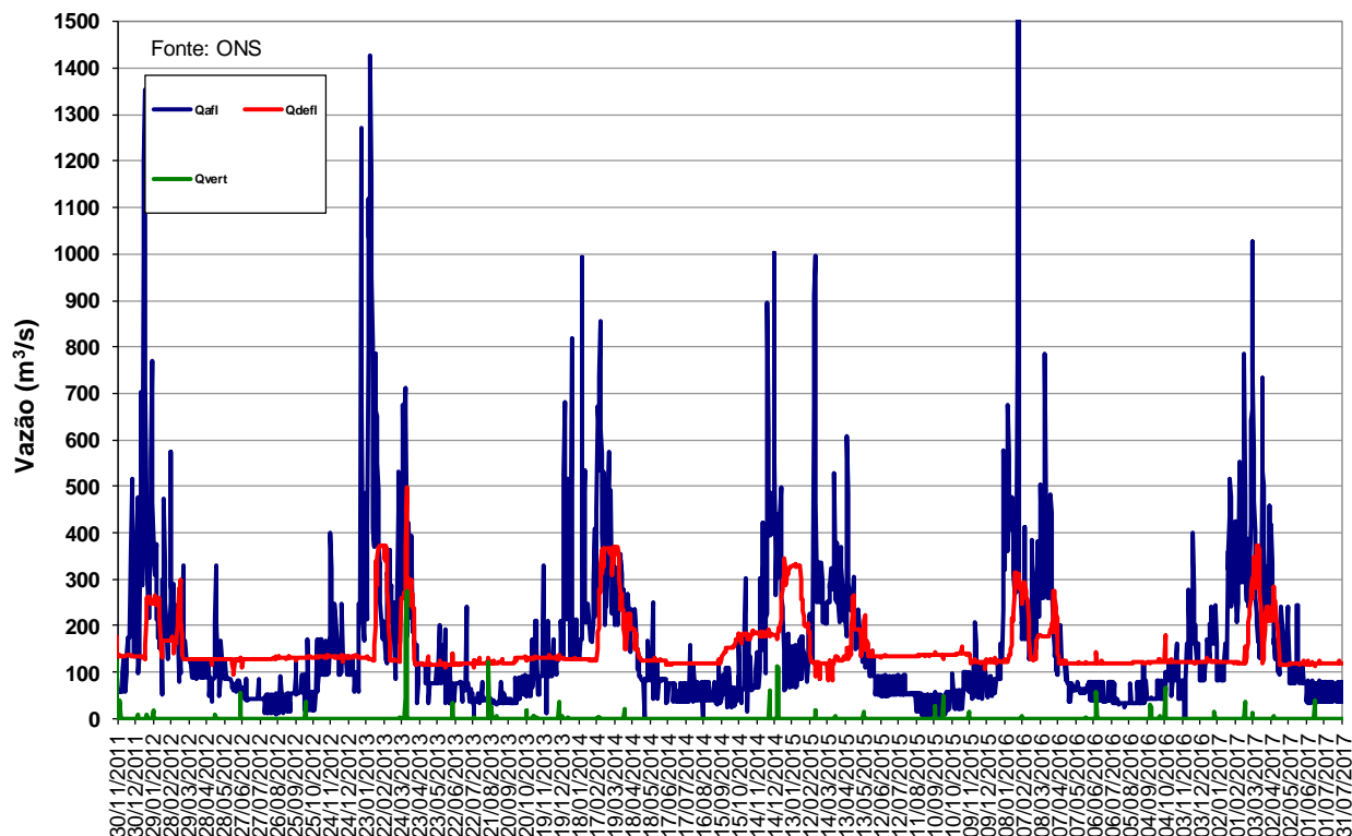
Figura 11 – Vazões na UHE Manso de novembro de 2011 a julho de 2017.
