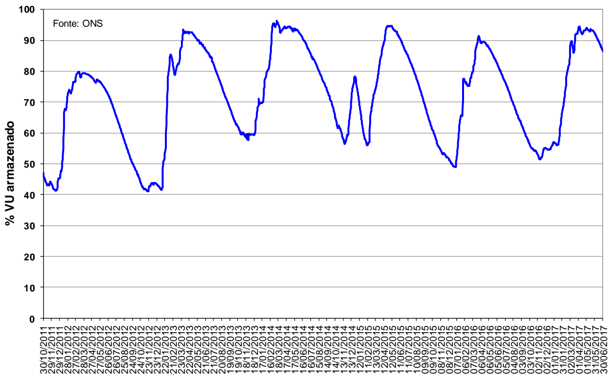
Figura 13 – Volume Útil armazenado na UHE Manso de outubro de 2011 a junho de 2017.
