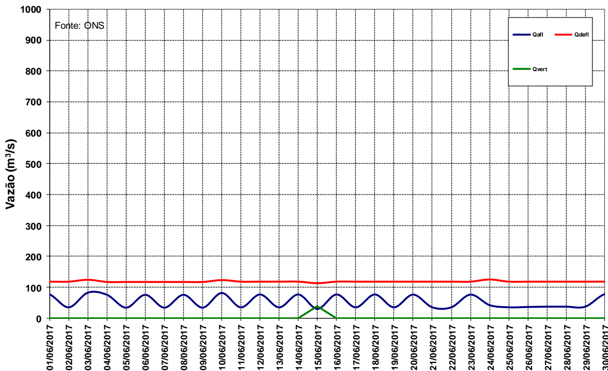
Figura 12 – Vazões na UHE Manso para o mês de junho de 2017.
