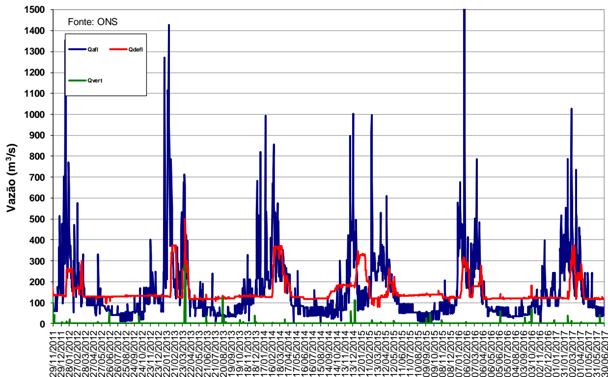
Figura 11 – Vazões na UHE Manso de novembro de 2011 a junho de 2017.
