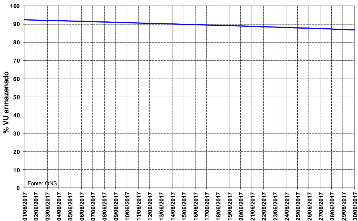
Figura 14 – Volume Útil armazenado na UHE Manso para o mês de junho de 2017.
