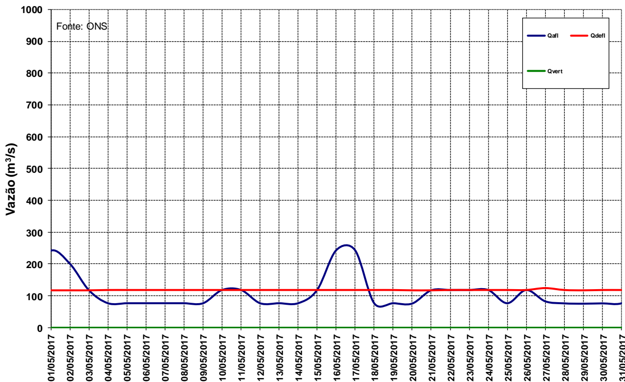
Figura 12 – Vazões na UHE Manso para o mês de maio de 2017.
