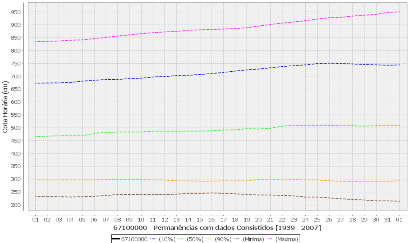
Figura 9 - Gráficos de permanência de cotas, cotas máximas, mínimas e observadas no rio Paraguai, em Porto Murtinho.
