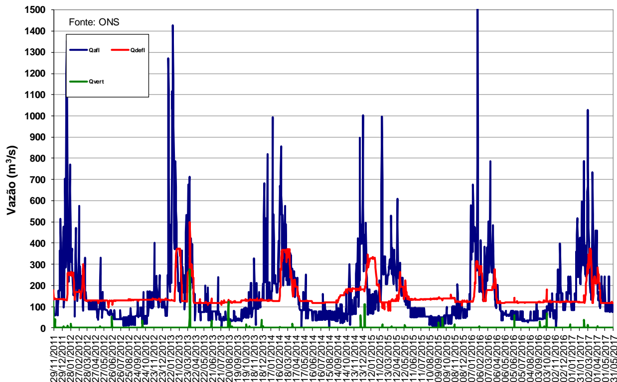
Figura 11 – Vazões na UHE Manso de novembro de 2011 a maio de 2017.
