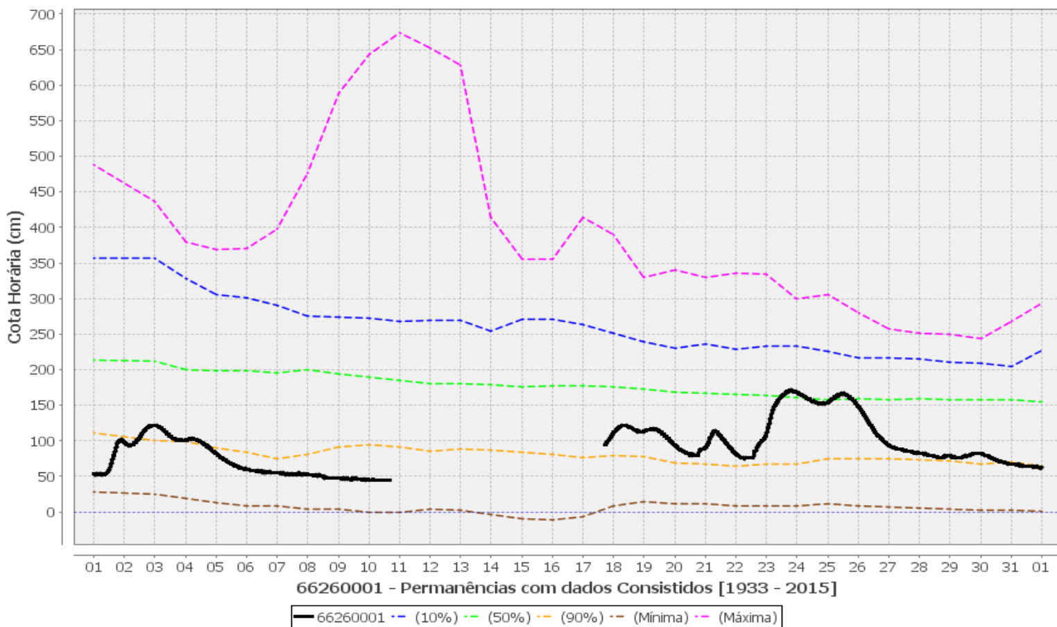
Figura 5 – Gráficos de permanência de cotas, cotas máximas, mínimas e observadas no rio Cuiabá, em Cuiabá.
