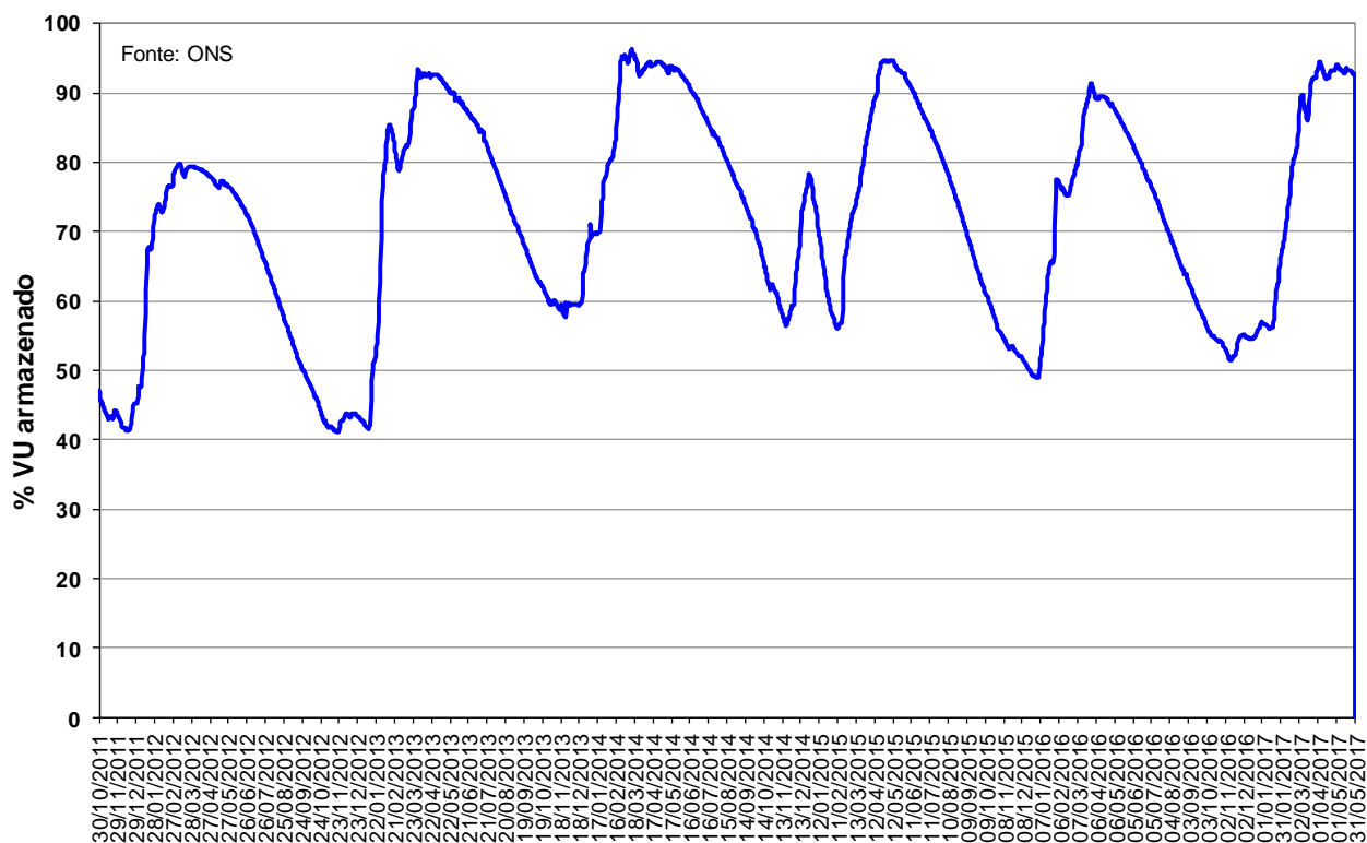
Figura 13 – Volume Útil armazenado na UHE Manso de outubro de 2011 a maio de 2017.
