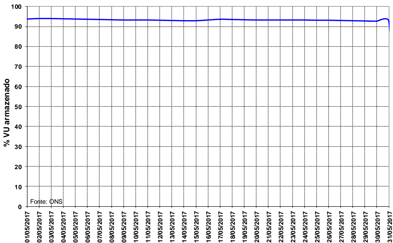
Figura 14 – Volume Útil armazenado na UHE Manso para o mês de maio de 2017.
