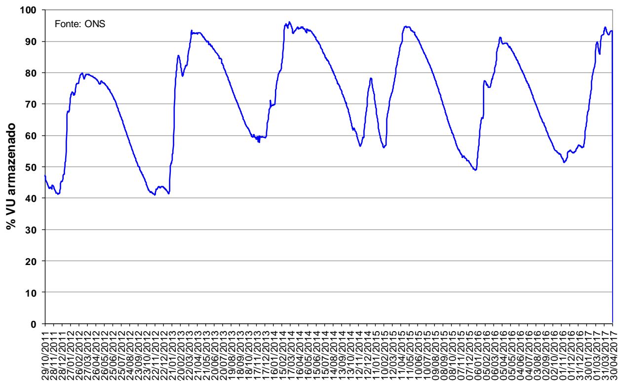
Figura 13 – Volume Útil armazenado na UHE Manso de outubro de 2011 a abril de 2017.
