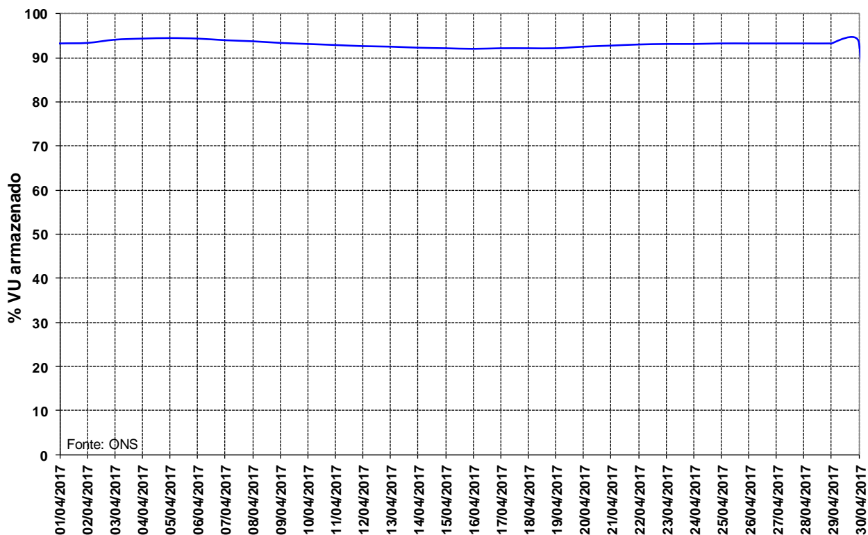
Figura 14 – Volume Útil armazenado na UHE Manso para o mês de abril de 2017.
