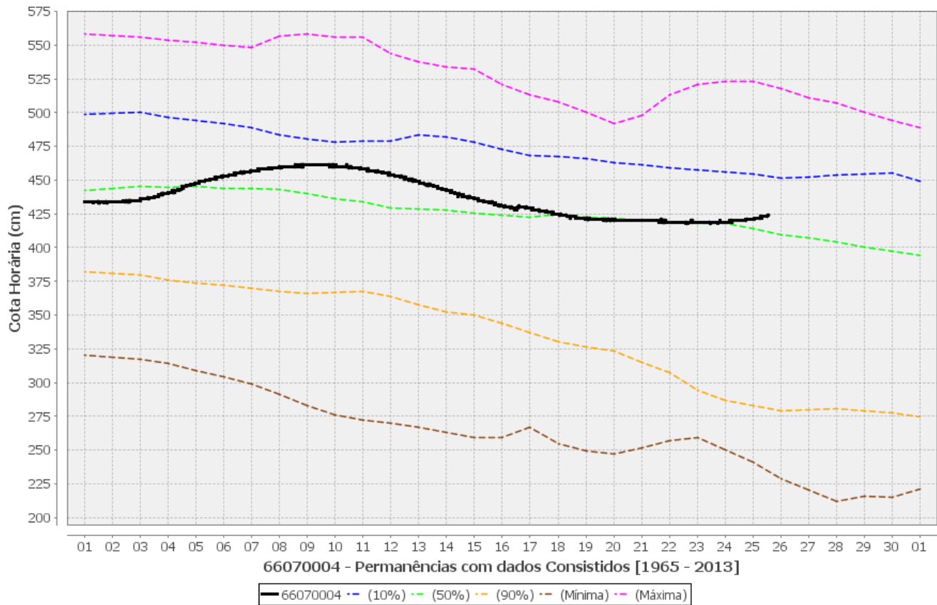
Figura 7 - Gráficos de permanência de cotas, cotas máximas, mínimas e observadas no rio Paraguai, em Cáceres.
