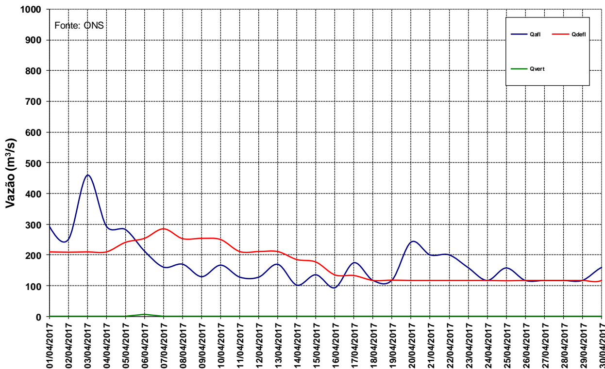
Figura 12 – Vazões na UHE Manso para o mês de abril de 2017.
