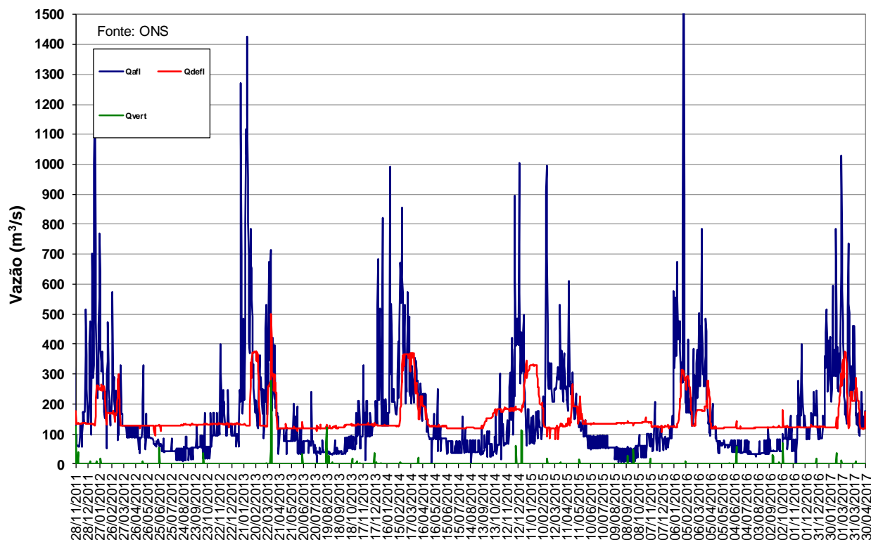
Figura 11 – Vazões na UHE Manso de novembro de 2011 a abril de 2017.
