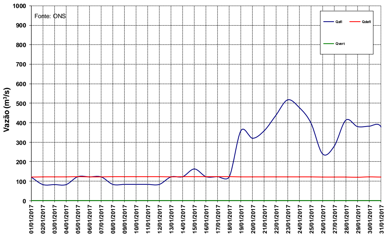
Figura 12 – Vazões na UHE Manso para o mês de janeiro de 2017.
