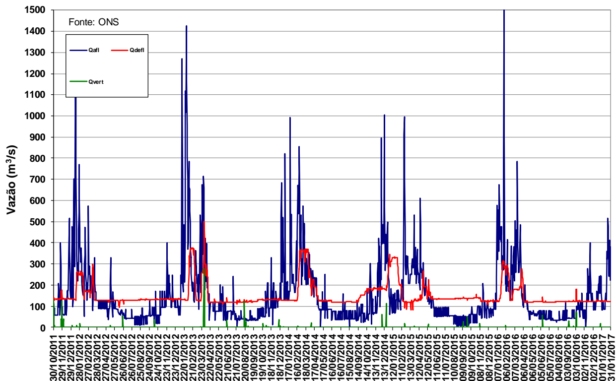
Figura 11 – Vazões na UHE Manso de outubro de 2011 a janeiro de 2017.
