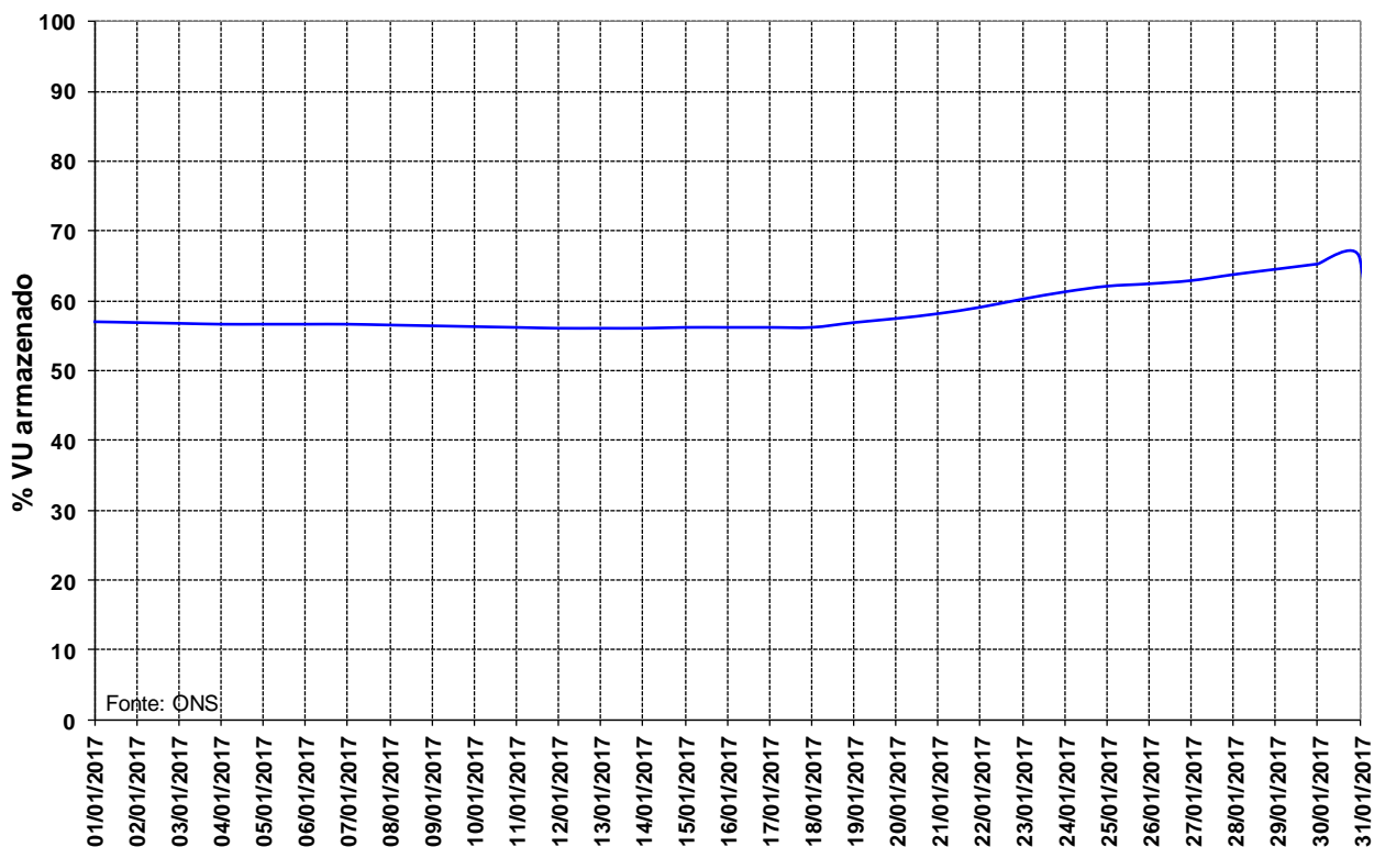
Figura 14 – Volume Útil armazenado na UHE Manso para o mês de janeiro de 2017.
