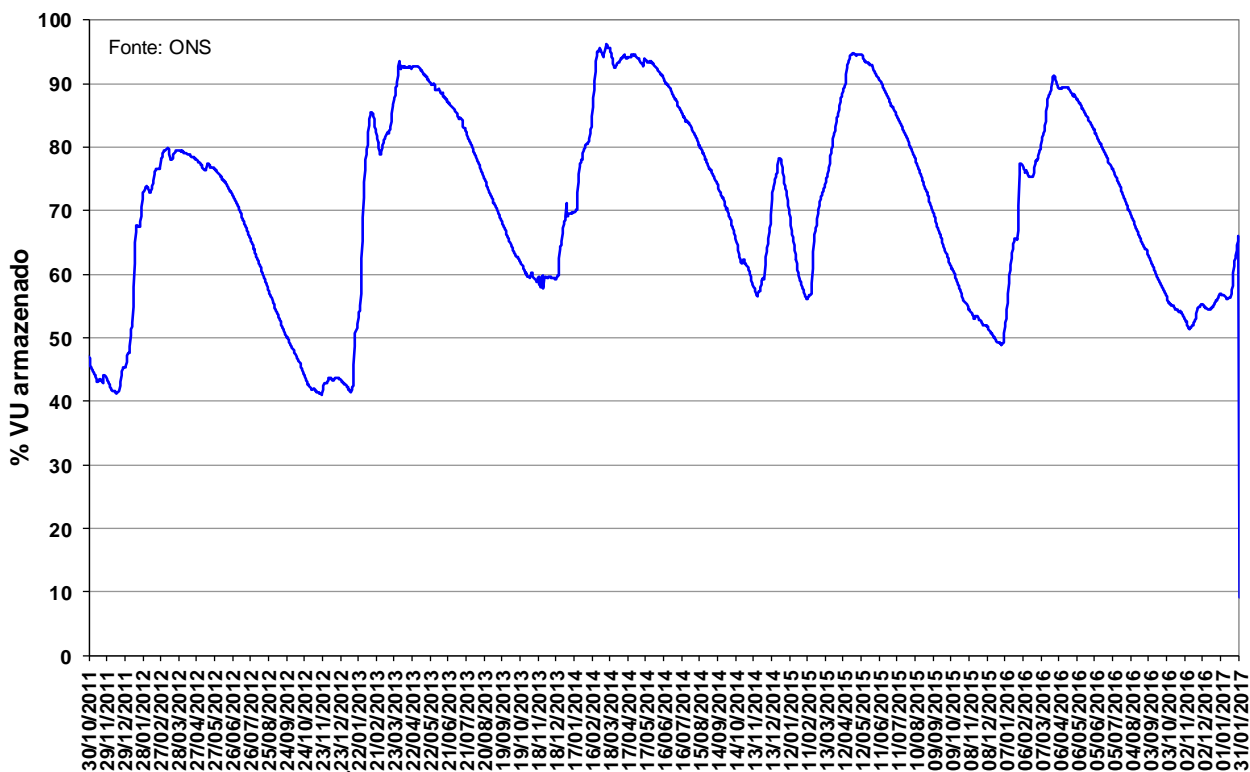
Figura 13 – Volume Útil armazenado na UHE Manso de outubro de 2011 a janeiro de 2017.
