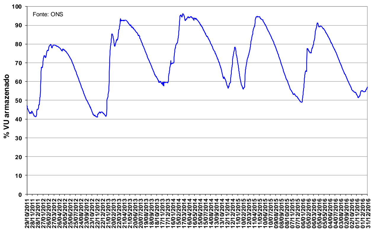
Figura 13 – Volume Útil armazenado na UHE Manso de outubro de 2011 a dezembro de 2016.
