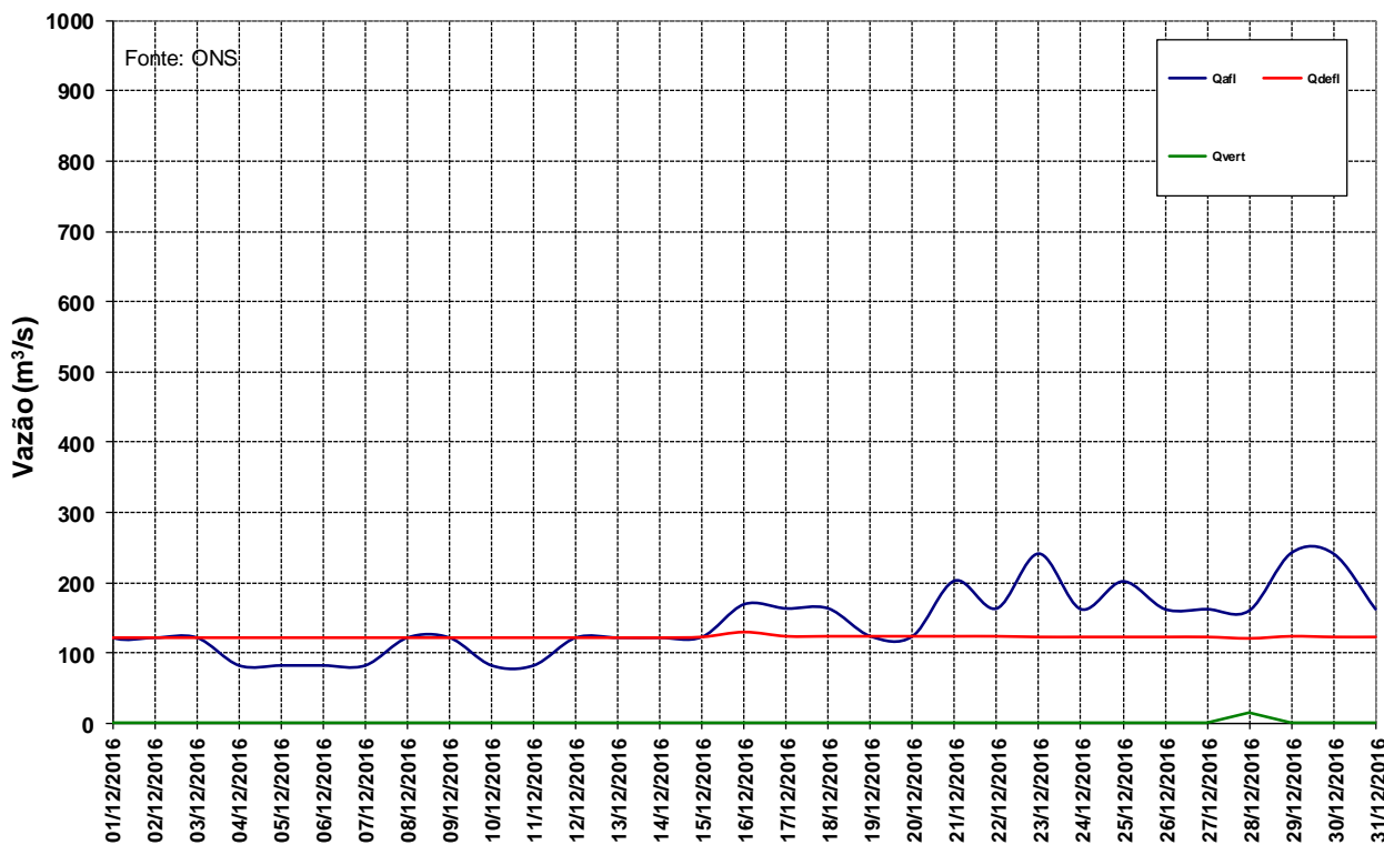
Figura 12 – Vazões na UHE Manso para o mês de dezembro de 2016.
