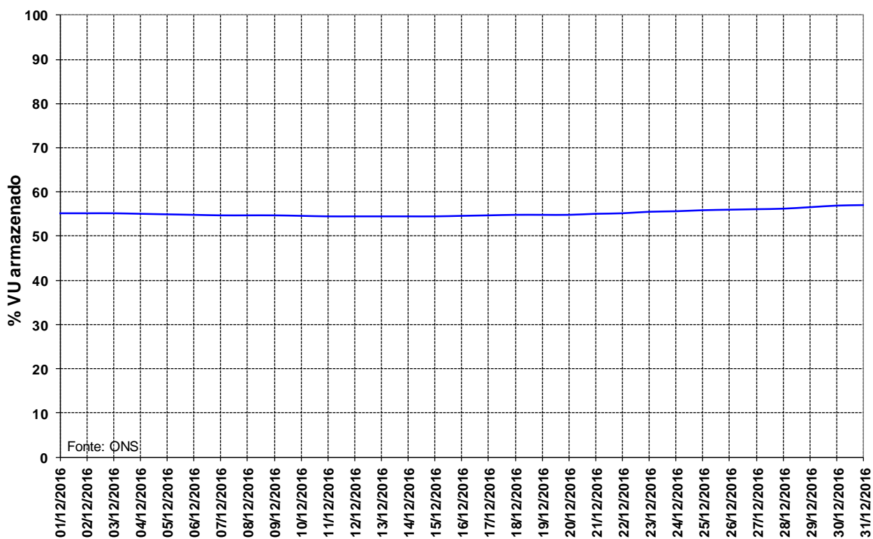
Figura 14 – Volume Útil armazenado na UHE Manso para o mês de dezembro de 2016.
