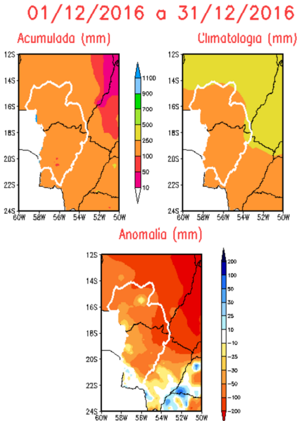
Figura 16 – Precipitação mensal acumulada, média climatológica e anomalia de precipitação na BAP, no período de 01/12/16 a 31/12/16.
