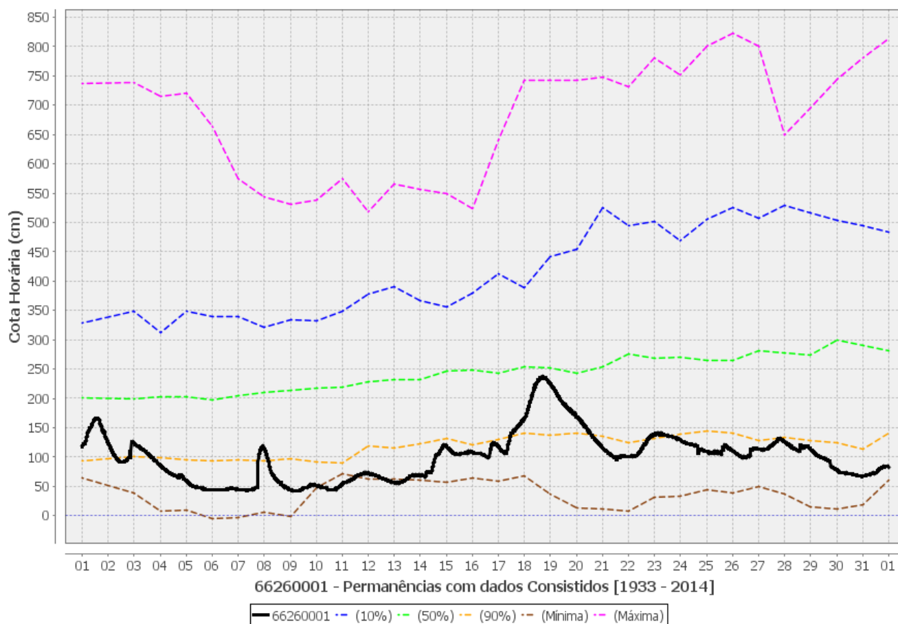
Figura 5 – Gráficos de permanência de cotas, cotas máximas, mínimas e observadas no rio Cuiabá, em Cuiabá.
