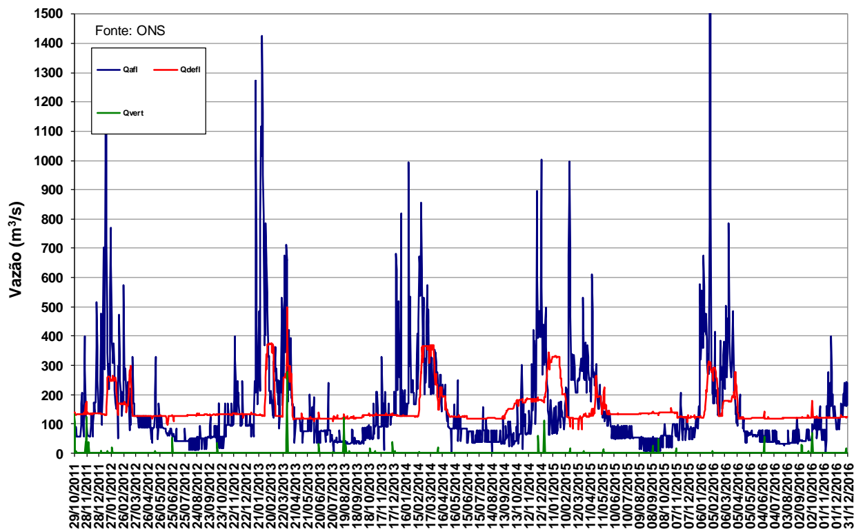
Figura 11 – Vazões na UHE Manso de outubro de 2011 a dezembro de 2016.
