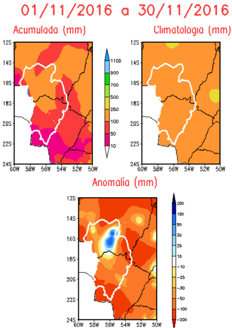
Figura 15 – Precipitação mensal acumulada, média climatológica e anomalia de precipitação na BAP, no período de 01/11/16 a 30/11/16.
