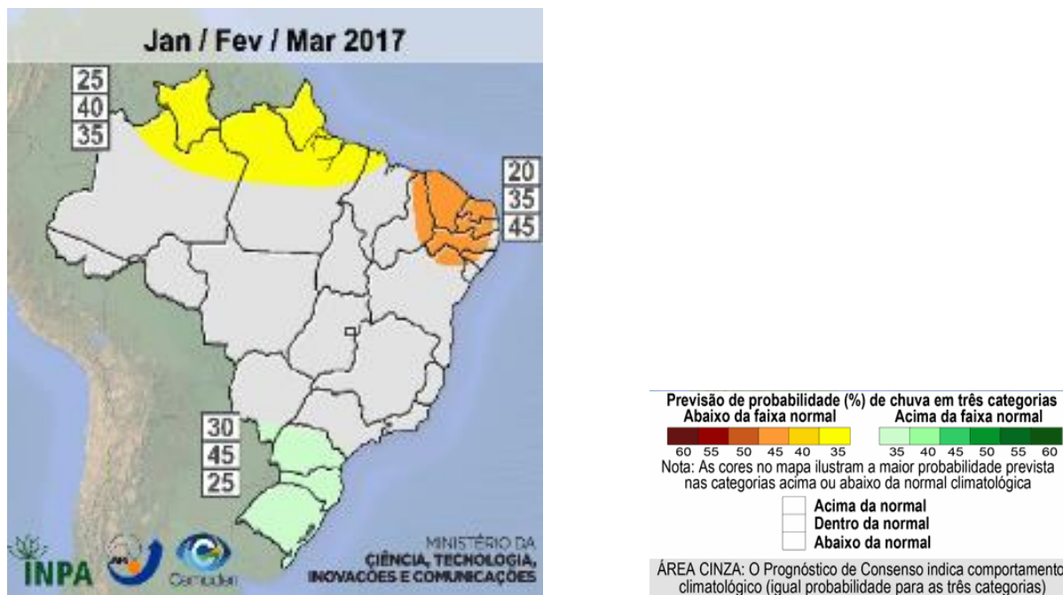
Figura 19 – Previsão climática para o trimestre Jan../2017 a março./2017.
