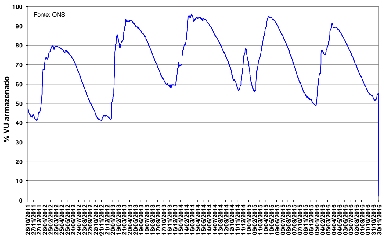
Figura 13 – Volume Útil armazenado na UHE Manso de outubro de 2011 a novembro de 2016.
