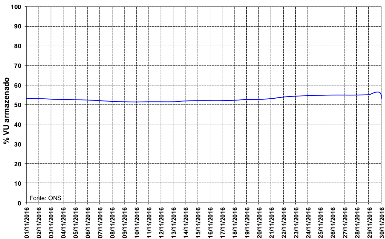
Figura 14 – Volume Útil armazenado na UHE Manso para o mês de novembro de 2016.
