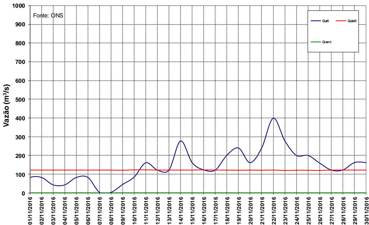
Figura 12 – Vazões na UHE Manso para o mês de novembro de 2016.
