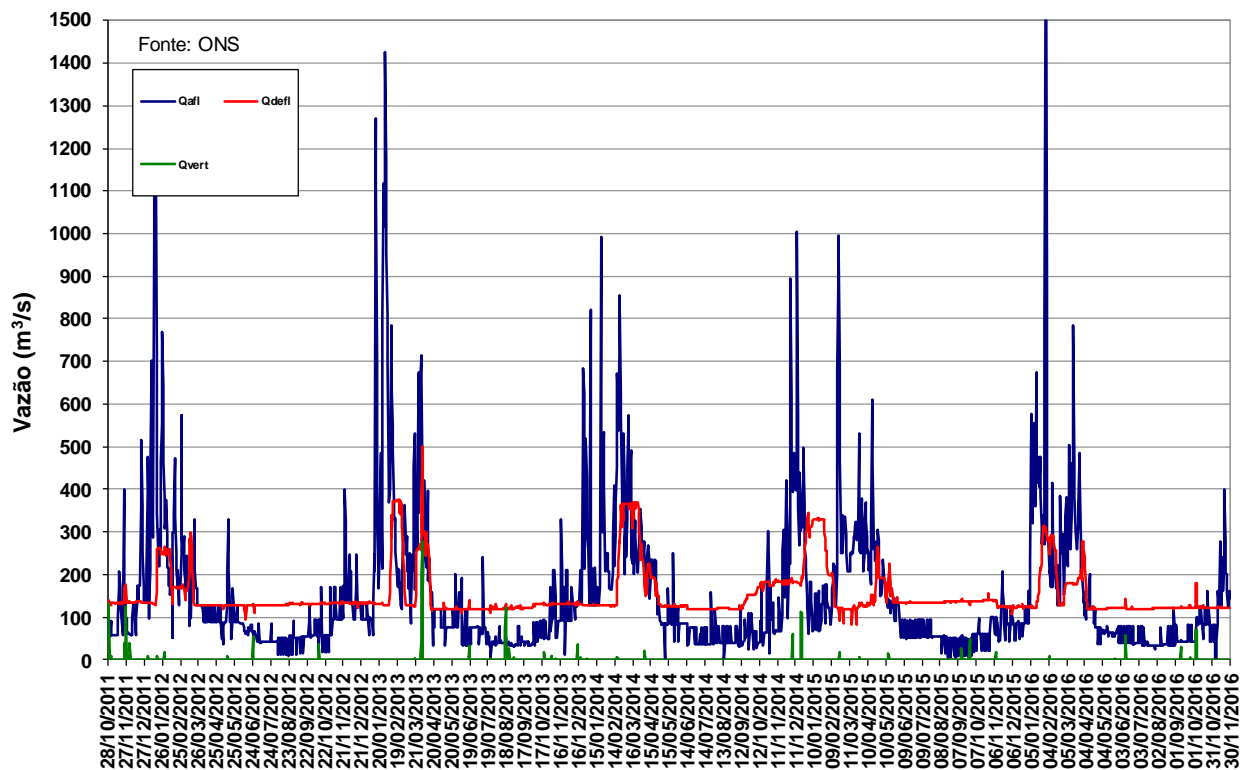
Figura 11 – Vazões na UHE Manso de outubro de 2011 a novembro de 2016.
