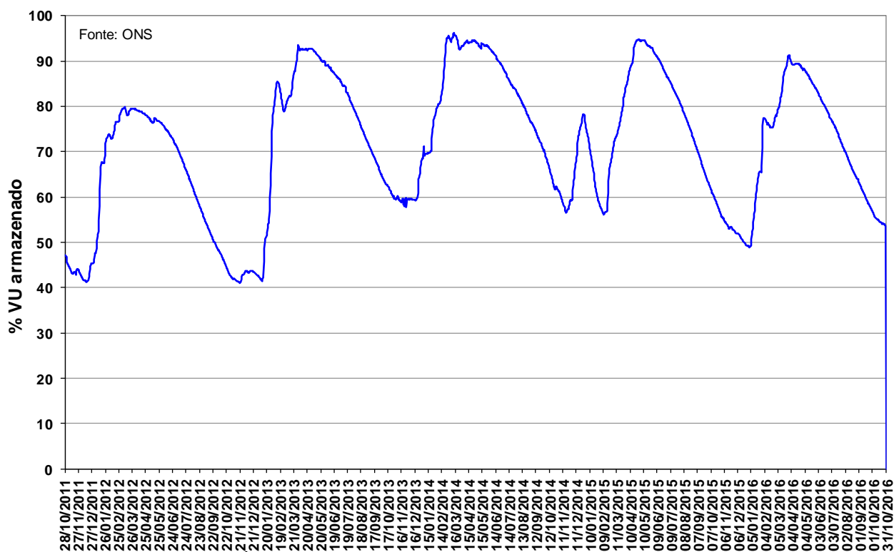
Figura 13 – Volume Útil armazenado na UHE Manso de outubro de 2011 a outubro de 2016.
