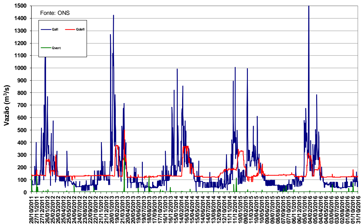
Figura 11 – Vazões na UHE Manso de outubro de 2011 a outubro de 2016.
