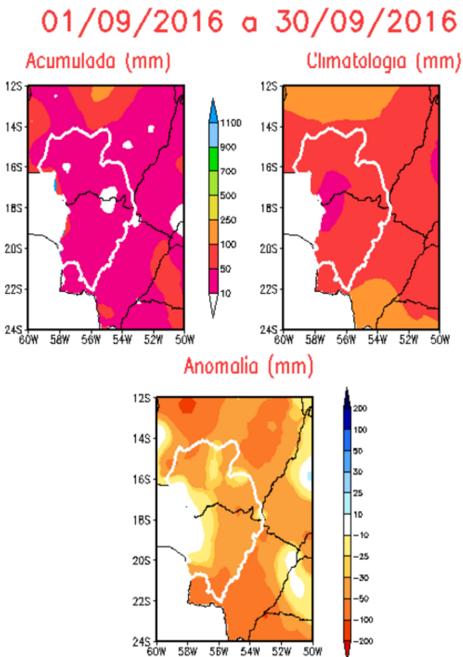
Figura 15 – Precipitação mensal acumulada, média climatológica e anomalia de precipitação na BAP, no período de 01/09/16 a 30/09/16.
