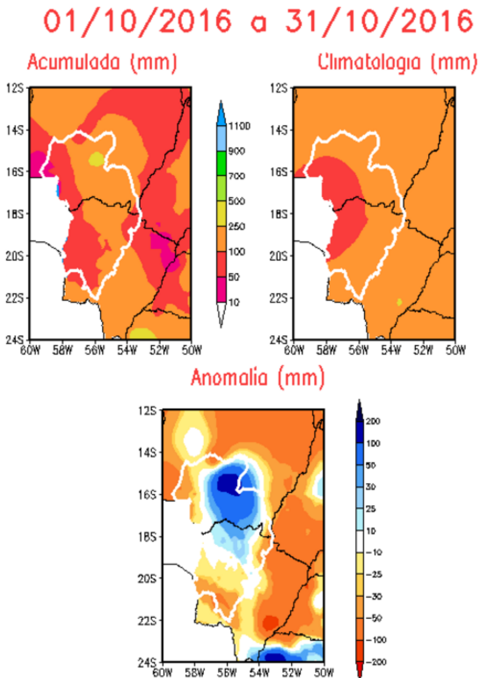
Figura 16 – Precipitação mensal acumulada, média climatológica e anomalia de precipitação na BAP, no período de 01/10/16 a 31/10/16.
