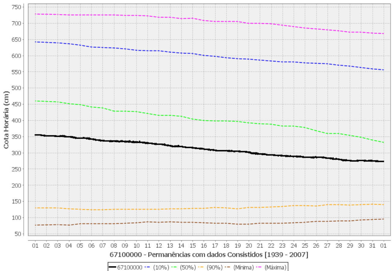
Figura 9 - Gráficos de permanência de cotas, cotas máximas, mínimas e observadas no rio Paraguai, em Porto Murtinho.
