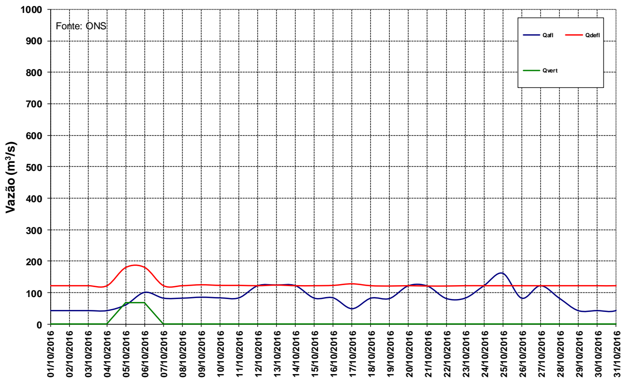
Figura 12 – Vazões na UHE Manso para o mês de outubro de 2016.
