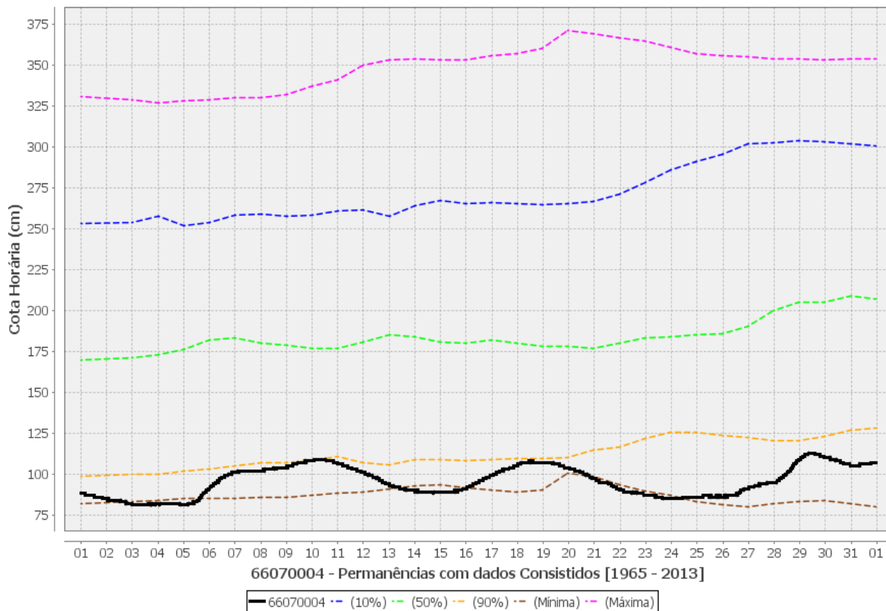
Figura 7 - Gráficos de permanência de cotas, cotas máximas, mínimas e observadas no rio Paraguai, em Cáceres.
