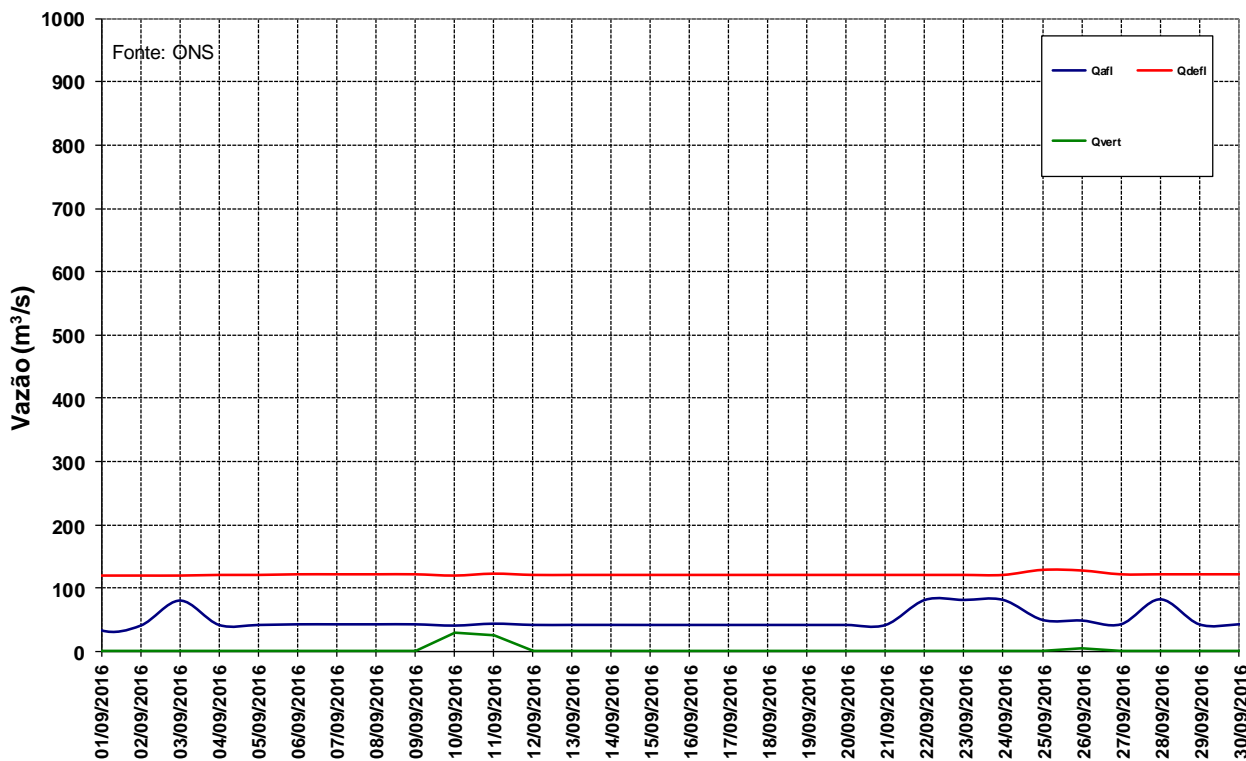
Fonte: ONS Figura 12 – Vazões na UHE Manso para o mês de setembro de 2016.
