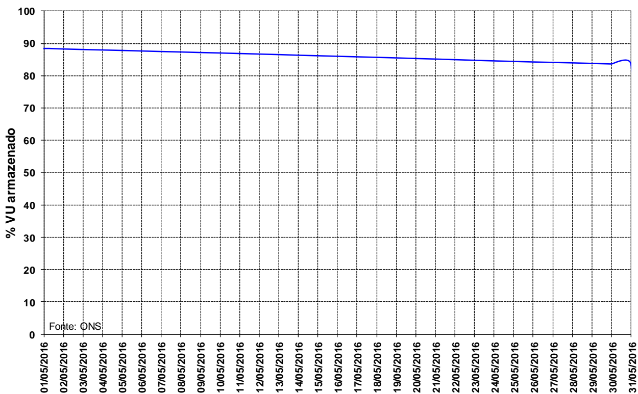
Figura 14 – Volume Útil armazenado na UHE Manso para o mês de maio de 2016.
