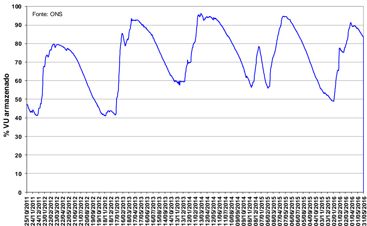
Figura 13 – Volume Útil armazenado na UHE Manso de outubro de 2011 a maio de 2016.
