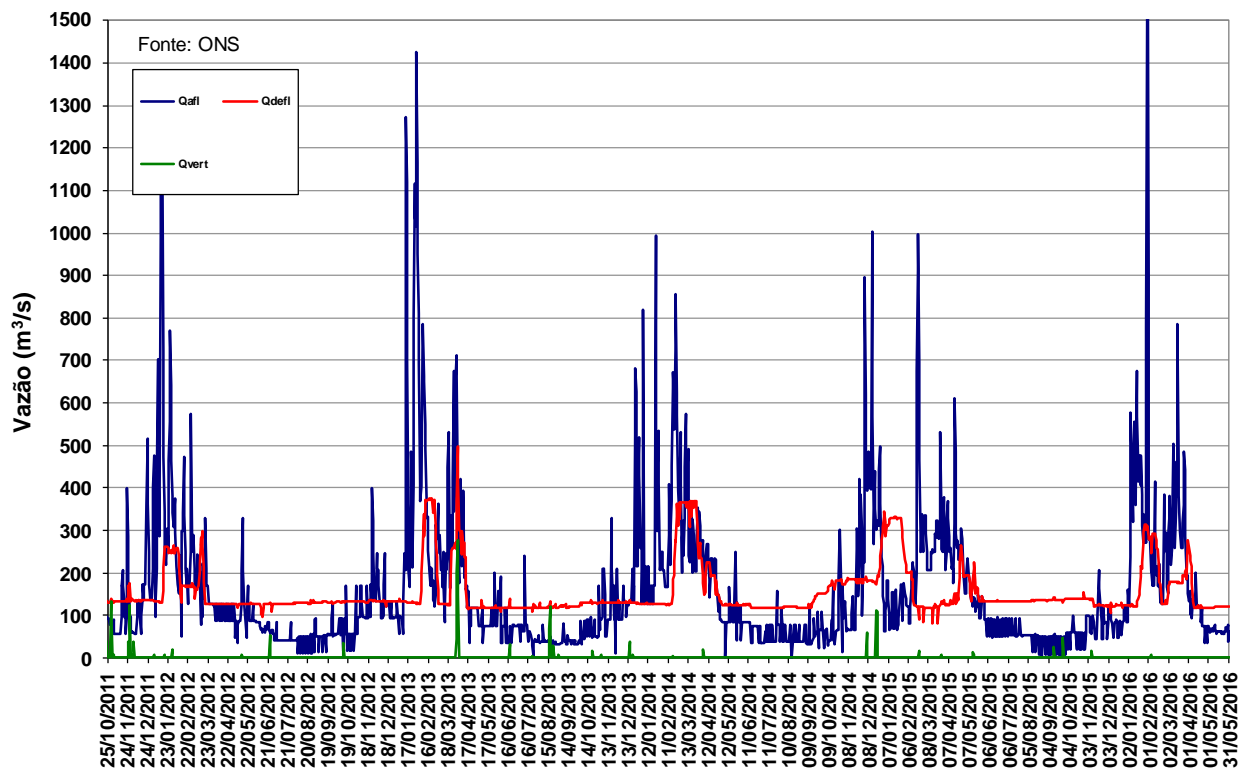
Figura 11 – Vazões na UHE Manso de outubro de 2011 a maio de 2016.
