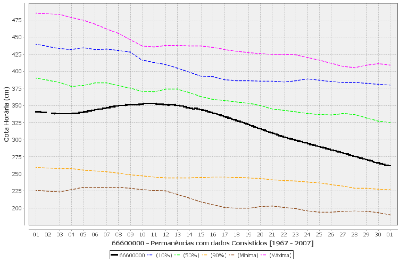
Figura 6 - Gráficos de permanência de cotas, cotas máximas, mínimas e observadas no rio Piquiri, em São Jerônimo.
