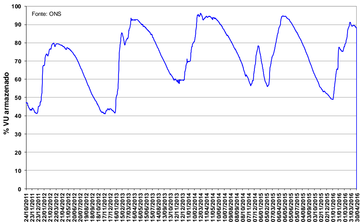
Figura 13 – Volume Útil armazenado na UHE Manso de outubro de 2011 a abril de 2016.
