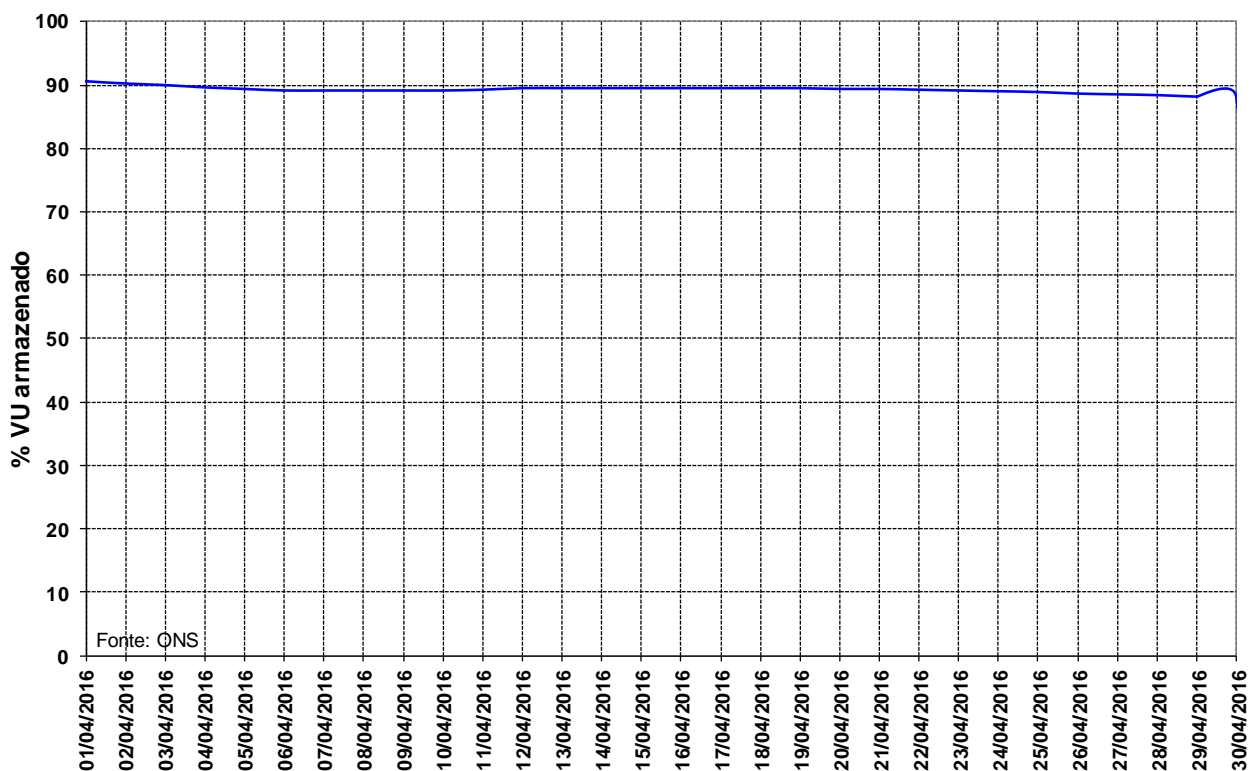
Figura 14 – Volume Útil armazenado na UHE Manso para o mês de abril de 2016.
