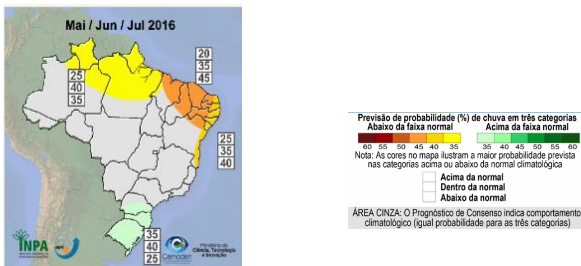
Figura 19 – Previsão climática para o trimestre maio/junho/julho de 2016.
