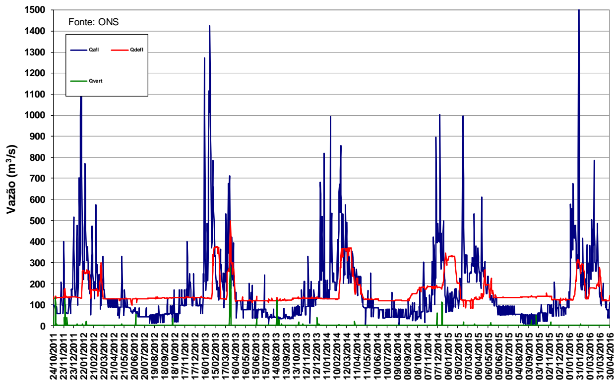
Figura 11 – Vazões na UHE Manso de outubro de 2011 a abril de 2016.
