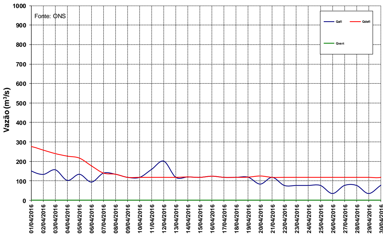
Figura 12 – Vazões na UHE Manso para o mês de abril de 2016.
