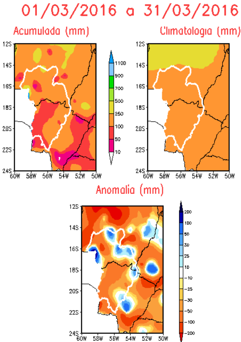
Figura 15 – Precipitação mensal acumulada, média climatológica e anomalia de precipitação na BAP, no período de 01/03/16 a 31/03/16.
