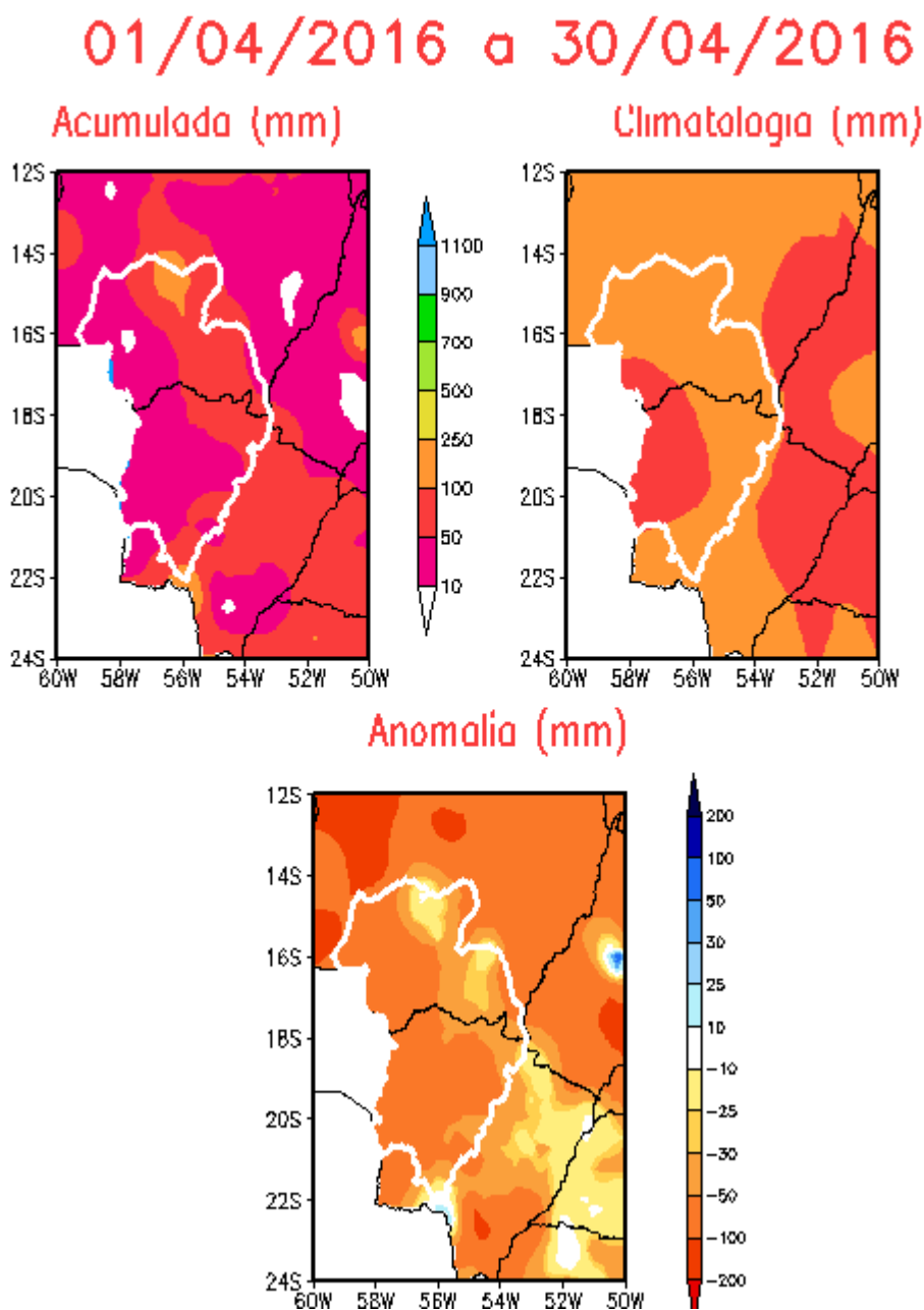
Figura 16 – Precipitação mensal acumulada, média climatológica e anomalia de precipitação na BAP, no período de 01/04/16 a 30/04/16.
