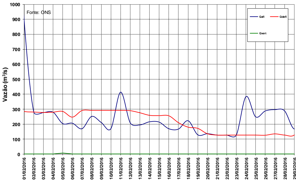
Fonte: ONS Figura 12 – Vazões na UHE Manso para o mês de fevereiro de 2016.
