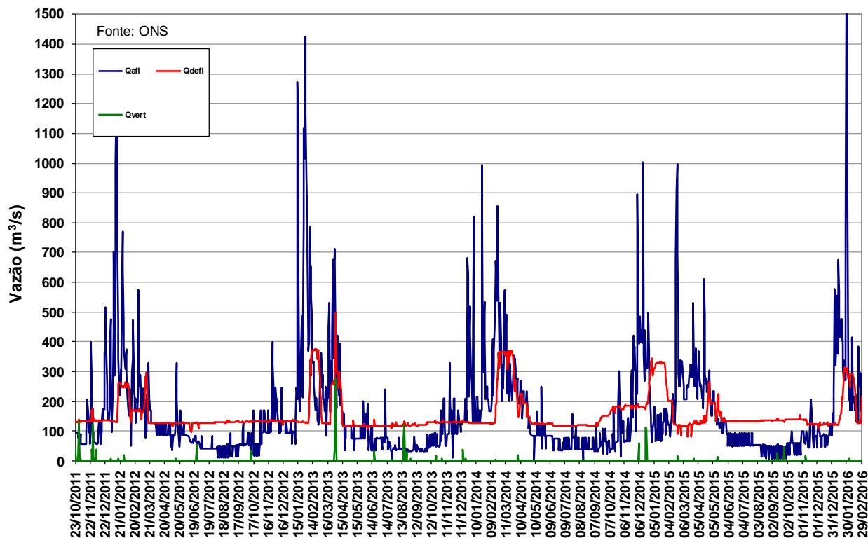
Fonte: ONS Figura 11 – Vazões na UHE Manso de outubro de 2011 a fevereiro de 2016.
