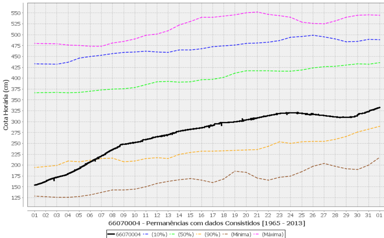
Figura 7 - Gráficos de permanência de cotas, cotas máximas, mínimas e observadas no rio Paraguai, em Cáceres.
