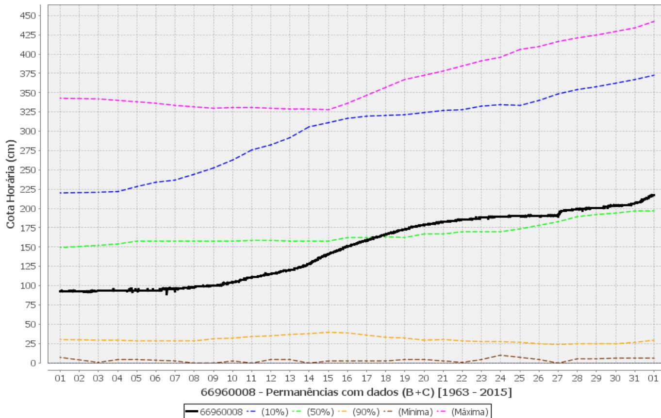
Figura 8 - Gráficos de permanência de cotas, cotas máximas, mínimas e observadas no rio Paraguai, em Porto Esperança.
