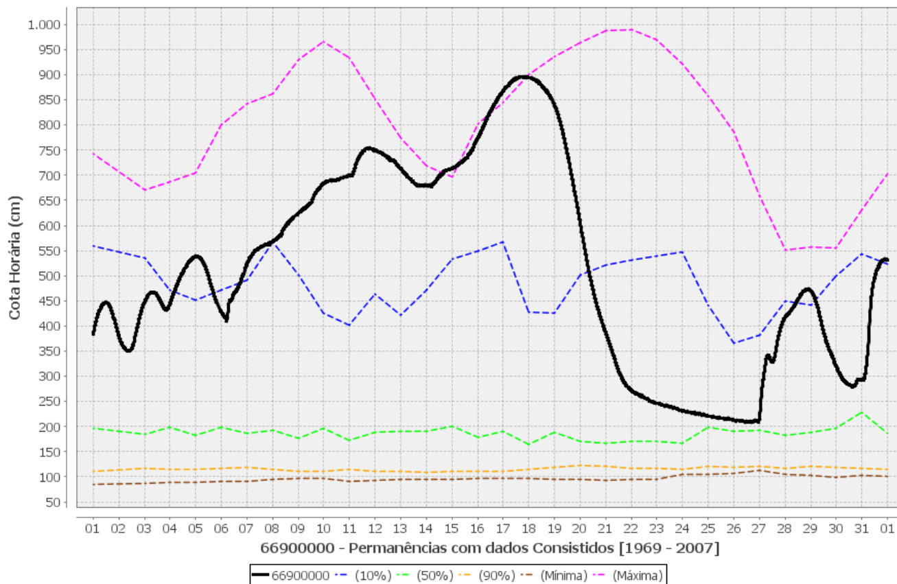
Figura 10 - Gráficos de permanência de cotas, cotas máximas, mínimas e observadas no rio Miranda, na Ponte MT-738.
