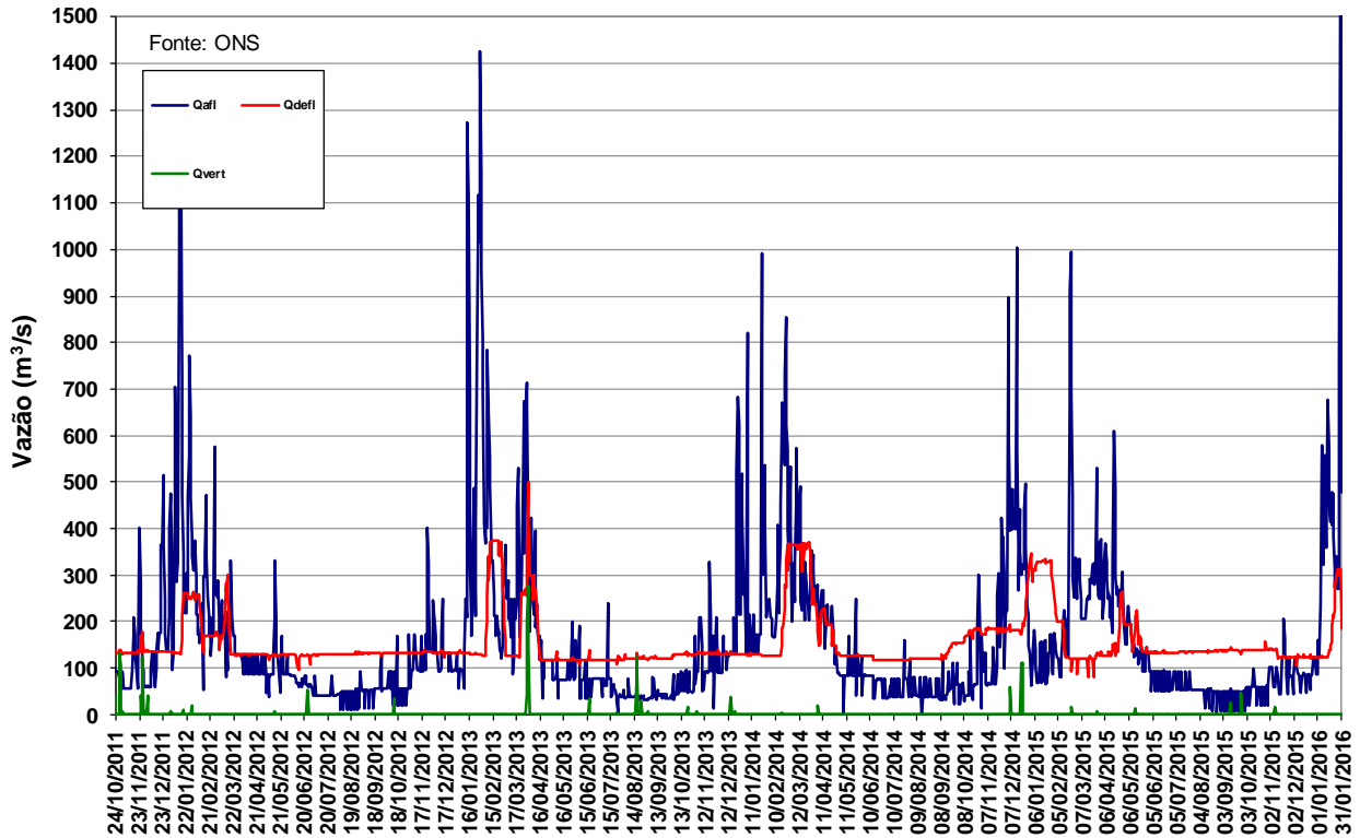
Figura 11 – Vazões na UHE Manso de outubro de 2011 a janeiro de 2016.
