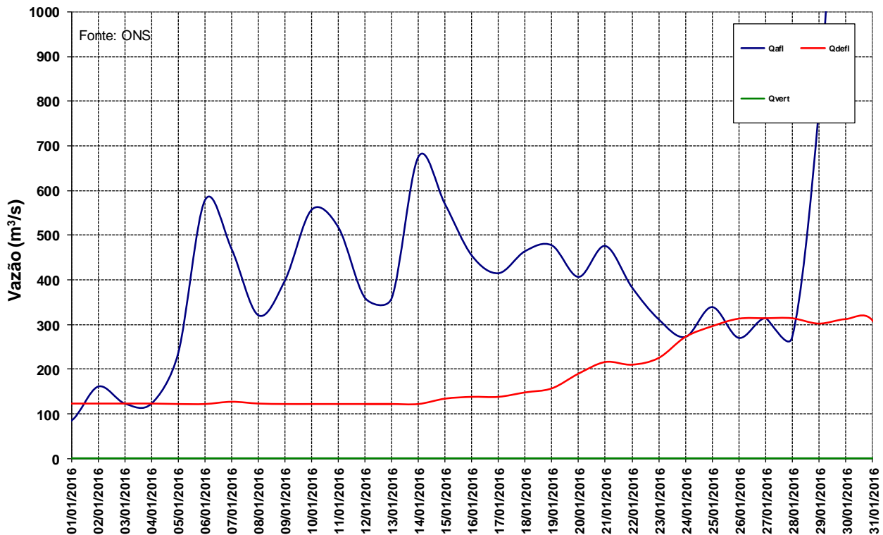
Figura 12 – Vazões na UHE Manso para o mês de janeiro de 2016.
