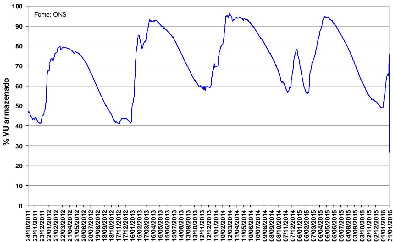
Figura 13 – Volume Útil armazenado na UHE Manso de outubro de 2011 a janeiro de 2016.
