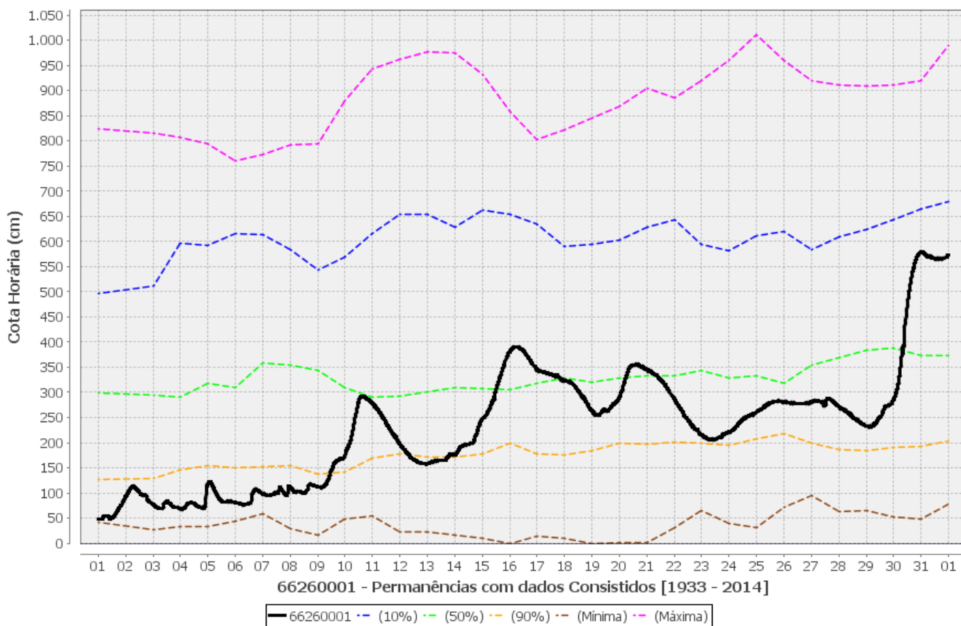
Figura 5 – Gráficos de permanência de cotas, cotas máximas, mínimas e observadas no rio Cuiabá, em Cuiabá.
