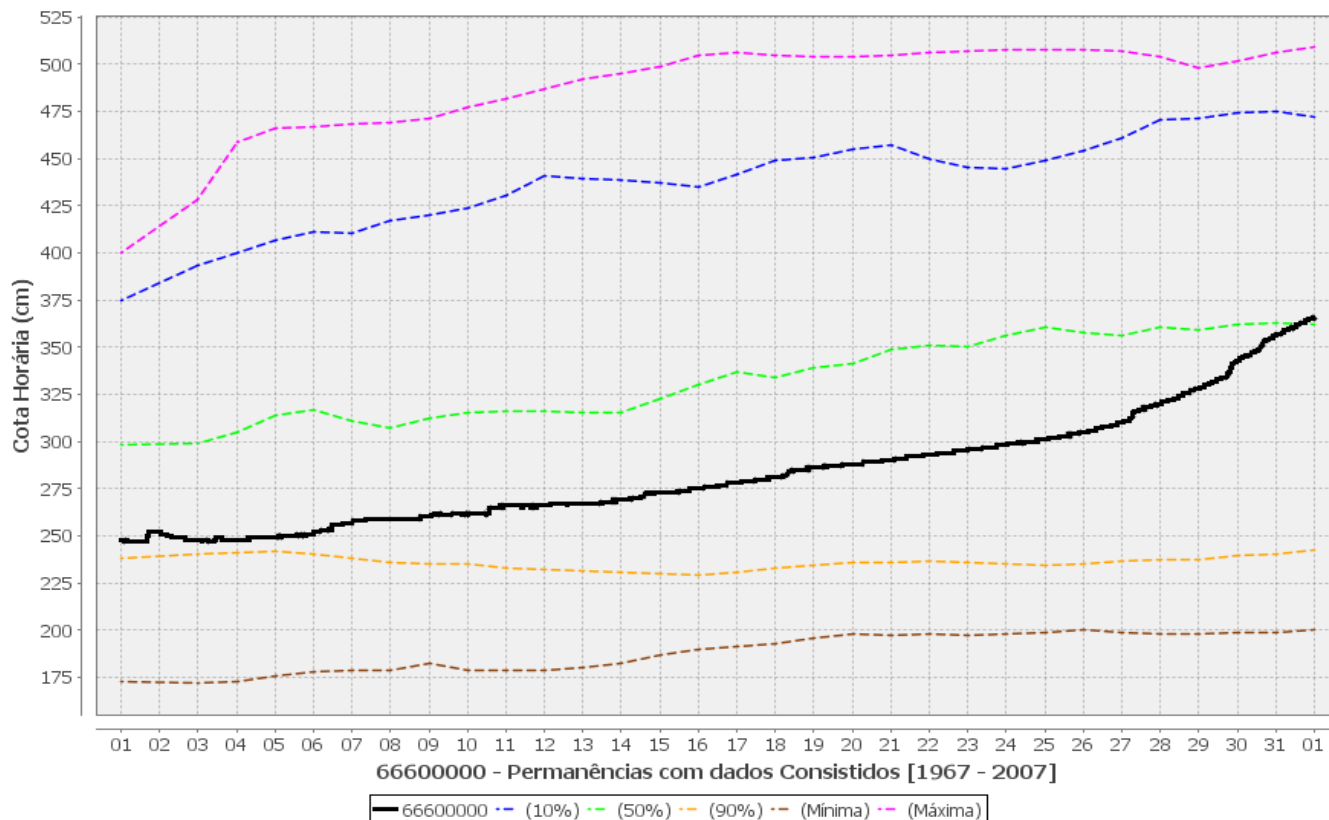
Figura 6 - Gráficos de permanência de cotas, cotas máximas, mínimas e observadas no rio Piquiri, em São Jerônimo.
