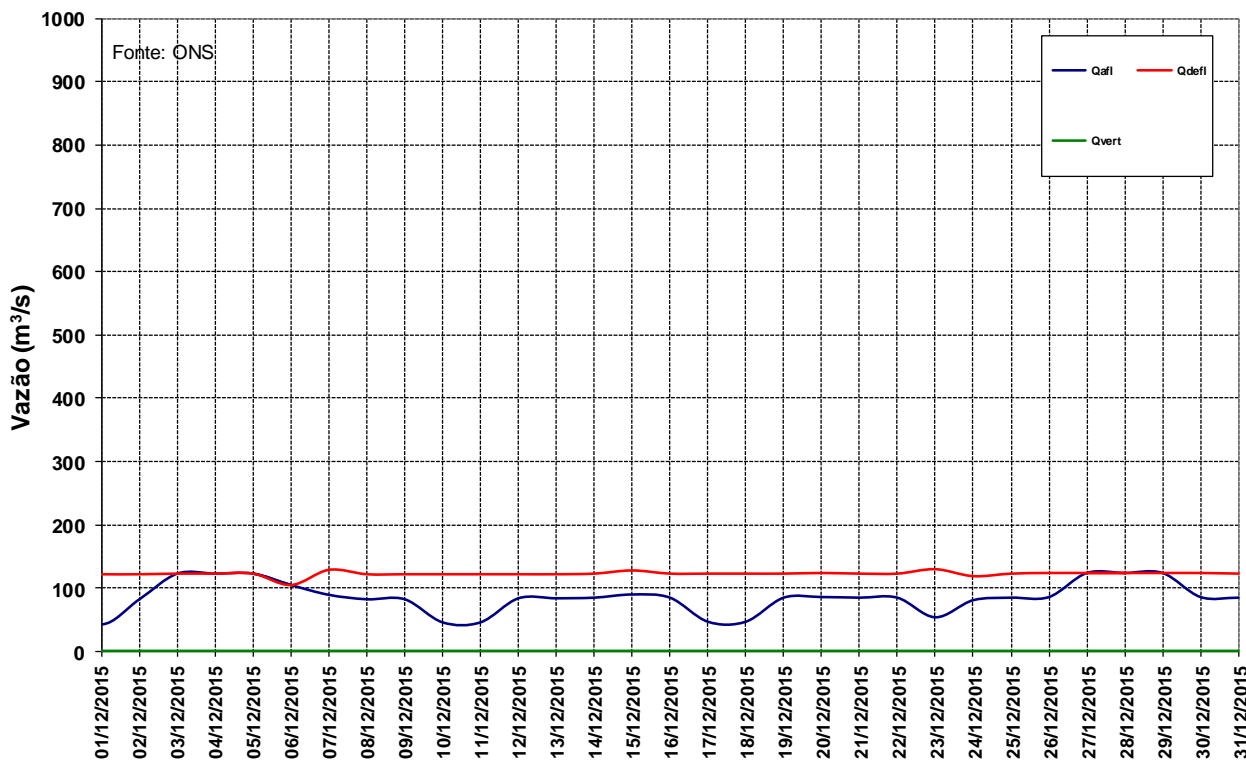
Figura 12 – Vazões na UHE Manso para o mês de dezembro de 2015.
