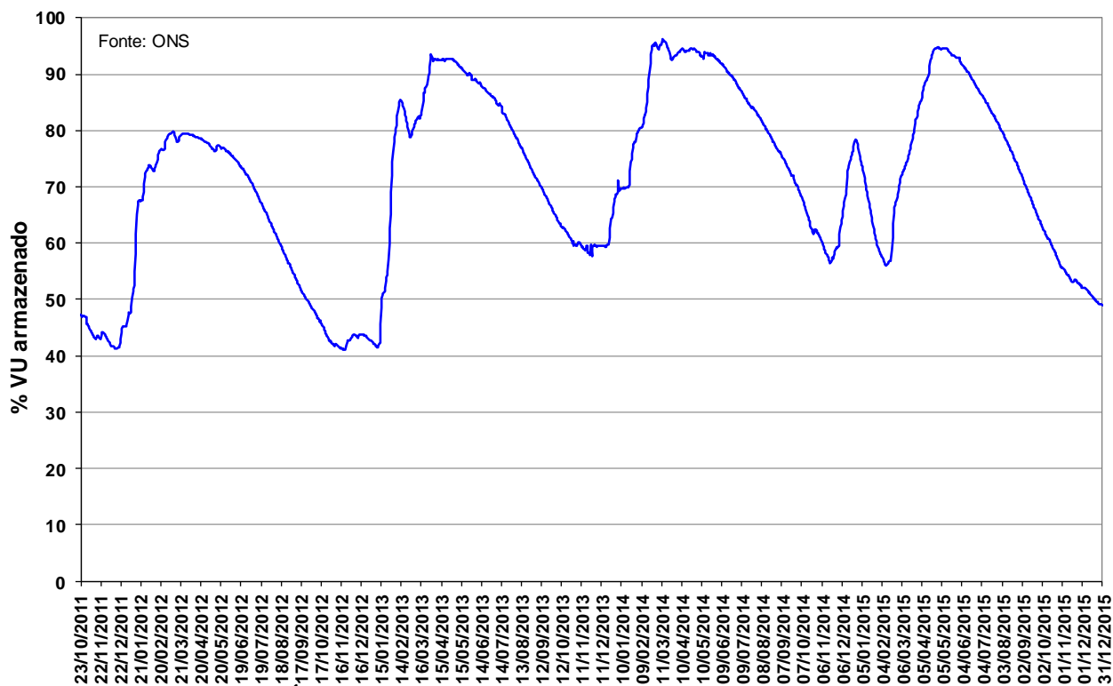
Figura 13 – Volume Útil armazenado na UHE Manso de outubro de 2011 a dezembro de 2015.
