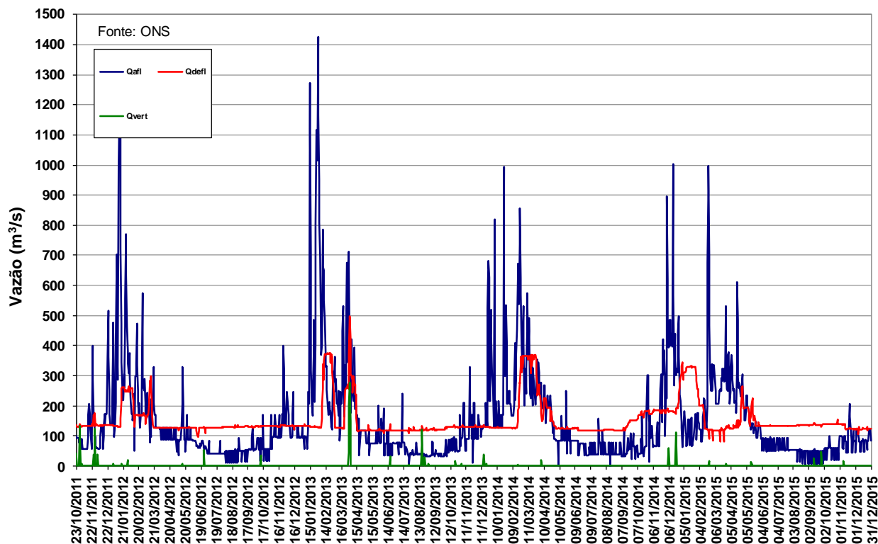
Figura 11 – Vazões na UHE Manso de outubro de 2011 a dezembro de 2015.
