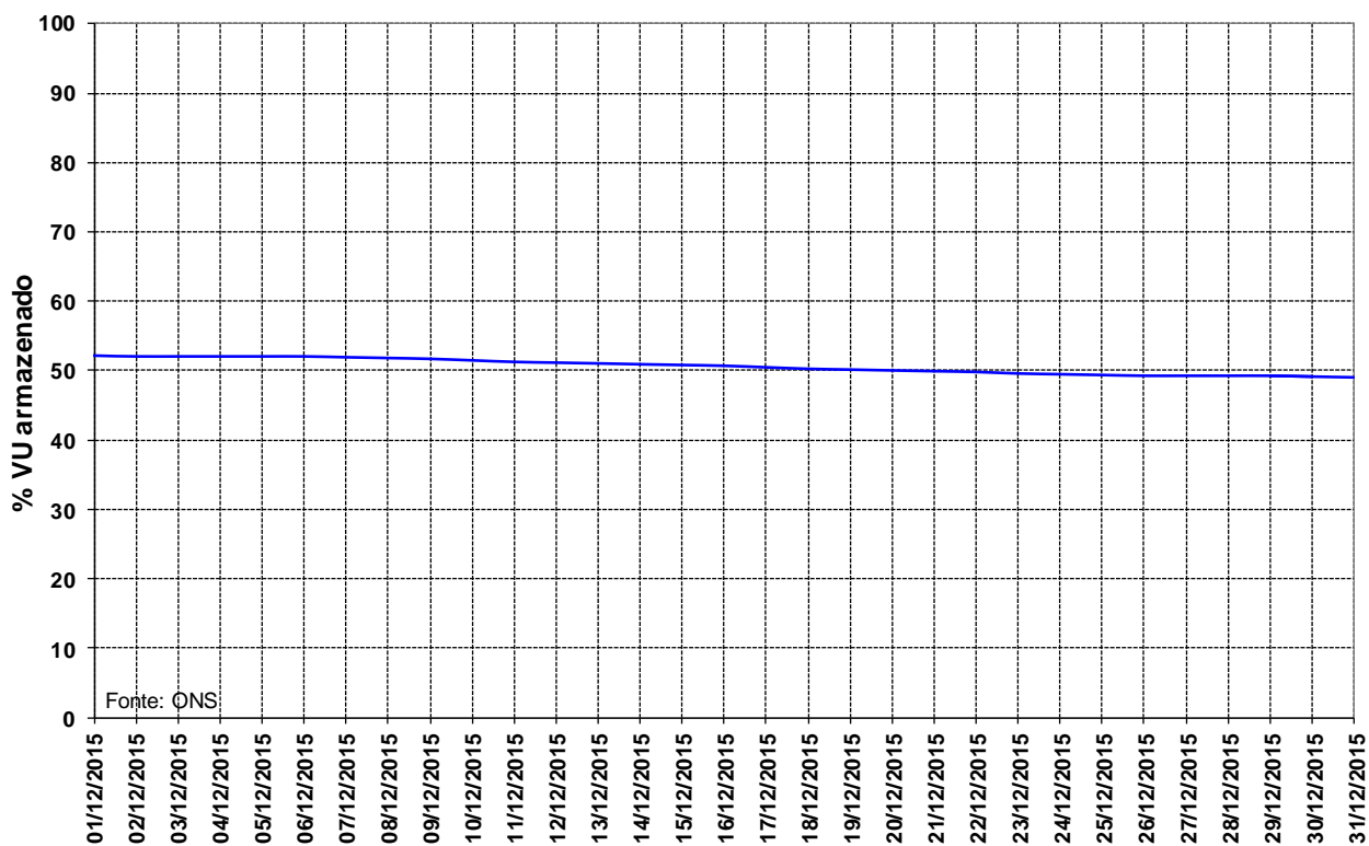
Figura 14 – Volume Útil armazenado na UHE Manso para o mês de dezembro de 2015.
