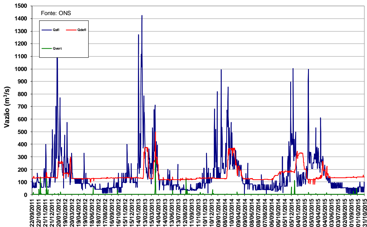
Figura 11 – Vazões na UHE Manso de setembro de 2011 a outubro de 2015.
