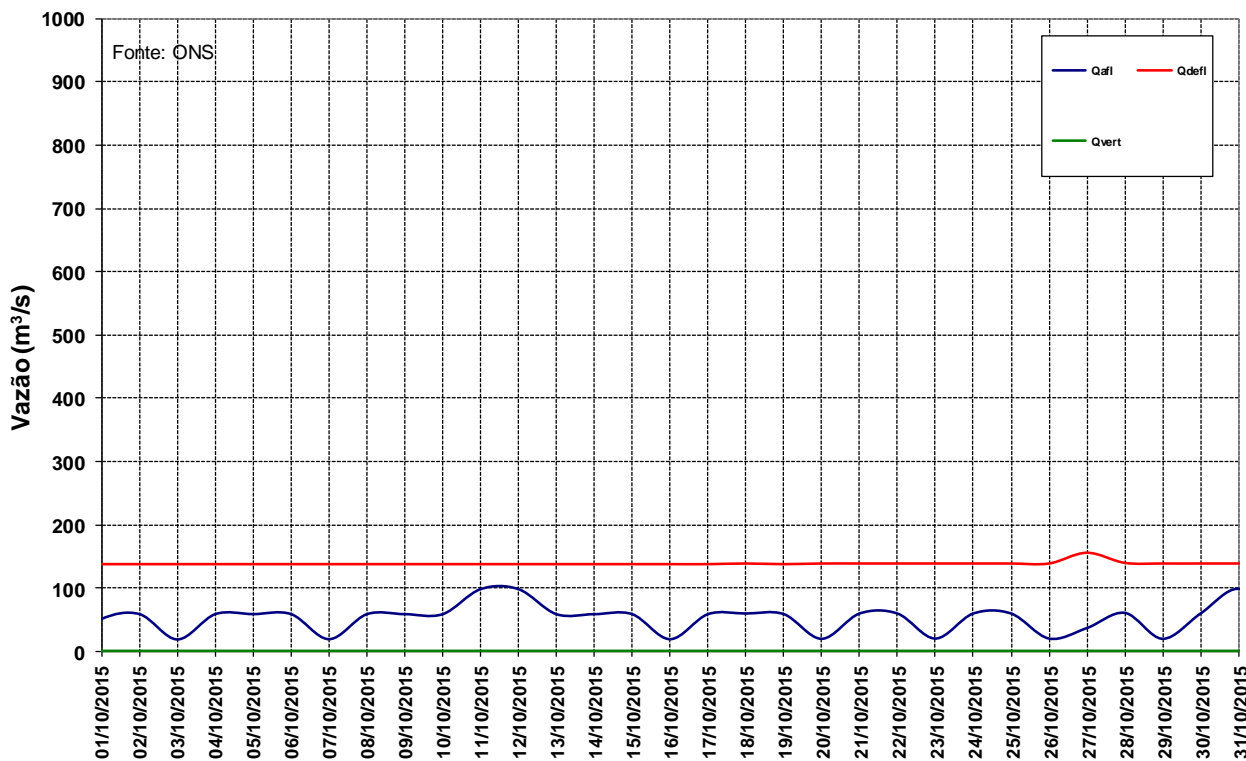
Figura 12 – Vazões na UHE Manso para o mês de outubro de 2015.
