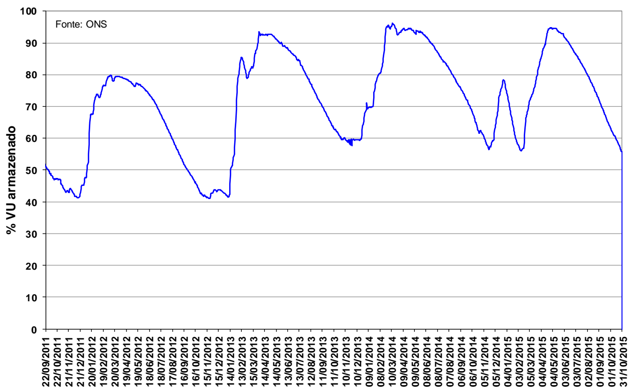
Figura 13 – Volume Útil armazenado na UHE Manso de setembro de 2011 a outubro de 2015.
