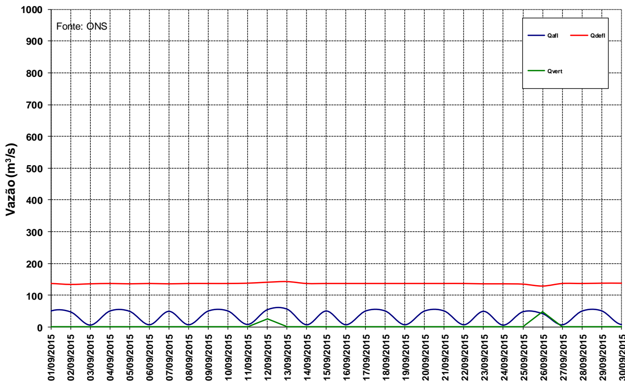
Fonte: ONS Figura 12 – Vazões na UHE Manso para o mês de setembro de 2015.
