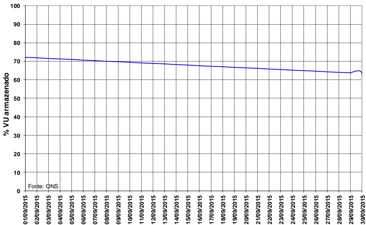
Figura 14 – Volume Útil armazenado na UHE Manso para o mês de setembro de 2015.
