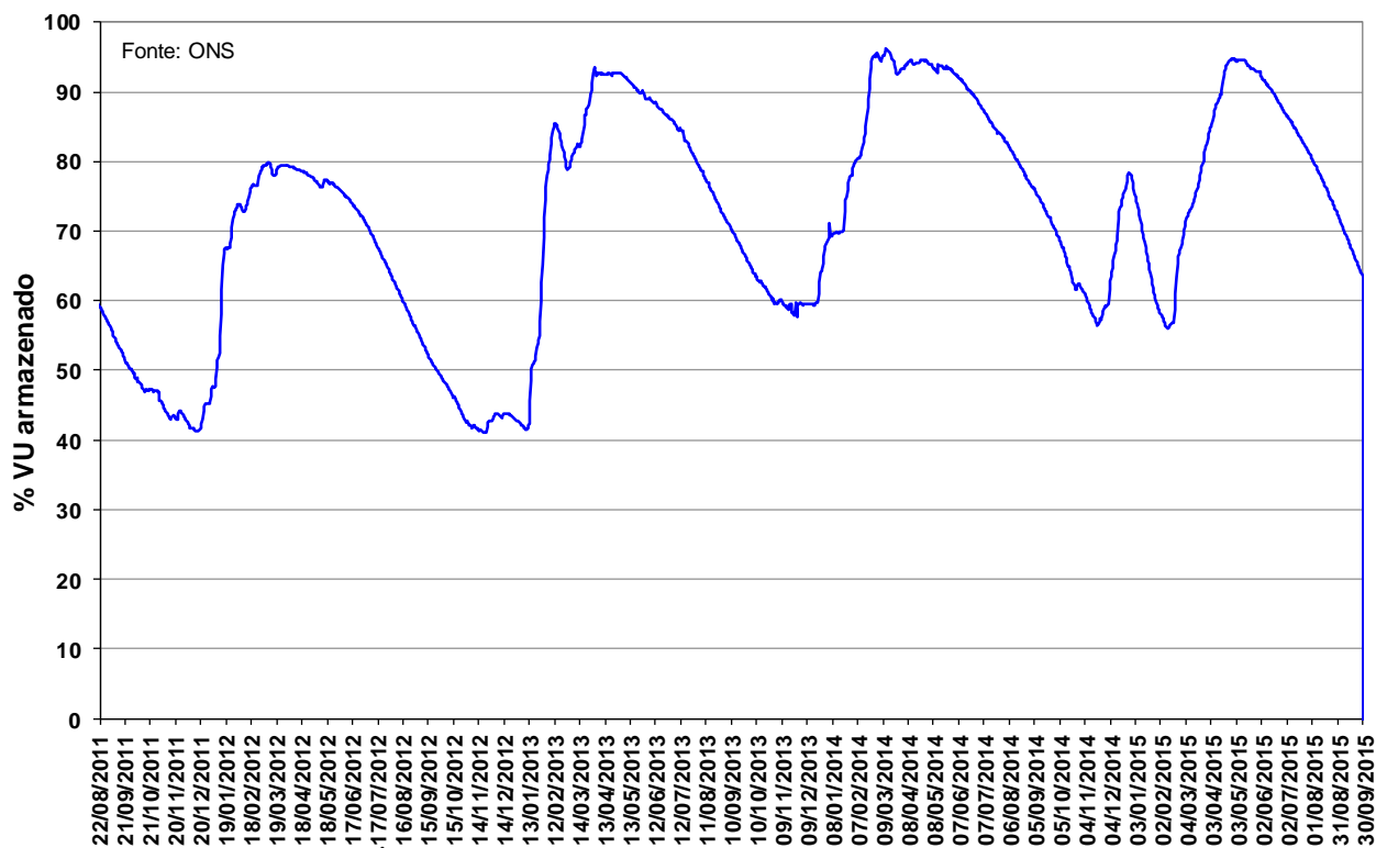
Figura 13 – Volume Útil armazenado na UHE Manso de agosto de 2011 a setembro de 2015.
