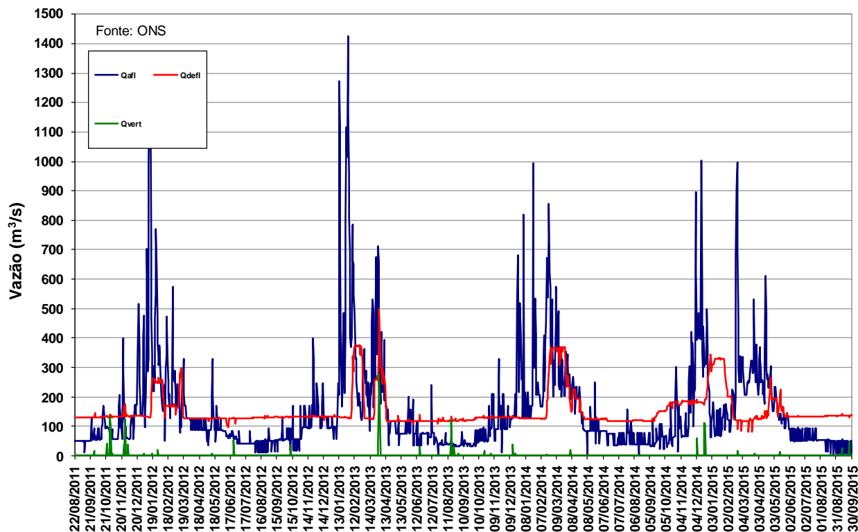
Fonte: ONS Figura 11 – Vazões na UHE Manso de agosto de 2011 a setembro de 2015.
