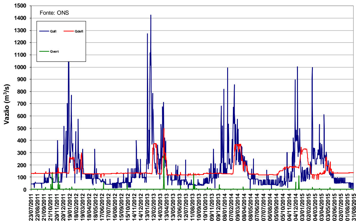
Figura 11 – Vazões na UHE Manso de julho de 2011 a agosto de 2015.
