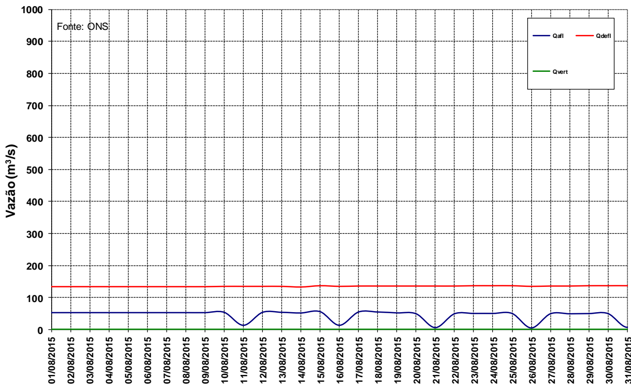
Figura 12 – Vazões na UHE Manso para o mês de agosto de 2015.
