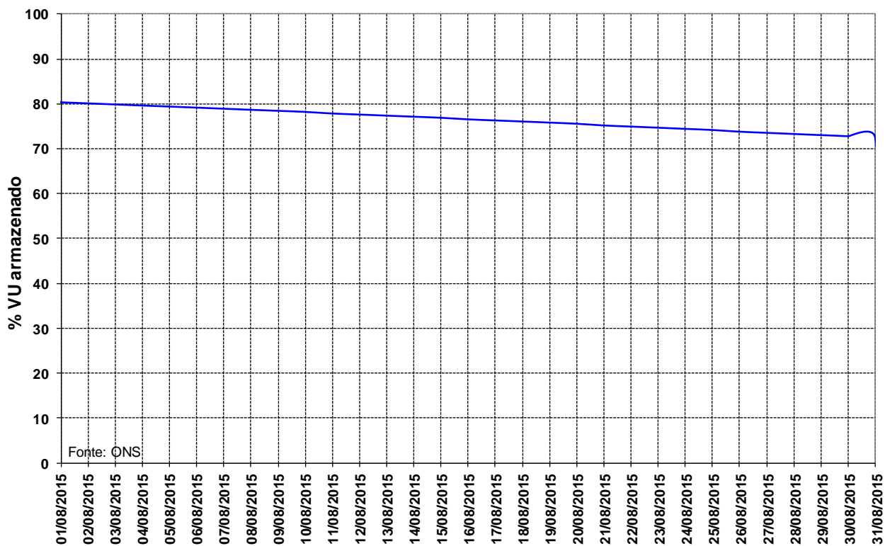
Figura 14 – Volume Útil armazenado na UHE Manso para o mês de agosto de 2015.
