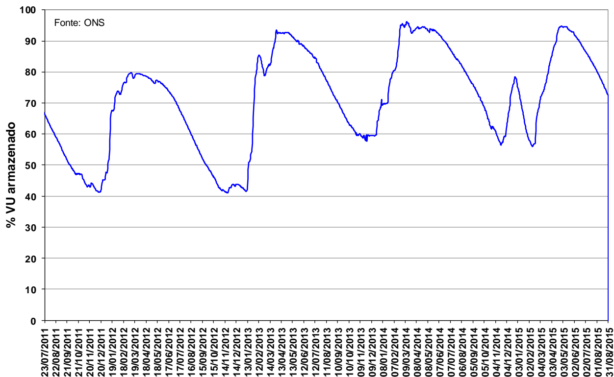
Figura 13 – Volume Útil armazenado na UHE Manso de julho de 2011 a agosto de 2015.
