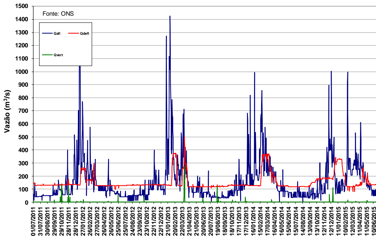
Figura 11 – Vazões na UHE Manso de julho de 2011 a junho de 2015.
