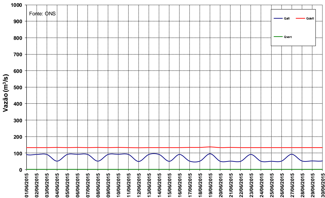
Figura 12 – Vazões na UHE Manso para o mês de junho de 2015.
