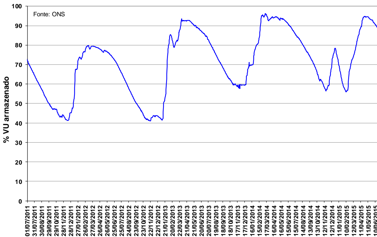
Figura 13 – Volume Útil armazenado na UHE Manso de julho de 2011 a junho de 2015.
