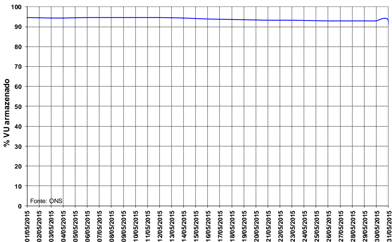
Figura 14 – Volume Útil armazenado na UHE Manso para o mês de maio de 2015.
