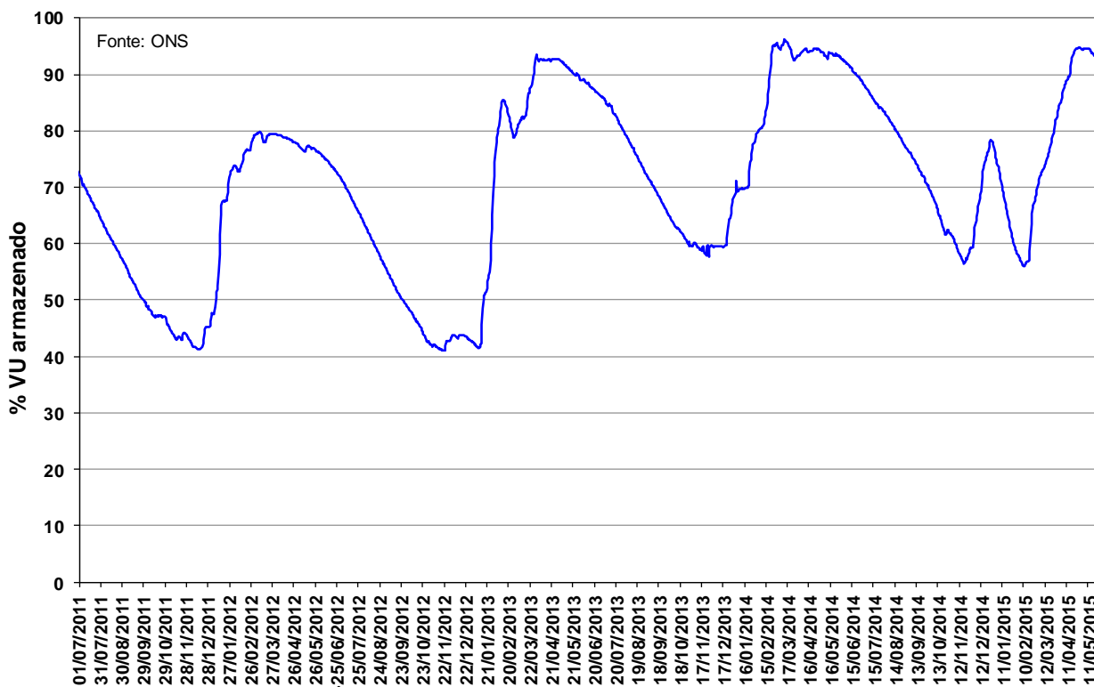
Figura 13 – Volume Útil armazenado na UHE Manso de julho de 2011 a maio de 2015.
