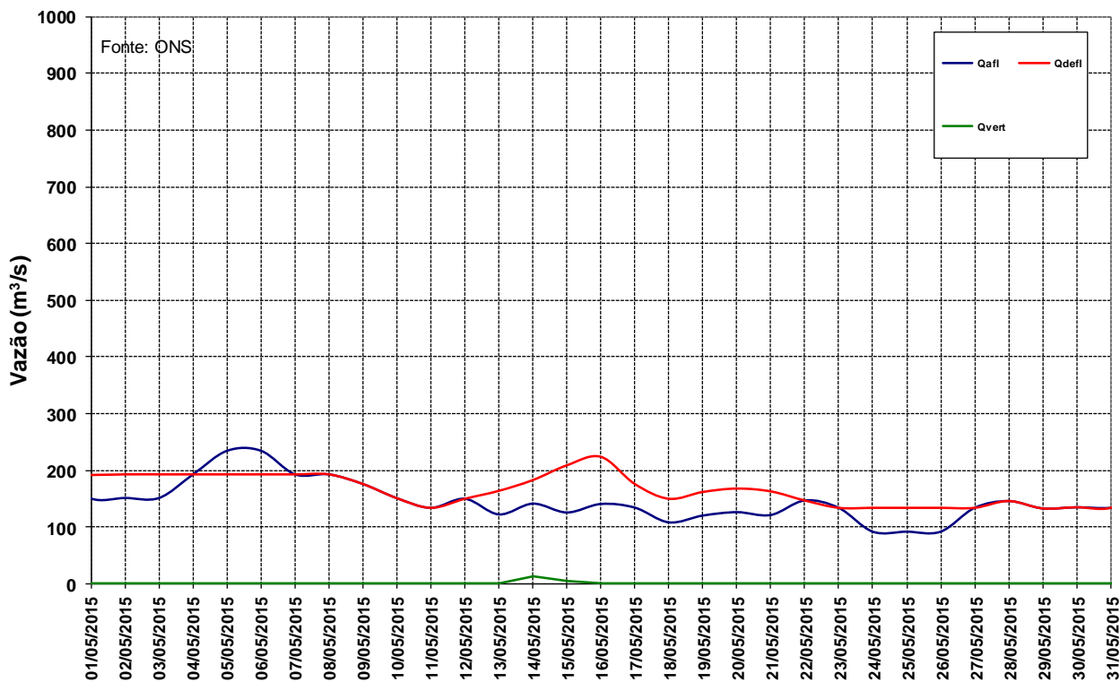
Figura 12 – Vazões na UHE Manso para o mês de maio de 2015.
