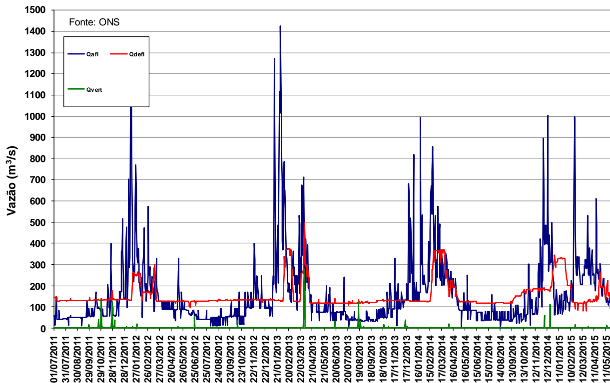
Figura 11 – Vazões na UHE Manso de julho de 2011 a maio de 2015.
